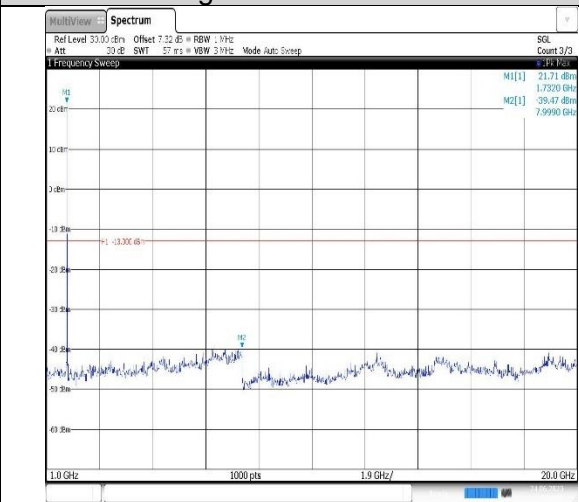
Band4-1.4MHz-QPSK-20393-1RB#0-Range2:1000~20000MHz
