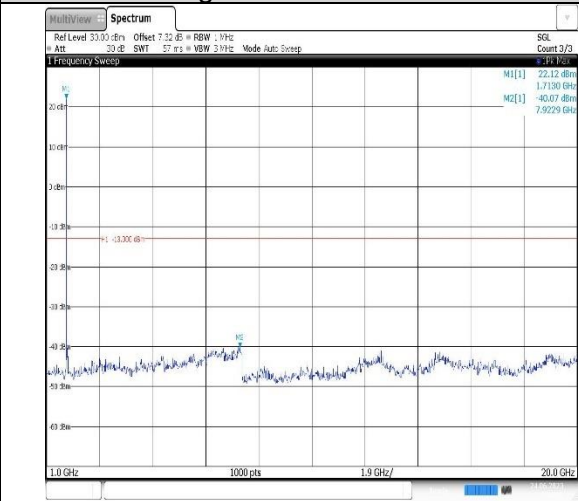
Band4-1.4MHz-QPSK-19957-1RB#0-Range2:1000~20000MHz
