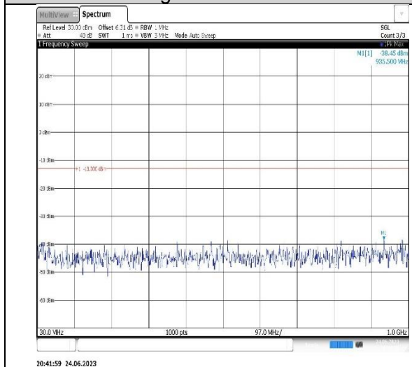
Band4-5MHz-QPSK-20375-1RB#0- Range1:30~1000MHz
