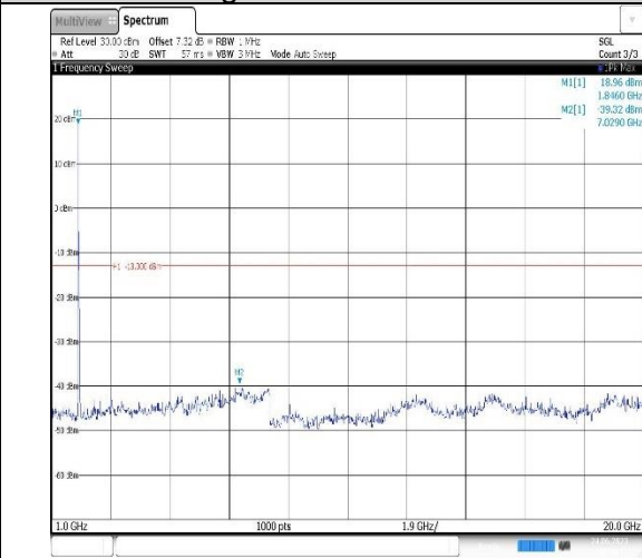
Band2-20MHz-16QAM-18700-1RB#0-Range2:1000~20000MHz
