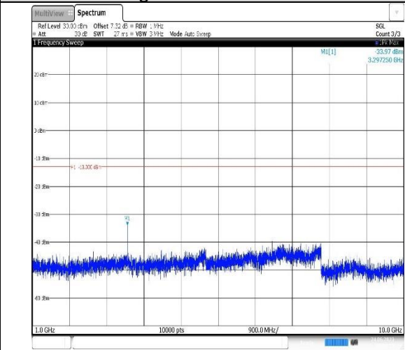
Band5-3MHz-QPSK-20415-1RB#0- Range2:1000~10000MHz
