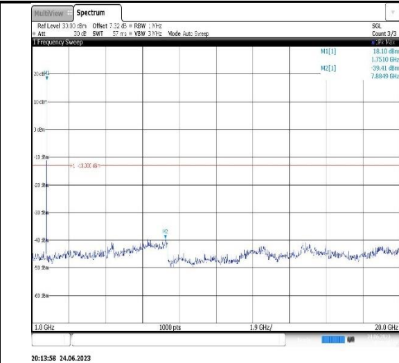
Band4-5MHz-QPSK-19975-1RB#0- Range2:1000~20000MHz
