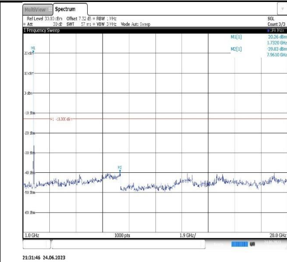
Band4-20MHz-QPSK-20050-1RB#0-Range2:1000~20000MHz
