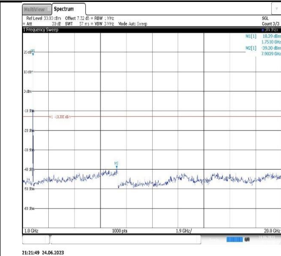
Band4-15MHz-QPSK-20025-1RB#0- Range2:1000~20000MHz
