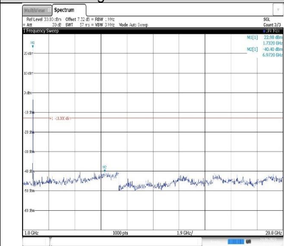
Band4-10MHz-QPSK-20350-1RB#0-Range2:1000~20000MHz
