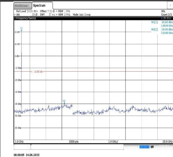
Band2-20MHz-16QAM-18700-1RB#0-Range2:1000~20000MHz
