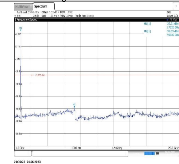
Band4-20MHz-QPSK-20300-1RB#0-Range2:1000~20000MHz
