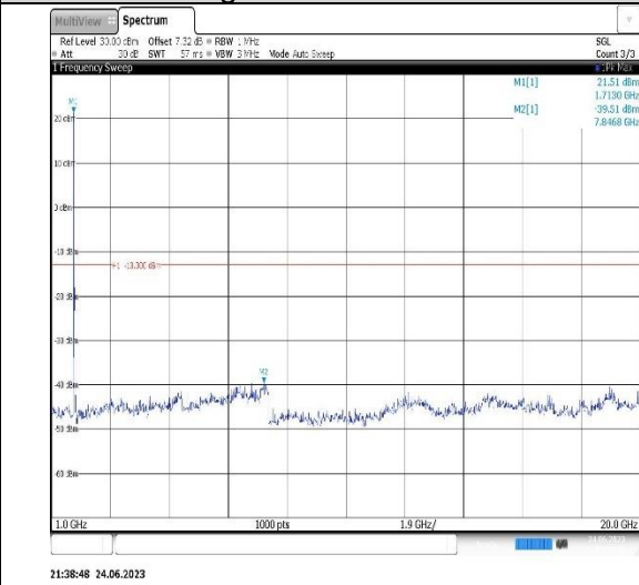
Band4-20MHz-QPSK-20175-1RB#0-Range2:1000~20000MHz
