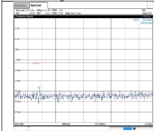
Band4-1.4MHz-QPSK-20393-1RB#0-Range1:30~1000MHz
