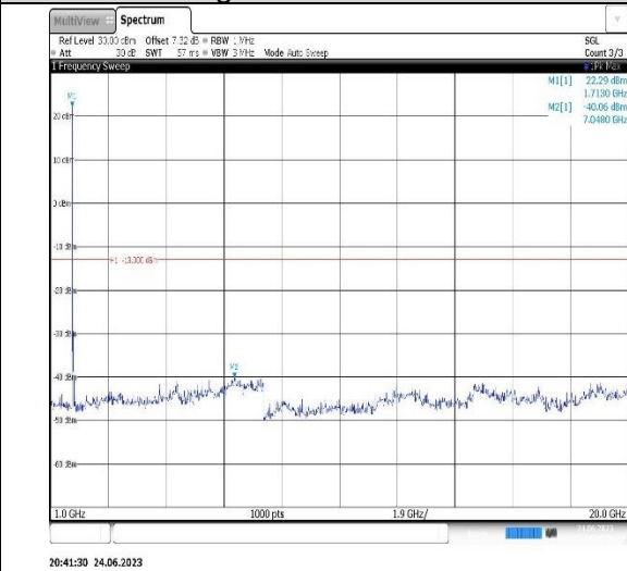
Band4-5MHz-QPSK-20175-1RB#0- Range2:1000~20000MHz
