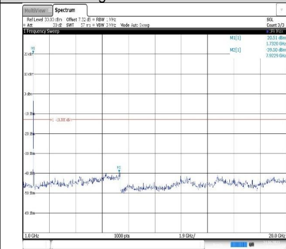
Band4-15MHz-QPSK-20325-1RB#0- Range2:1000~20000MHz
