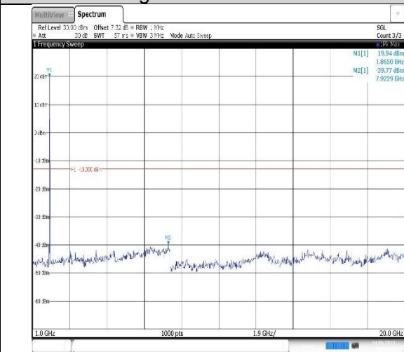
Band2-20MHz-16QAM-19100-1RB#0-Range2:1000~20000MHz
