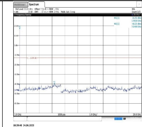
18:39:48 24.06.2023 Band2-20MHz-QPSK-18700-1RB#0-Range2:1000~20000MHz
