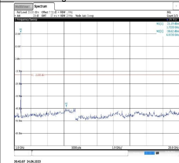
Band4-5MHz-QPSK-20375-1RB#0- Range2:1000~20000MHz
