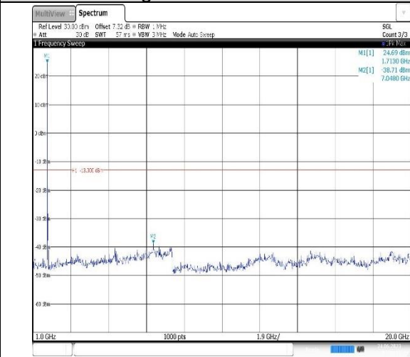
Band4-15MHz-QPSK-20025-1RB#0- Range2:1000~20000MHz
