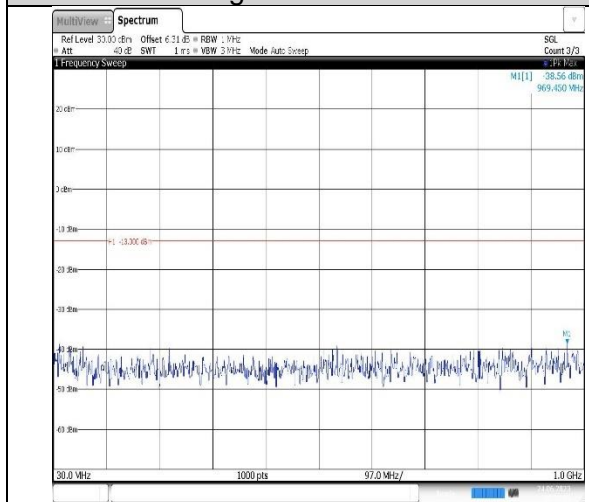
Band2-5MHz-QPSK-19175-1RB#0- Range1:30~1000MHz
