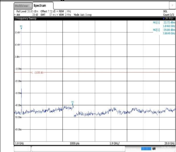
Band2-5MHz-QPSK-18625-1RB#0- Range2:1000~20000MHz
