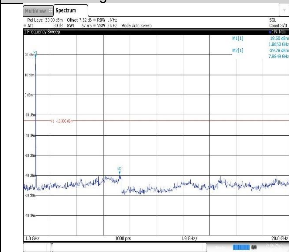
Band2-15MHz-QPSK-19125-1RB#0-Range2:1000~20000MHz
