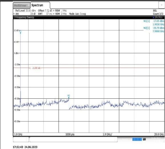
Band2-5MHz-QPSK-18625-1RB#0- Range2:1000~20000MHz
