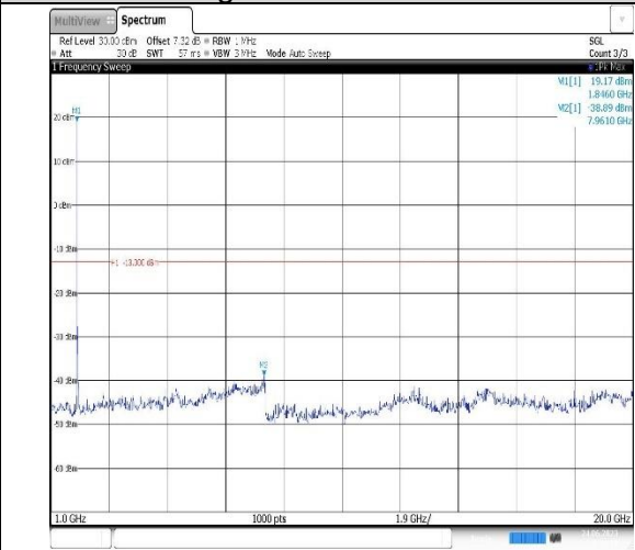
Band2-3MHz-QPSK-18615-1RB#0-Range2:1000~20000MHz
