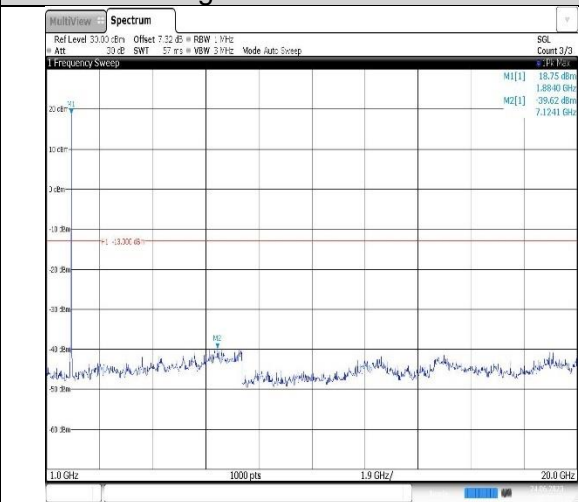
Band2-5MHz-QPSK-19175-1RB#0- Range2:1000~20000MHz
