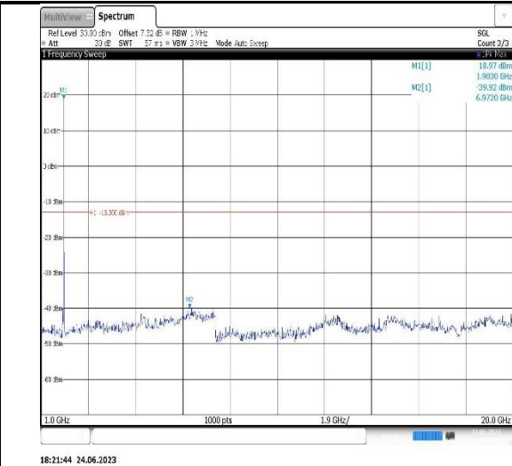
Band2-10MHz-QPSK-18650-1RB#0-Range2:1000~20000MHz
