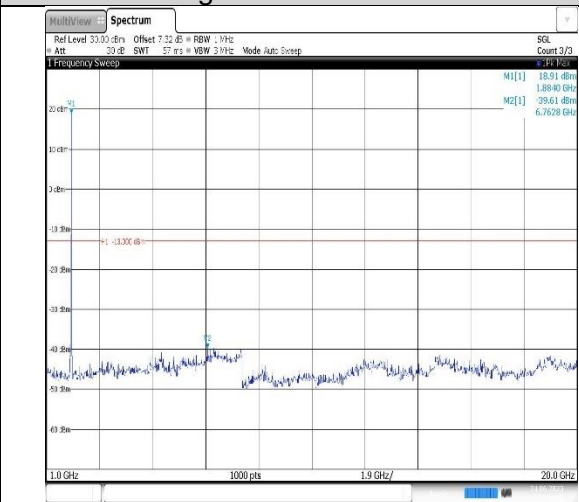
Band2-3MHz-QPSK-19185-1RB#0-Range2:1000~20000MHz
