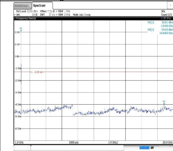
Band2-10MHz-QPSK-18650-1RB#0-Range2:1000~20000MHz
