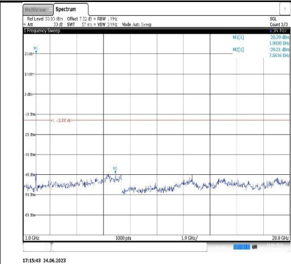
Band2-3MHz-QPSK-18615-1RB#0-Range2:1000~20000MHz
