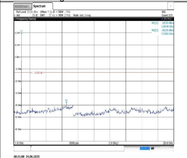
Band2-5MHz-16QAM-19175-1RB#0-Range2:1000~20000MHz
