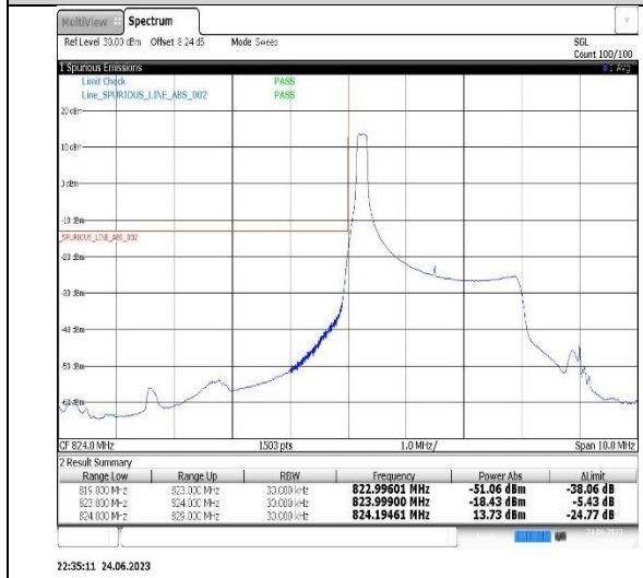
Band5-3MHz-QPSK-20635-1RB#14
