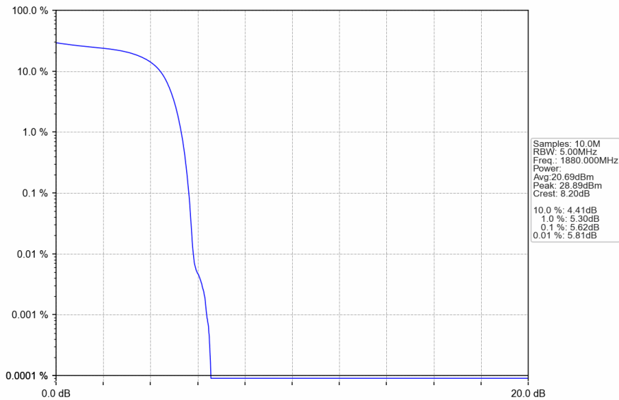
Band2_HSUPA_MCH_1880MHz_Subtest 1_NTNV
