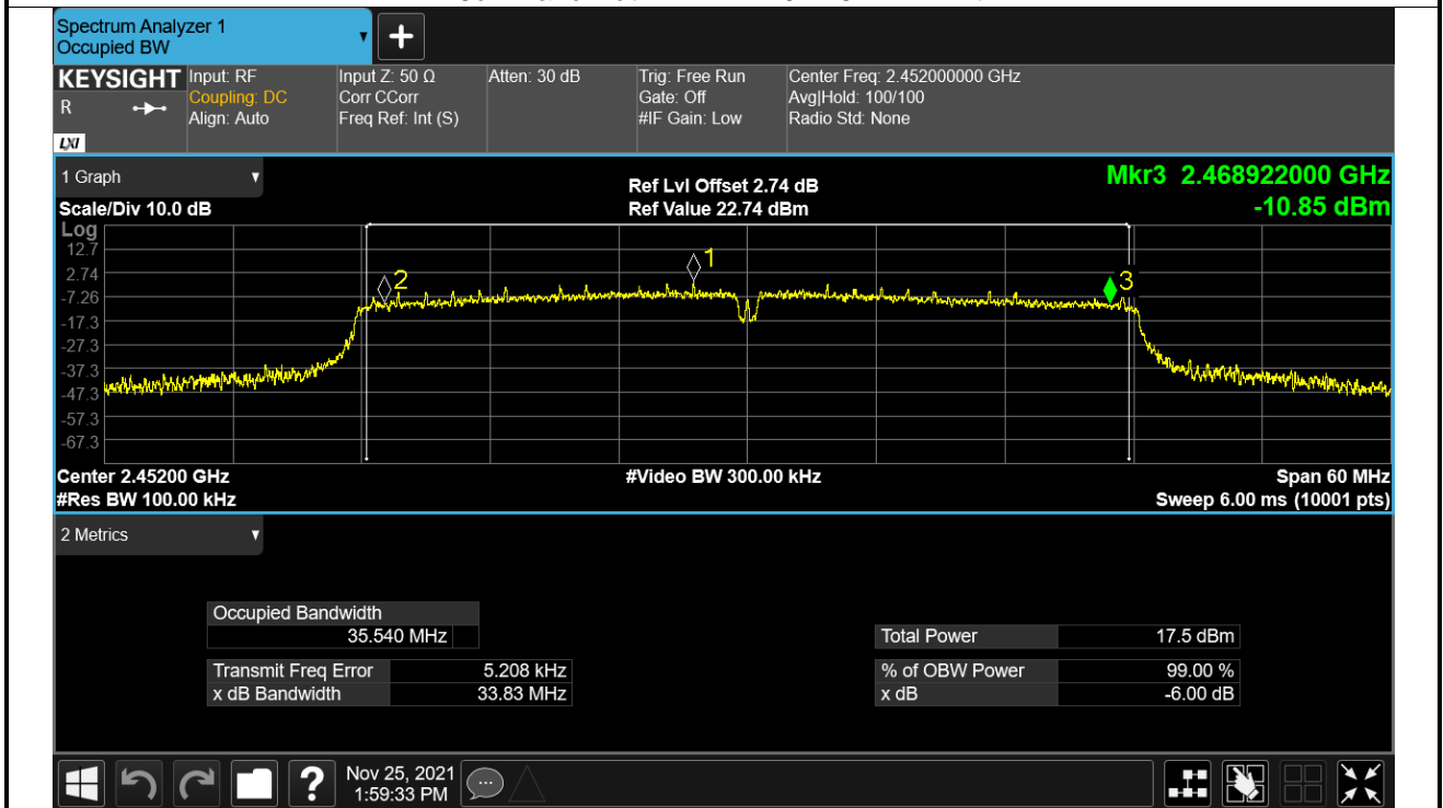
-6dB Bandwidth NVNT n40 2452MHz Ant1
