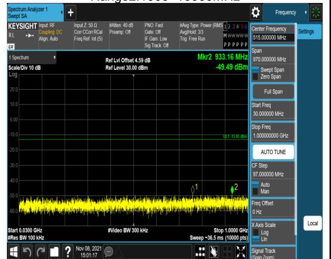
Band13-5MHz-QPSK-23230-1RB#0- Range1:30~1000MHz
