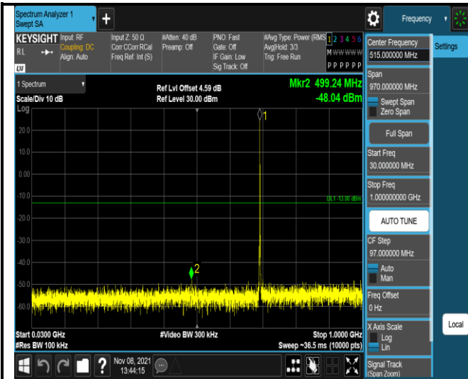
Band12-1.4MHz-QPSK-23017-1RB#0- Range1:30~1000MHz
