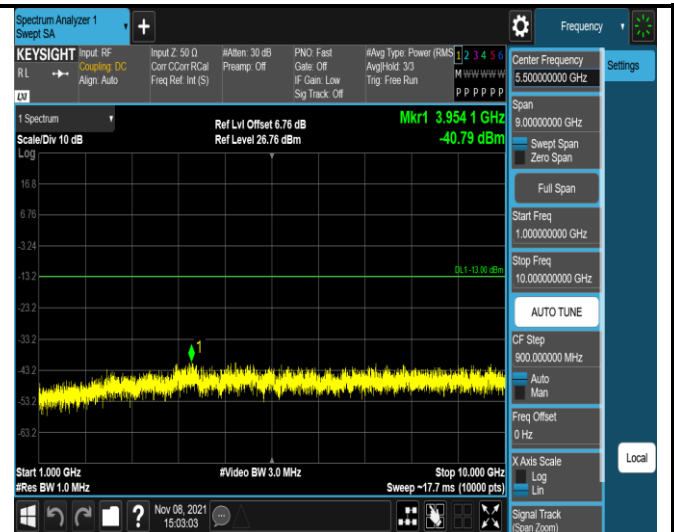
Band13-5MHz-QPSK-23255-1RB#0- Range2:1000~10000MHz
