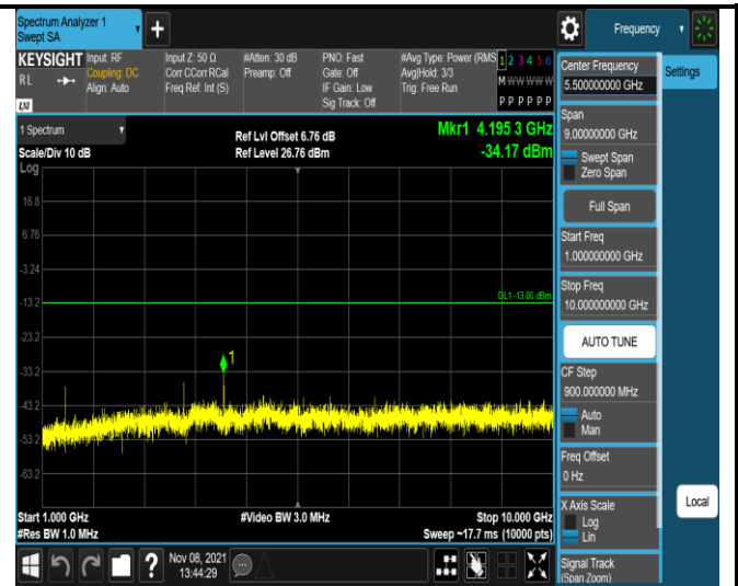
Band12-1.4MHz-QPSK-23017-1RB#0- Range2:1000~10000MHz
