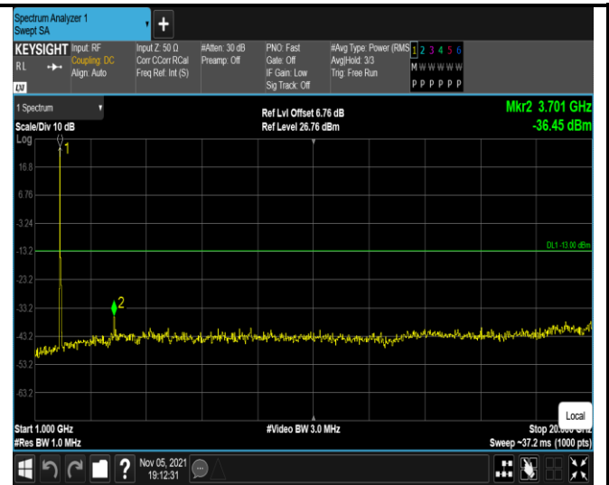
Band2-20MHz-QPSK-18700-1RB#0-Range2:1000~20000MHz
