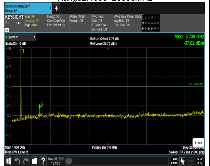
Band2-20MHz-QPSK-18900-1RB#0-Range2:1000~20000MHz
