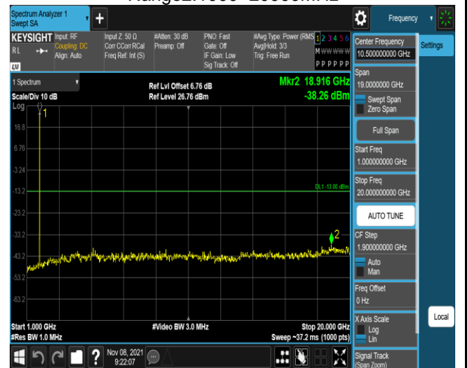
Band4-1.4MHz-QPSK-20393-1RB#0- Range2:1000~20000MHz
