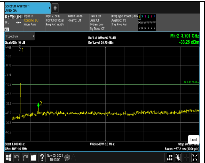
Band2-20MHz-16QAM-18700-1RB#0- Range2:1000~20000MHz
