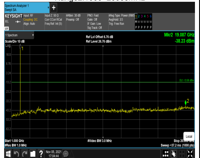
Band2-1.4MHz-QPSK-19193-1RB#0- Range2:1000~20000MHz
