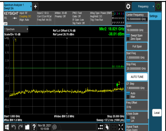
Band4-20MHz-QPSK-20050-1RB#0- Range2:1000~20000MHz
