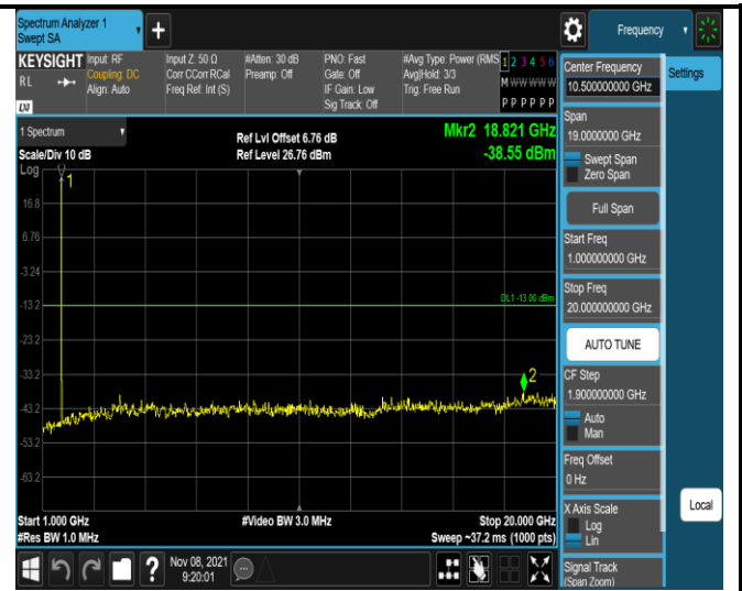
Band4-1.4MHz-QPSK-19957-1RB#0- Range2:1000~20000MHz
