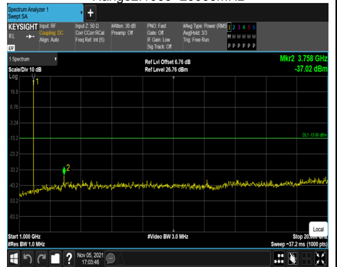
Band2-1.4MHz-QPSK-18900-1RB#0- Range2:1000~20000MHz
