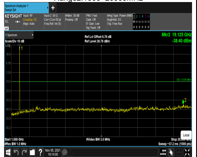
Band2-20MHz-16QAM-18900-1RB#0- Range2:1000~20000MHz
