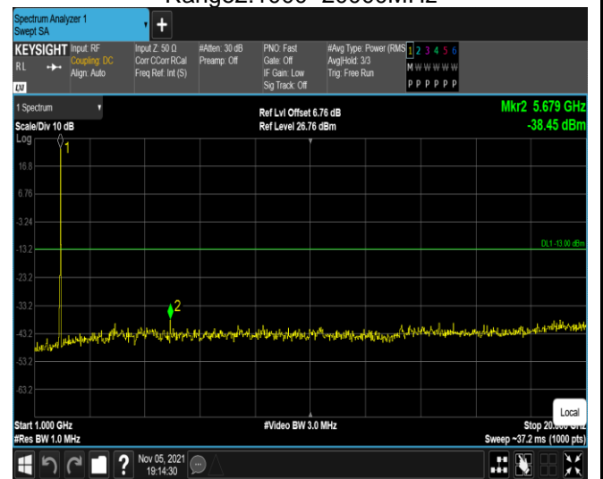
Band2-20MHz-QPSK-19100-1RB#0-Range2:1000~20000MHz
