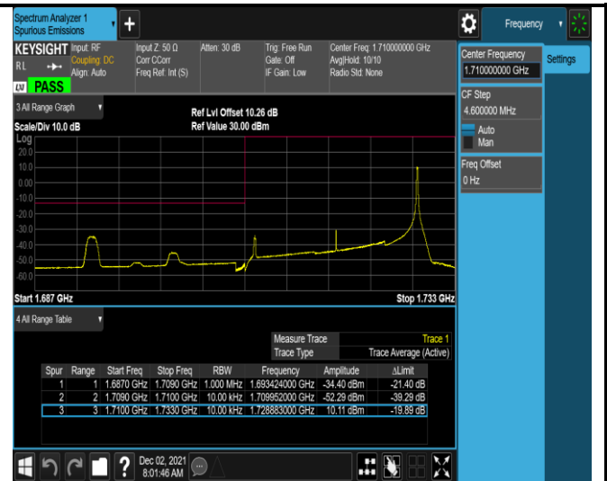
Band4-20MHz-QPSK-20050-1RB#99
