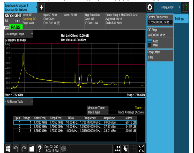
Band4-20MHz-QPSK-20050-100RB#99
