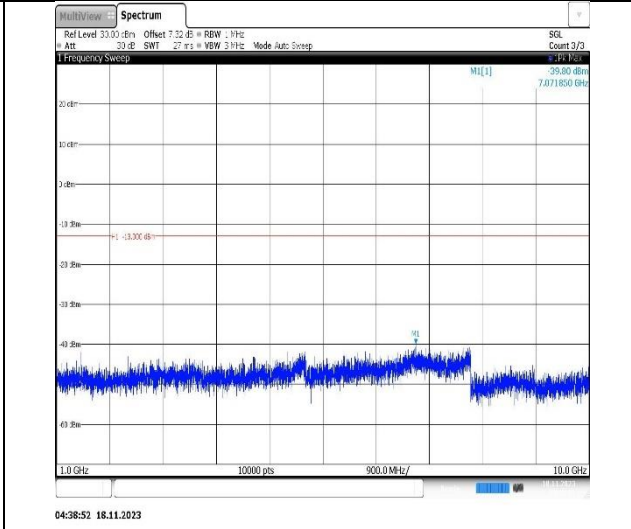
Band12-5MHz-QPSK-23155-1RB#0-Range2:1000~10000MHz
