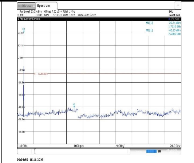
Band4-15MHz-QPSK-20025-1RB#0-Range2:1000~20000MHz
