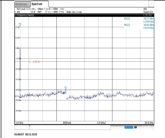
Band4-20MHz-QPSK-20300-1RB#0-Range2:1000~20000MHz
