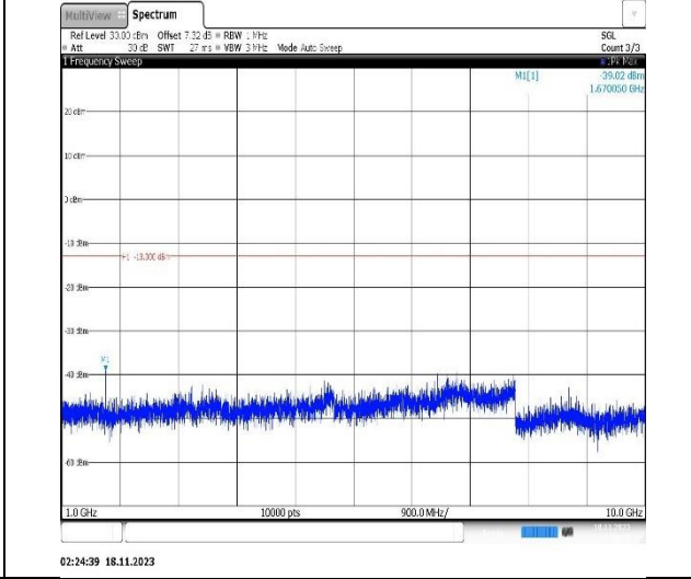
Band5-3MHz-QPSK-20635-1RB#0-Range2:1000~10000MHz
