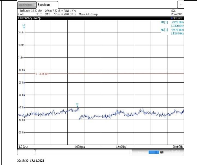
Band4-3MHz-QPSK-20385-1RB#0-Range2:1000~20000MHz
