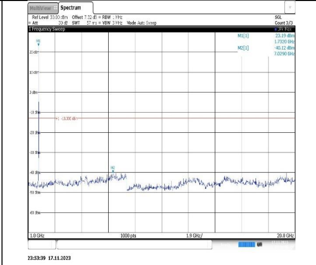
Band4-10MHz-QPSK-20350-1RB#0- Range2:1000~20000MHz
