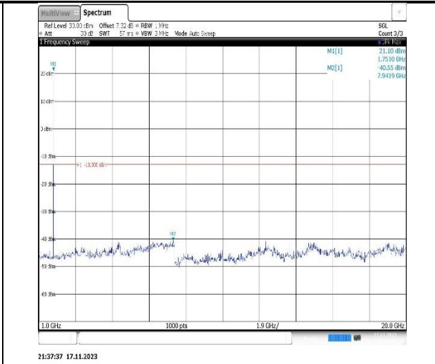
Band4-3MHz-QPSK-19965-1RB#0-Range2:1000~20000MHz
