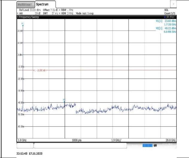
Band4-3MHz-QPSK-20175-1RB#0-Range2:1000~20000MHz
