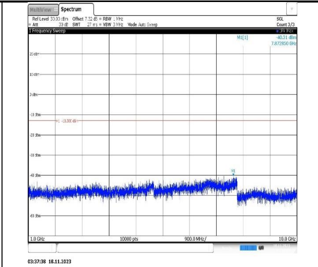
Band12-1.4MHz-QPSK-23017-1RB#0-Range2:1000~10000MHz
