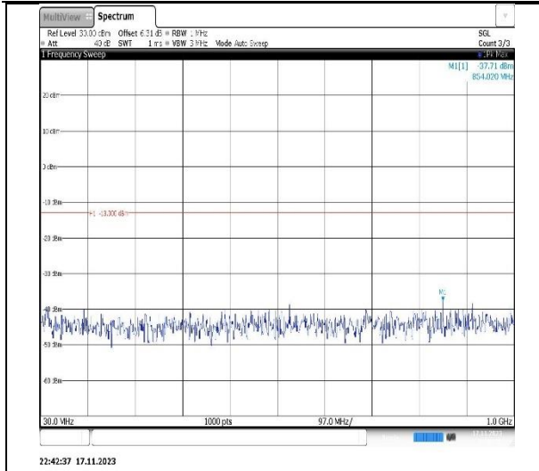
Band4-10MHz-QPSK-20000-1RB#0- Range1:30~1000MHz
