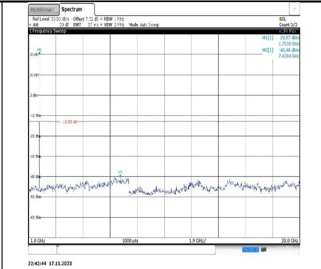
Band4-10MHz-QPSK-20000-1RB#0- Range2:1000~20000MHz
