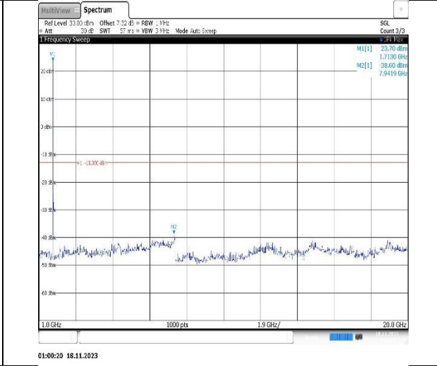
Band4-20MHz-QPSK-20175-1RB#0-Range2:1000~20000MHz
