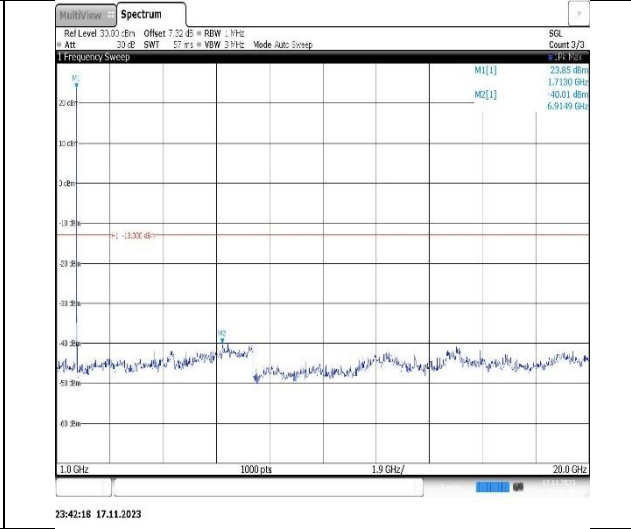
Band4-10MHz-QPSK-20175-1RB#0- Range2:1000~20000MHz
