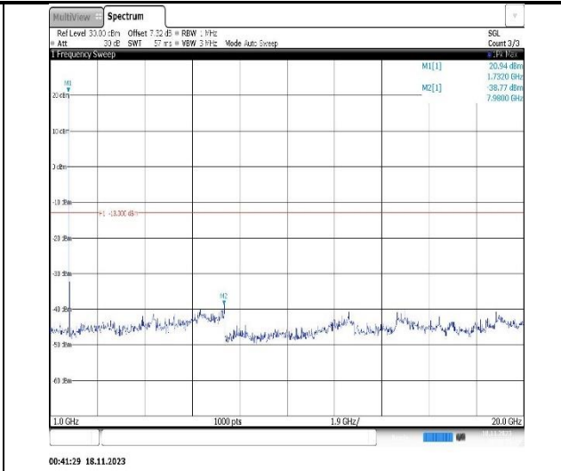
Band4-20MHz-QPSK-20050-1RB#0-Range2:1000~20000MHz
