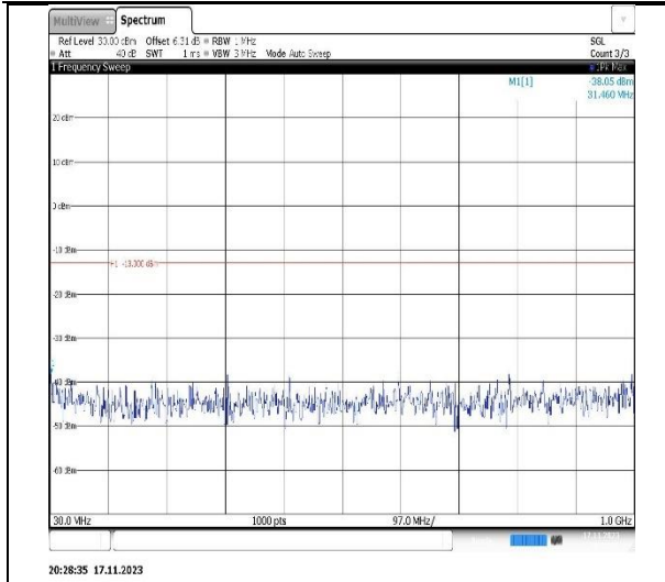
Band2-20MHz-QPSK-18700-1RB#0-Range1:30~1000MHz
