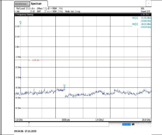
Band2-10MHz-QPSK-18900-1RB#0-Range2:1000~20000MHz
