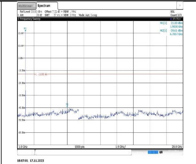
Band2-5MHz-QPSK-18625-1RB#0-Range2:1000~20000MHz
