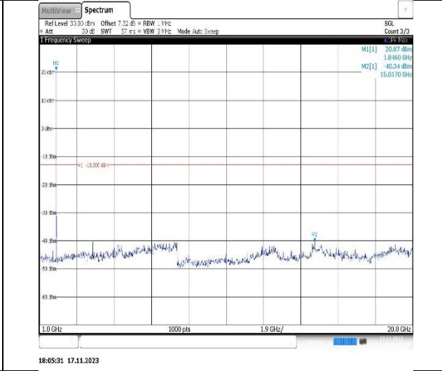
Band2-3MHz-QPSK-18900-1RB#0-Range2:1000~20000MHz
