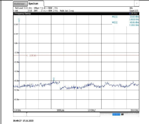
Band2-20MHz-QPSK-19100-1RB#0-Range2:1000~20000MHz
