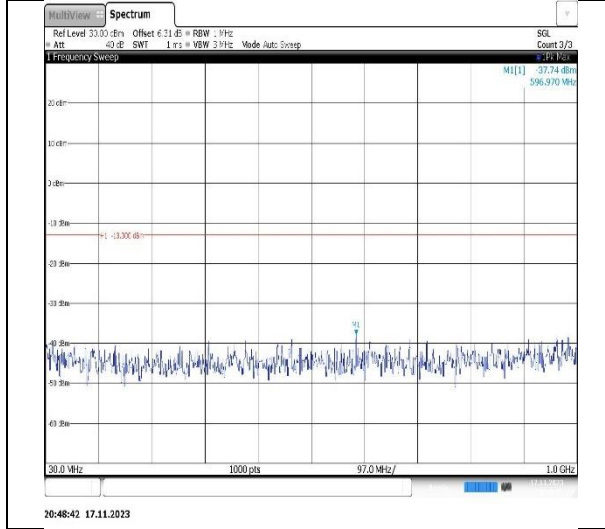
Band2-20MHz-QPSK-18900-1RB#0-Range1:30~1000MHz
