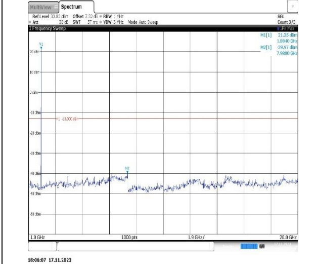
Band2-3MHz-QPSK-19185-1RB#0-Range2:1000~20000MHz
