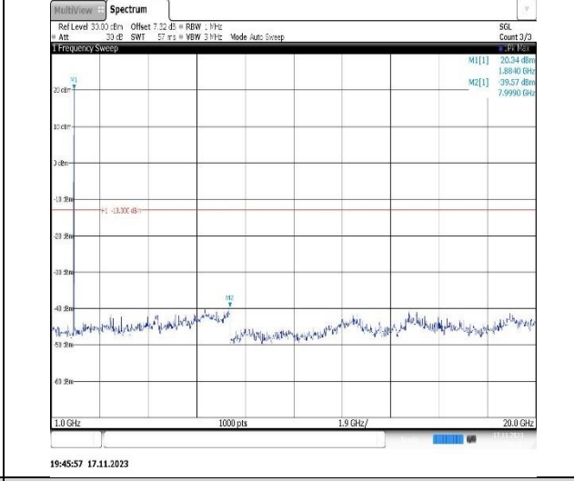
Band2-10MHz-QPSK-19150-1RB#0-Range2:1000~20000MHz
