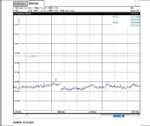
Band2-20MHz-QPSK-18900-1RB#0-Range2:1000~20000MHz
