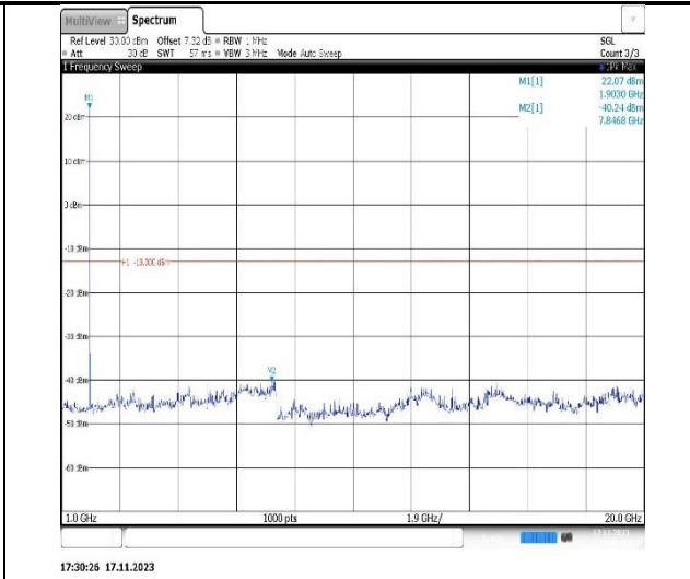
Band2-3MHz-QPSK-18615-1RB#0-Range2:1000~20000MHz
