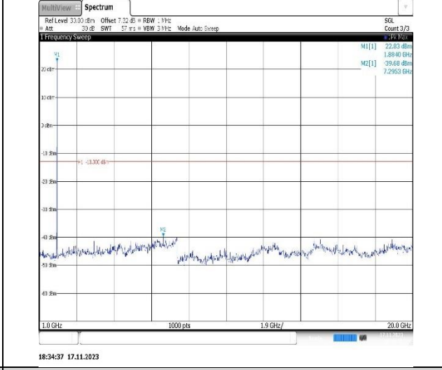
Band2-5MHz-QPSK-19175-1RB#0-Range2:1000~20000MHz
