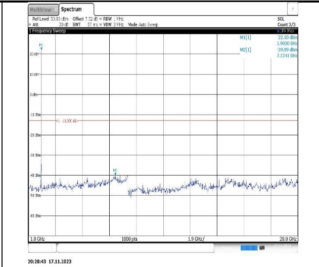
Band2-20MHz-QPSK-18700-1RB#0-Range2:1000~20000MHz
