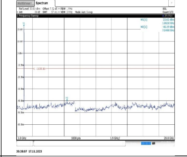
Band2-15MHz-QPSK-19125-1RB#0-Range2:1000~20000MHz
