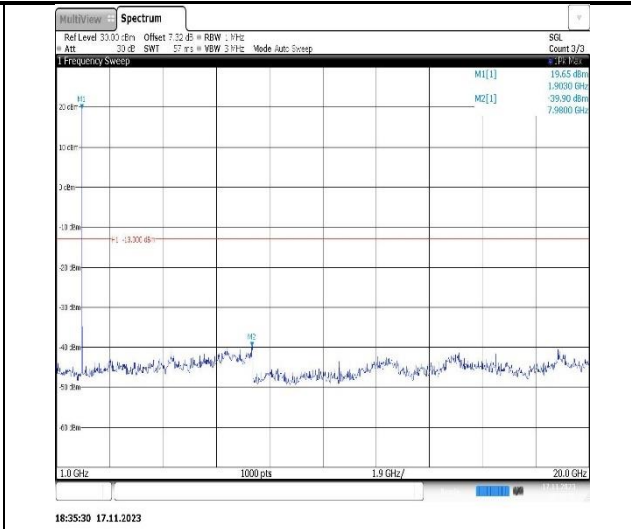
Band2-10MHz-QPSK-18650-1RB#0-Range2:1000~20000MHz
