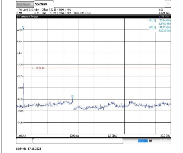
Band2-5MHz-QPSK-18900-1RB#0-Range2:1000~20000MHz
