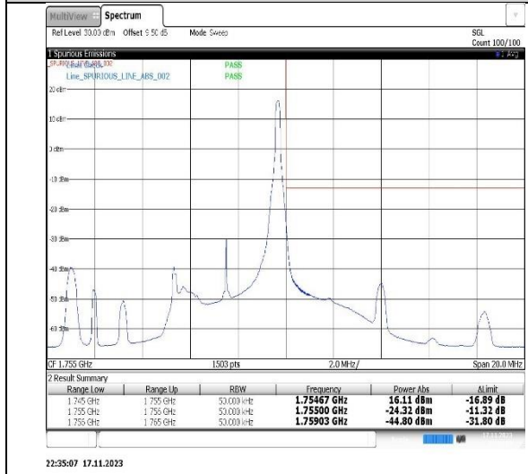
Band4-10MHz-QPSK-20000-1RB#0
