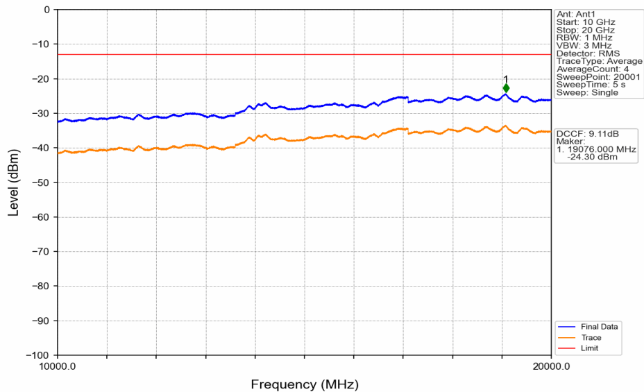
PCS1900_EGPRS_HCH_1909.8MHz_1 TX Slot_NTNV
