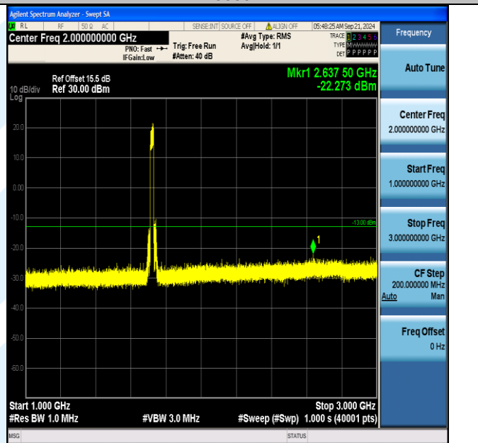
Band66_20MHz_QPSK_132072_100RB#0_1000~3000_1000~3000
