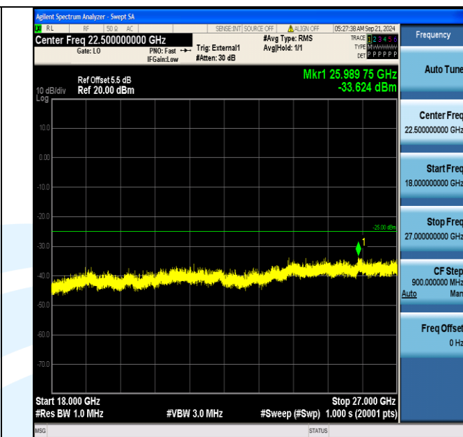
Band41_20MHz_16QAM_41140_100RB#0_18000~27000_1800~27000
