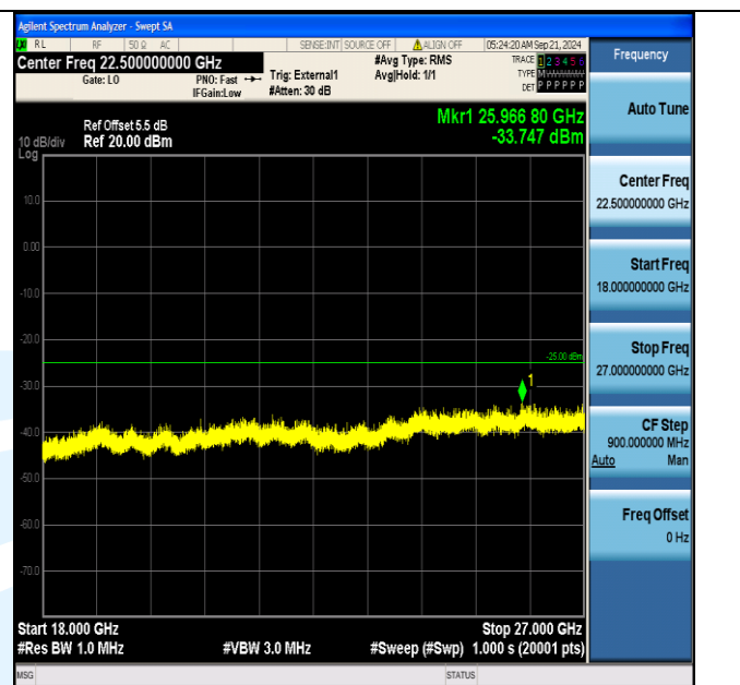
Band41_20MHz_16QAM_41140_1RB#99_18000~27000_18000~27000
