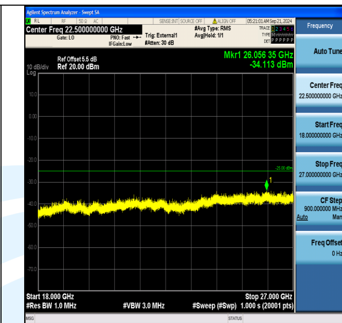
Band41_20MHz_16QAM_41140_1RB#0_18000~27000_18000~27000
