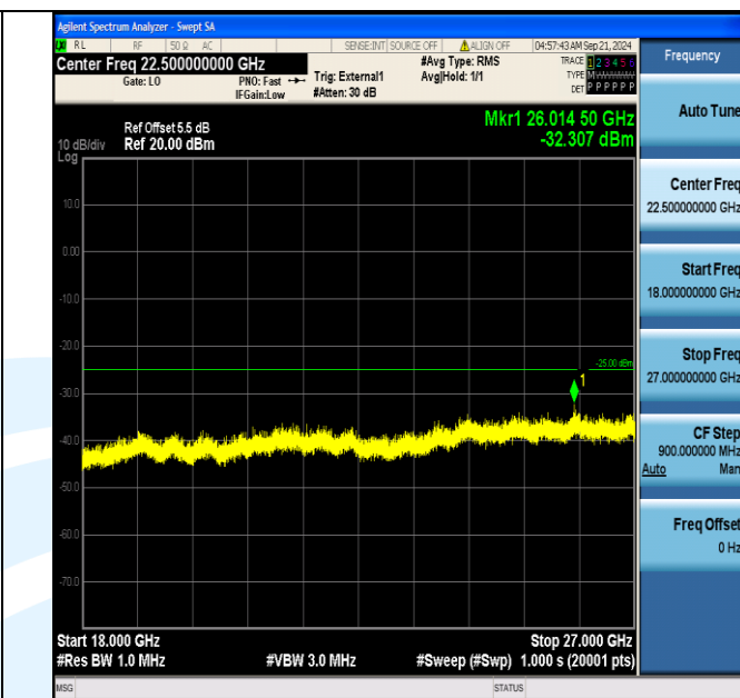
Band41_15MHz_16QAM_41165_75RB#0_18000~27000_18000~27000
