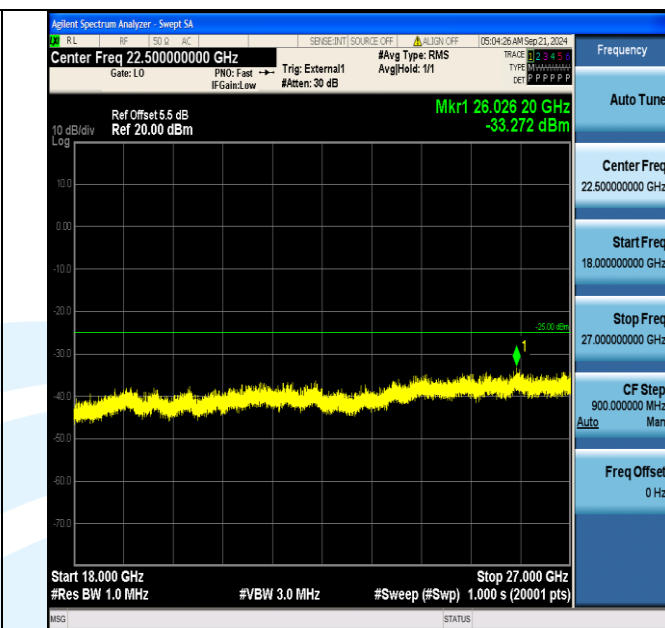
Band41_20MHz_16QAM_40340_1RB#99_18000~27000_18000~27000
