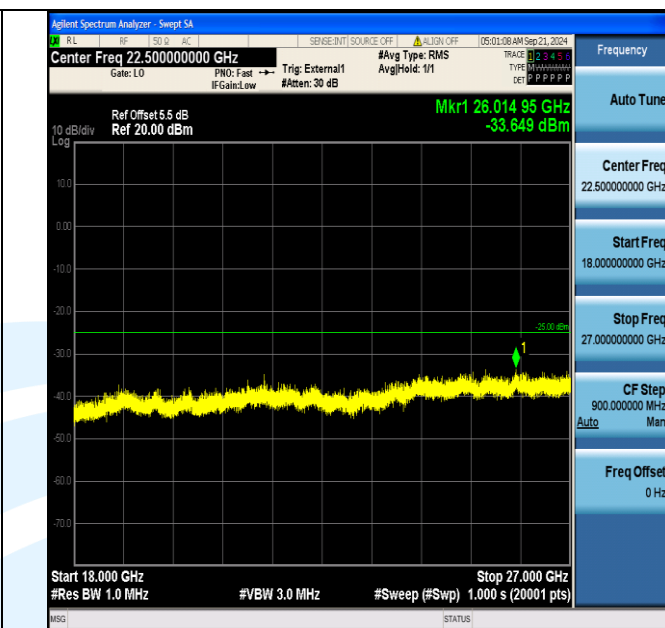
Band41_20MHz_16QAM_40340_1RB#0_18000~27000_18000~27000
