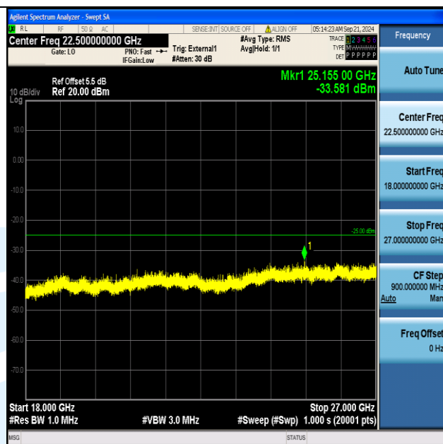
Band41_20MHz_16QAM_40690_1RB#99_18000~27000_18000~27000
