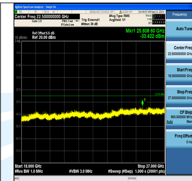
Band41_15MHz_QPSK_41165_1RB#0_18000~27000_18000~27000
