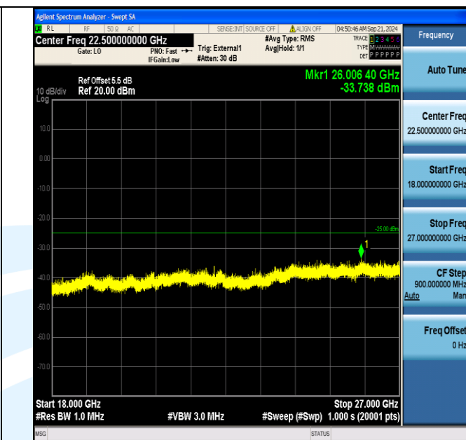
Band41_15MHz_16QAM_41165_1RB#0_18000~27000_18000~27000
