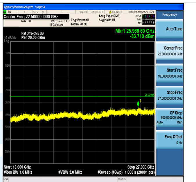
Band41_15MHz_16QAM_40690_1RB#0_18000~27000_18000~27000
