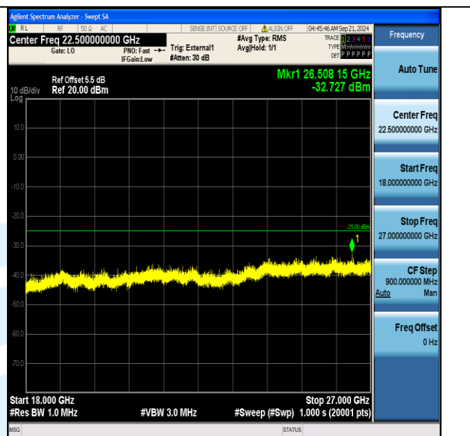
Band41_15MHz_QPSK_40690_75RB#0_18000~27000_18000~27000
