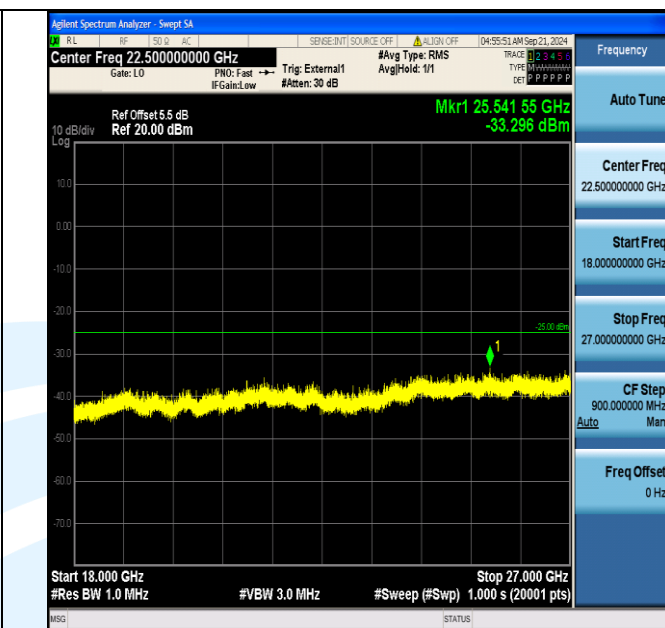
Band41_15MHz_QPSK_41165_75RB#0_18000~27000_18000~27000
