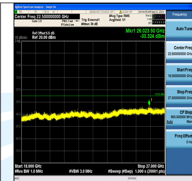
Band41_15MHz_16QAM_40690_1RB#74_18000~27000_18000~27000
