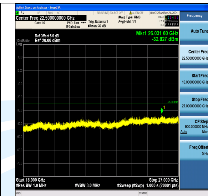
Band41_15MHz_16QAM_40690_75RB#0_18000~27000_18000~27000
