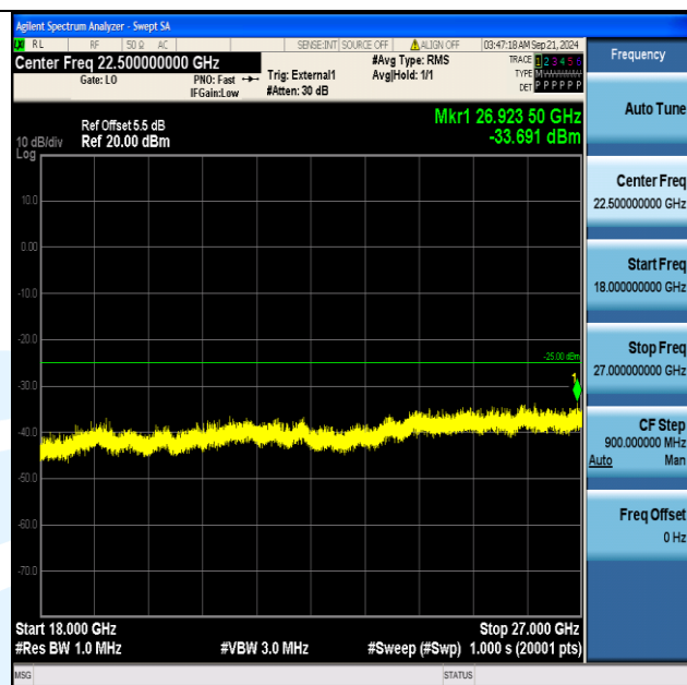
Band41_5MHz_16QAM_40690_25RB#0_18000~27000_18000~27000
