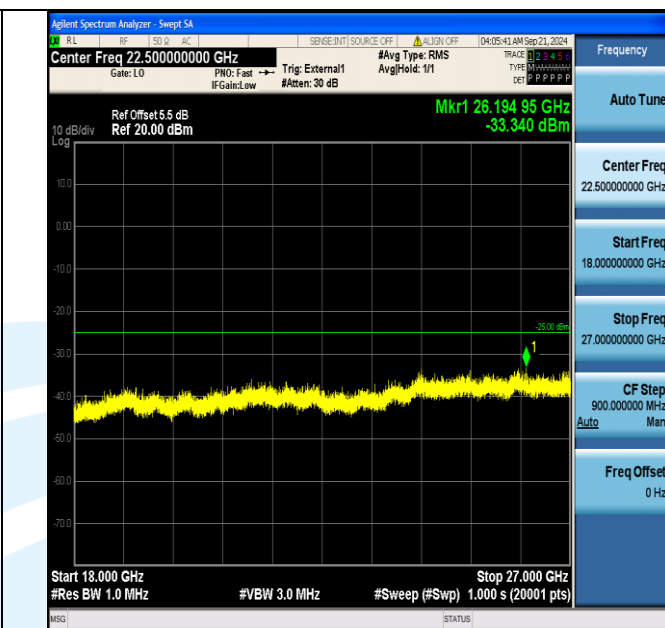
Band41_10MHz_QPSK_40290_50RB#0_18000~27000_18000~27000
