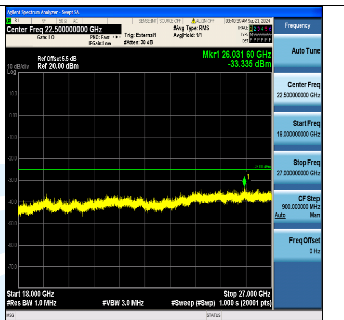
Band41_5MHz_16QAM_40690_1RB#0_18000~27000_18000~27000
