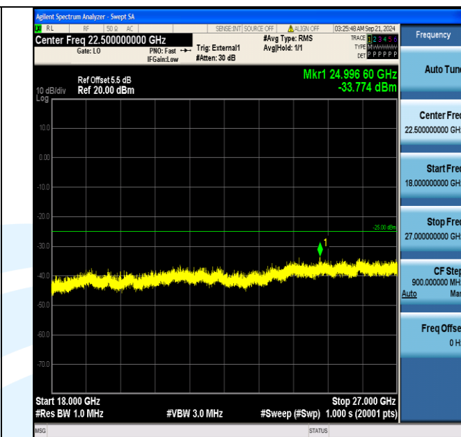
Band38_20MHz_16QAM_38150_100RB#0_18000~27000_18000~27000
