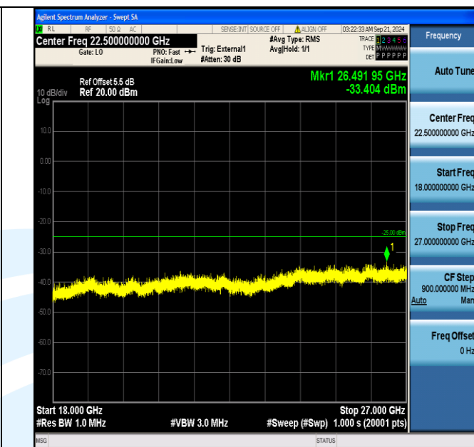
Band38_20MHz_16QAM_38150_1RB#99_18000~27000_18000~27000
