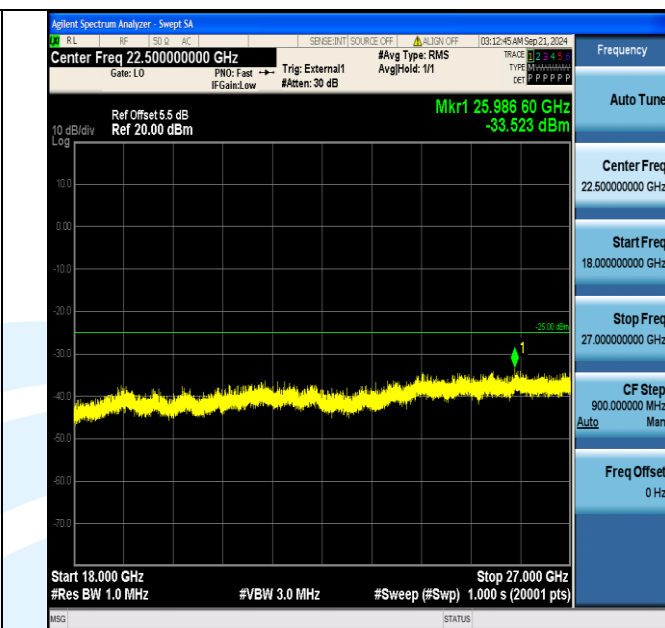
Band38_20MHz_16QAM_38000_1RB#99_18000~27000_18000~27000
