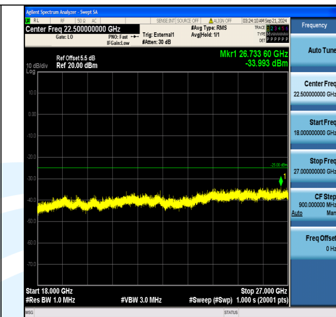
Band38_20MHz_QPSK_38150_100RB#0_18000~27000_18000~27000
