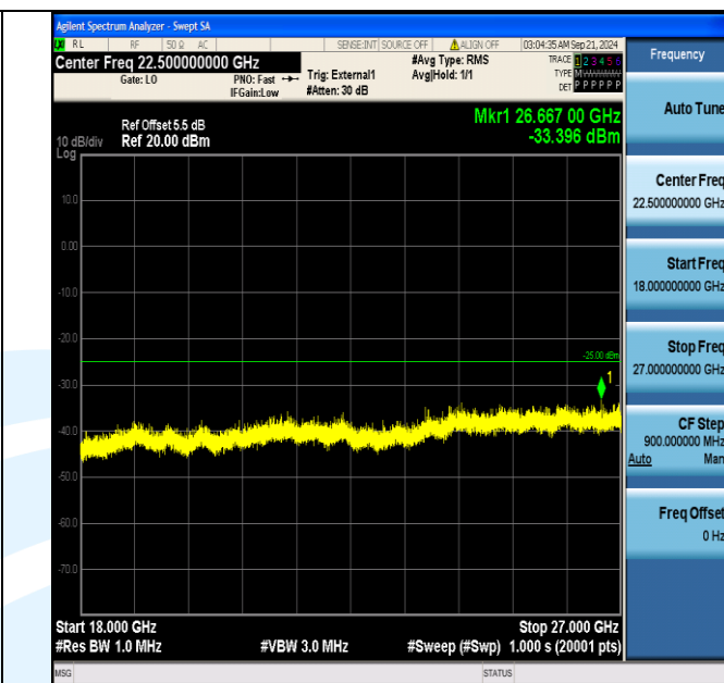
Band38_20MHz_QPSK_37850_100RB#0_18000~27000_18000~27000
