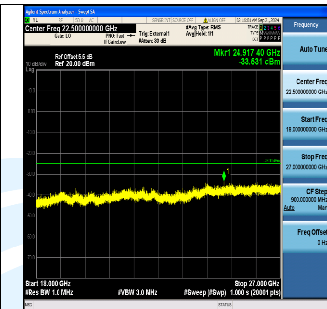
Band38_20MHz_16QAM_38000_100RB#0_18000~27000_18000~27000
