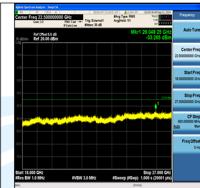
Band38_20MHz_16QAM_38000_1RB#0_18000~27000_18000~27000
