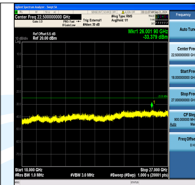
Band38_20MHz_QPSK_38000_1RB#99_18000~27000_18000~27000
