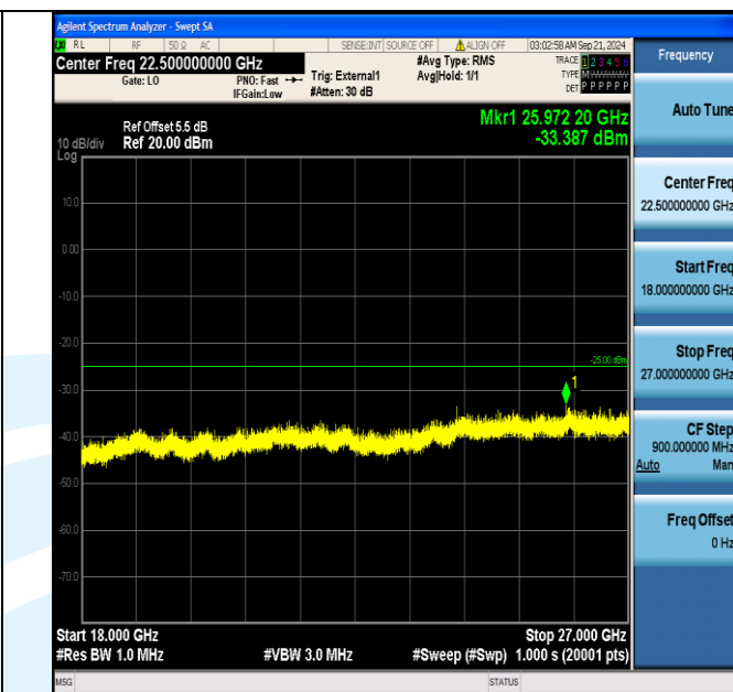
Band38_20MHz_16QAM_37850_1RB#99_18000~27000_18000~27000
