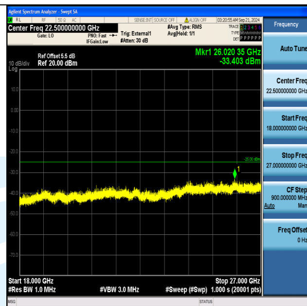
Band38_20MHz_QPSK_38150_1RB#99_18000~27000_18000~27000
