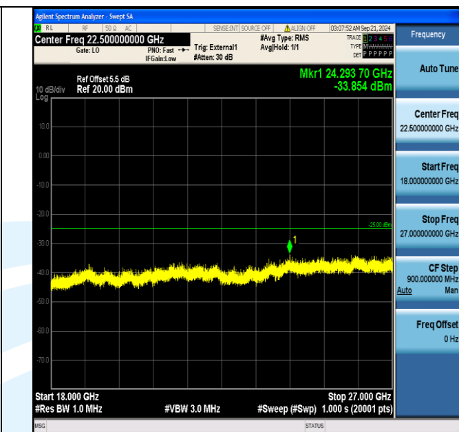
Band38_20MHz_QPSK_38000_1RB#0_18000~27000_18000~27000
