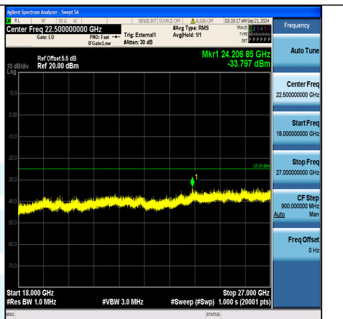
Band38_20MHz_16QAM_38150_1RB#0_18000~27000_18000~27000
