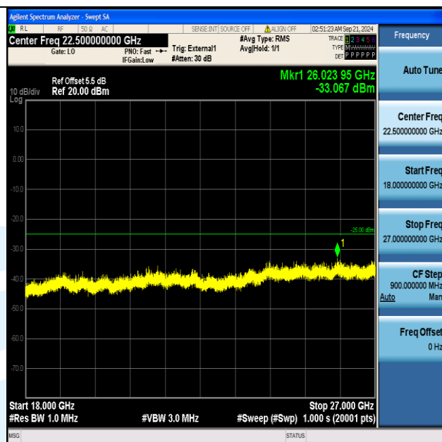
Band38_15MHz_QPSK_38175_1RB#74_18000~27000_18000~27000
