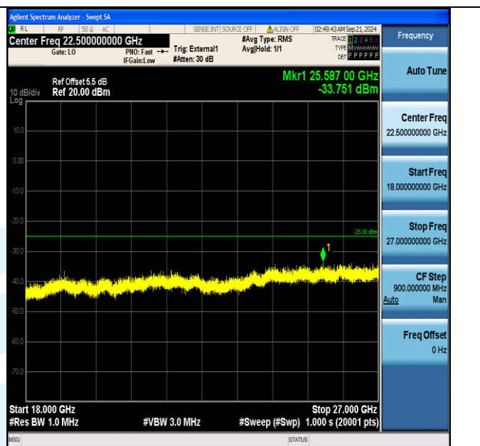
Band38_15MHz_16QAM_38175_1RB#0_18000~27000_18000~27000
