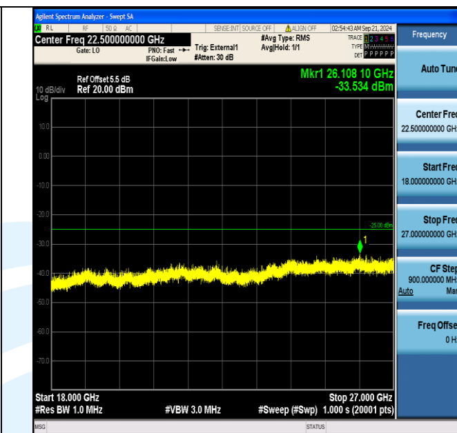
Band38_15MHz_QPSK_38175_75RB#0_18000~27000_18000~27000
