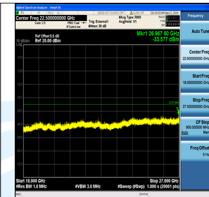
Band38_15MHz_16QAM_38000_1RB#74_18000~27000_18000~27000
