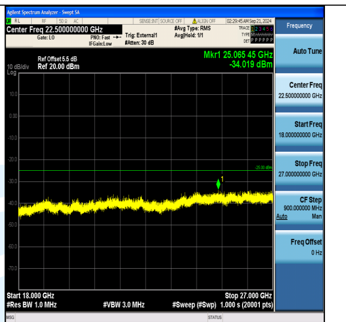
Band38_15MHz_16QAM_37825_1RB#0_18000~27000_18000~27000
