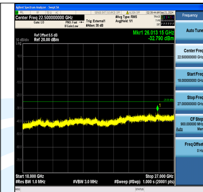
Band38_15MHz_16QAM_38000_1RB#0_18000~27000_18000~27000
