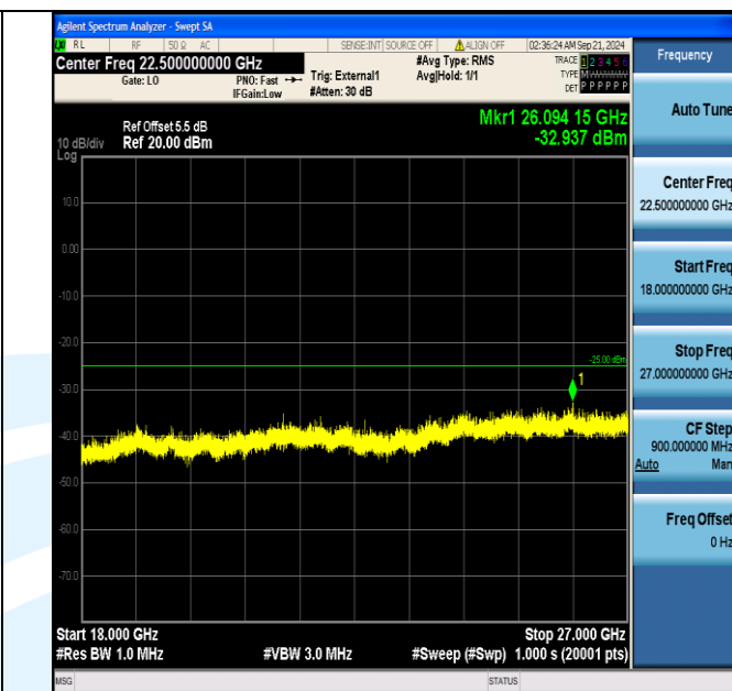
Band38_15MHz_16QAM_37825_75RB#0_18000~27000_18000~27000
