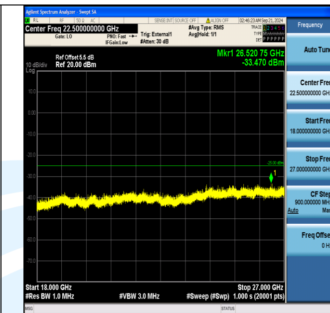
Band38_15MHz_16QAM_38000_75RB#0_18000~27000_18000~27000
