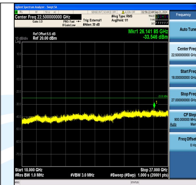
Band38_15MHz_16QAM_38175_75RB#0_18000~27000_18000~27000
