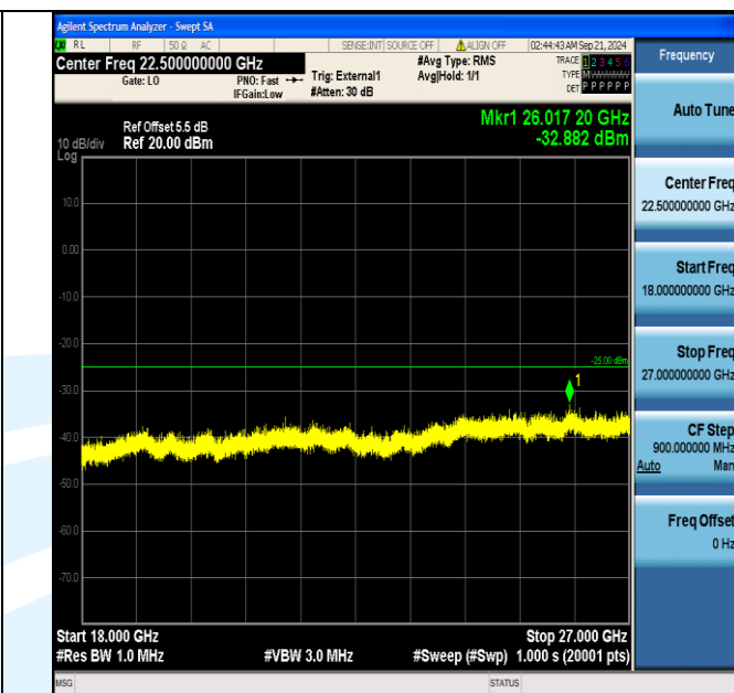
Band38_15MHz_QPSK_38000_75RB#0_18000~27000_18000~27000
