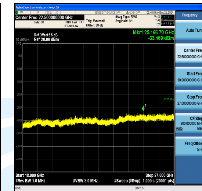
Band38_15MHz_QPSK_38175_1RB#0_18000~27000_18000~27000
