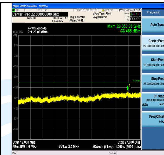
Band38_15MHz_16QAM_38175_1RB#74_18000~27000_18000~27000
