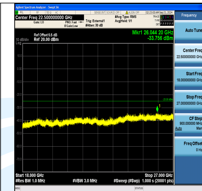
Band38_10MHz_16QAM_38200_1RB#49_18000~27000_18000~27000
