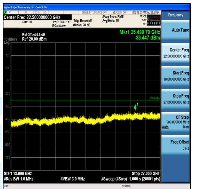
Band38_15MHz_QPSK_38000_1RB#0_18000~27000_18000~27000
