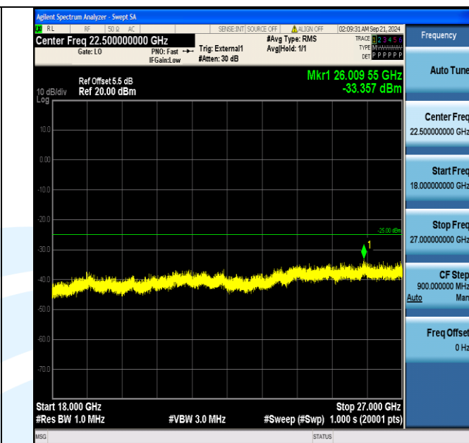
Band38_10MHz_16QAM_38000_1RB#0_18000~27000_18000~27000
