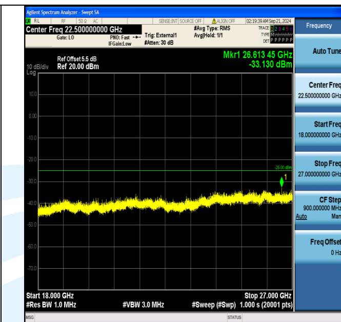
Band38_10MHz_16QAM_38200_1RB#0_18000~27000_18000~27000
