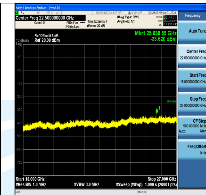
Band38_10MHz_16QAM_38200_50RB#0_18000~27000_18000~27000
