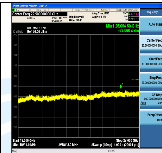
Band38_10MHz_16QAM_38000_50RB#0_18000~27000_18000~27000
