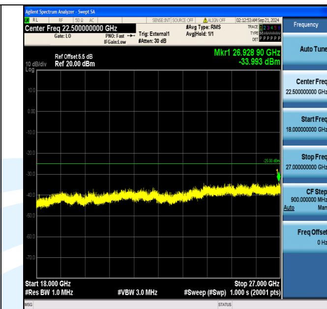
Band38_10MHz_16QAM_38000_1RB#49_18000~27000_18000~27000
