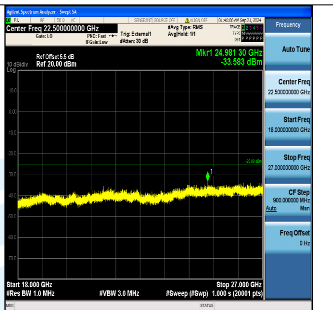
Band38_5MHz_16QAM_38000_25RB#0_18000~27000_18000~27000
