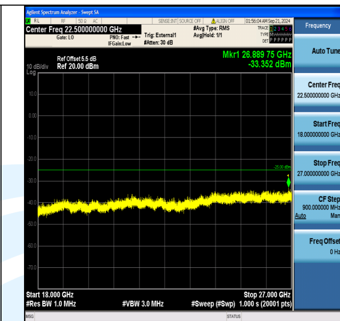
Band38_5MHz_16QAM_38225_25RB#0_18000~27000_18000~27000
