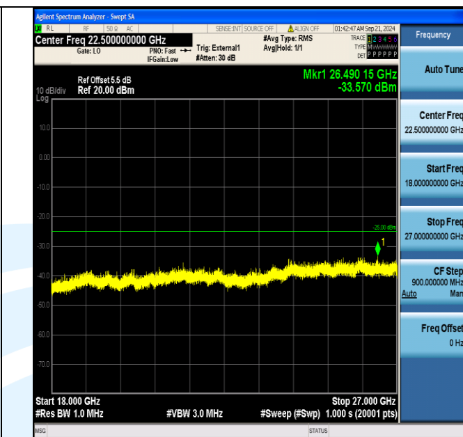
Band38_5MHz_16QAM_38000_1RB#24_18000~27000_18000~27000
