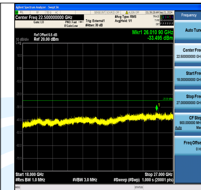
Band38_5MHz_16QAM_38000_1RB#0_18000~27000_18000~27000
