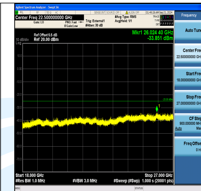
Band38_5MHz_16QAM_38225_1RB#0_18000~27000_18000~27000
