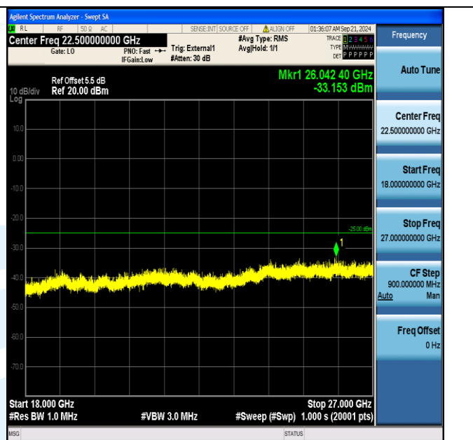
Band38_5MHz_16QAM_37775_25RB#0_18000~27000_18000~27000
