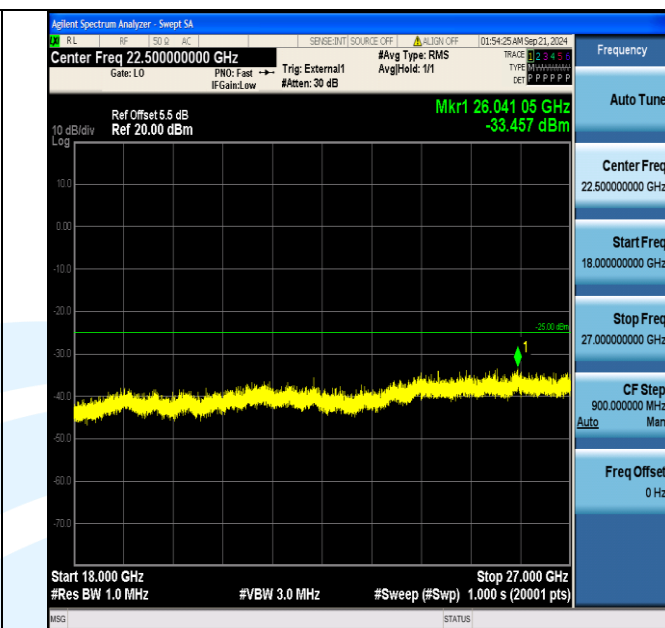
Band38_5MHz_QPSK_38225_25RB#0_18000~27000_18000~27000
