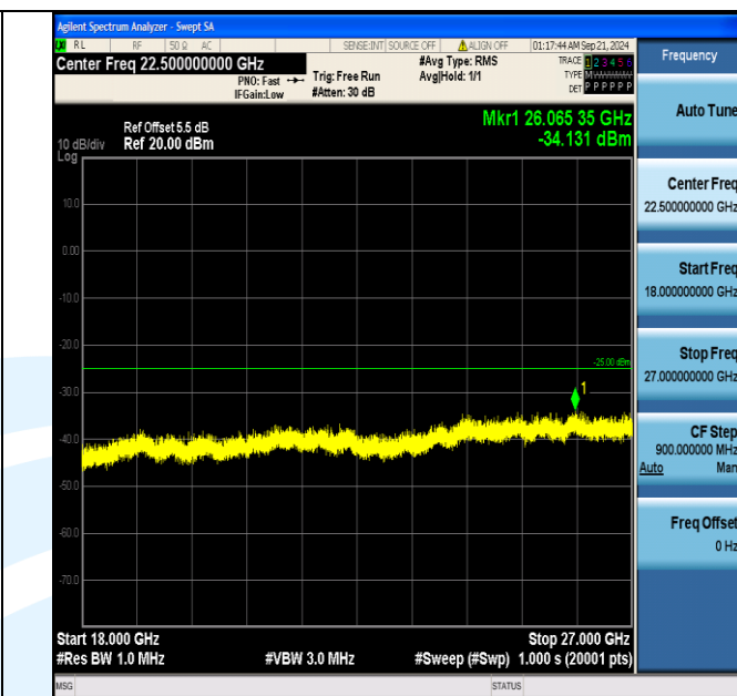
Band7_20MHz_16QAM_21350_1RB#99_18000~27000_18000~27000
