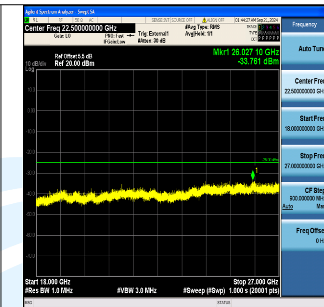
Band38_5MHz_QPSK_38000_25RB#0_18000~27000_18000~27000
