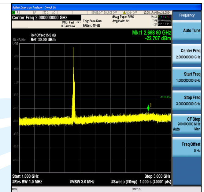
Band4 20MHz QPSK 20050 1RB#0 1000~3000 1000~3000
