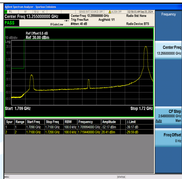
Band66 10MHz QPSK 132022 1RB#49
