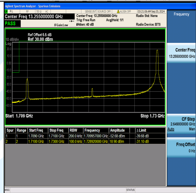
Band66 20MHz 16QAM 132072 1RB#99
