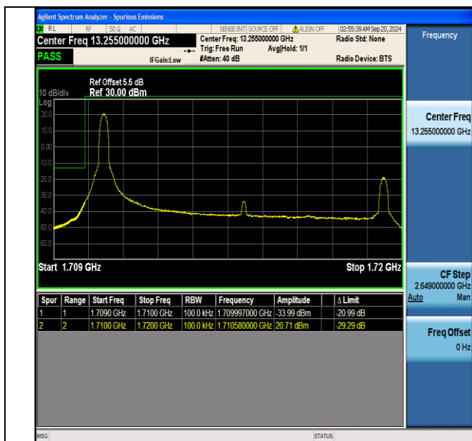
Band66 10MHz QPSK 132022 1RB#0
