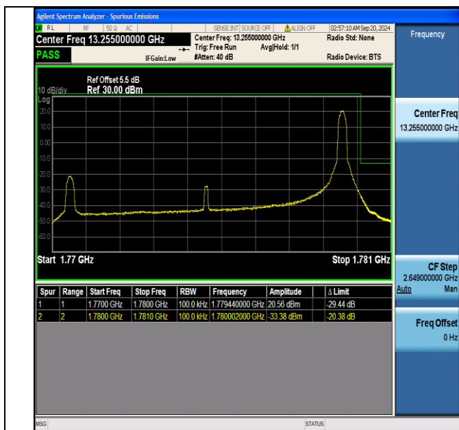
Band66 10MHz QPSK 132622 1RB#49
