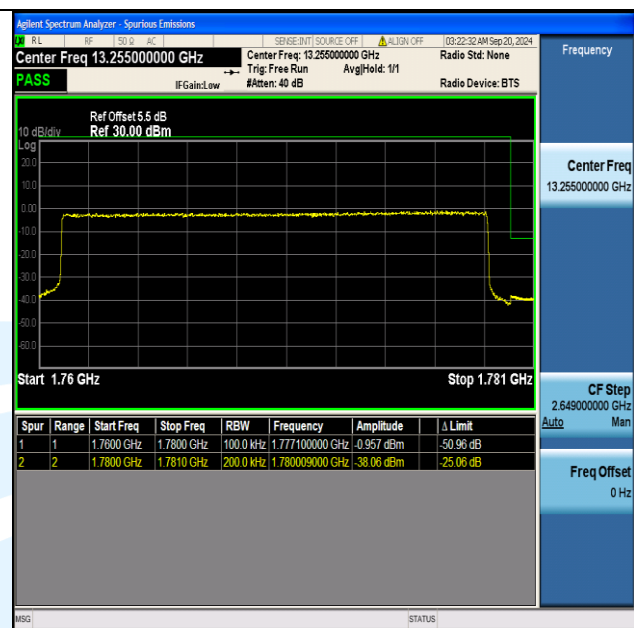
Band66 20MHz QPSK 132572 100RB#0
