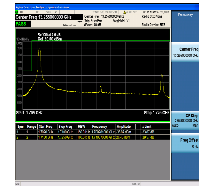
Band66 15MHz QPSK 132047 1RB#0
