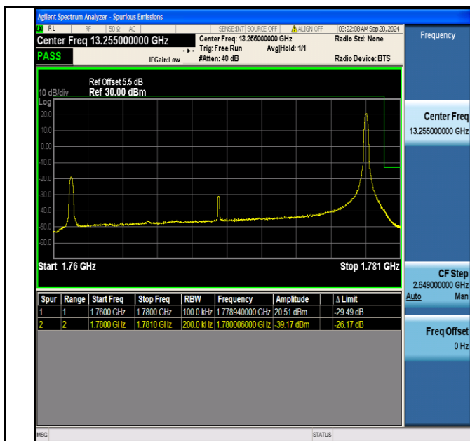
Band66 20MHz QPSK 132572 1RB#99
