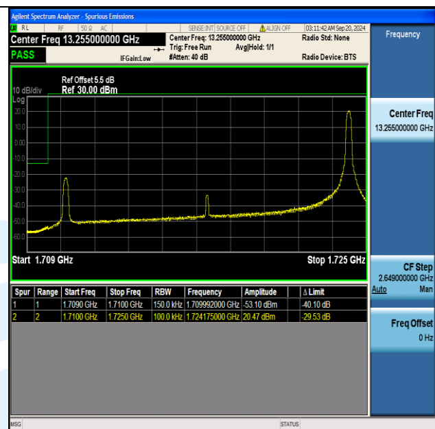
Band66 15MHz QPSK 132047 1RB#74
