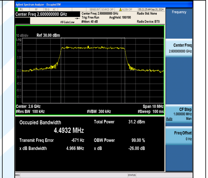
Band41(2555-2655)-5MHz-QPSK-40690-25RB#0-PASS
