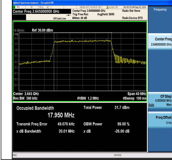
Band41(2555-2655)-20MHz-QPSK-41140-100RB#0-PASS
