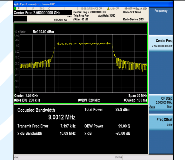
Band41(2555-2655)-10MHz-16QAM-40290-50RB#0-PASS
