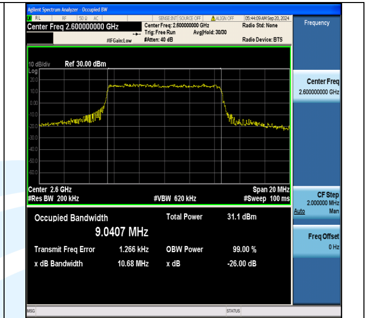
Band41(2555-2655)-10MHz-QPSK-40690-50RB#0-PASS
