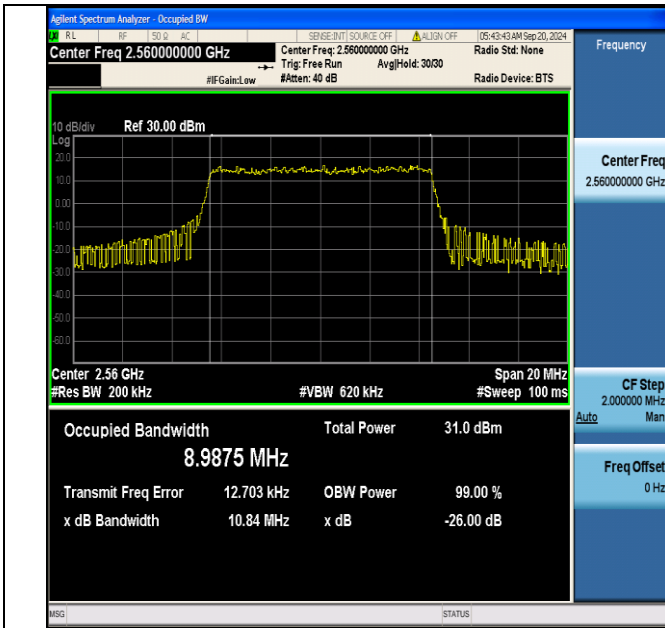
Band41(2555-2655)-10MHz-QPSK-40290-50RB#0-PASS
