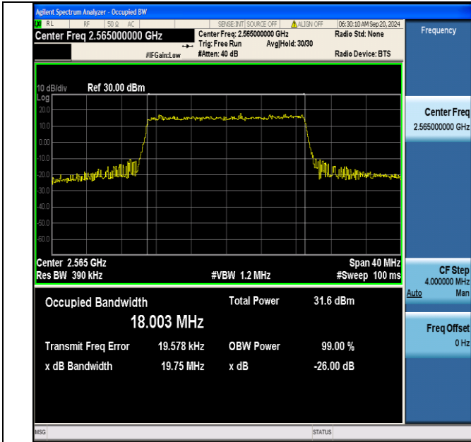
Band41(2555-2655)-20MHz-QPSK-40340-100RB#0-PASS
