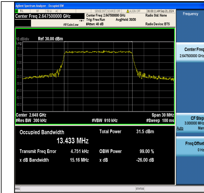
Band41(2555-2655)-15MHz-QPSK-41165-75RB#0-PASS
