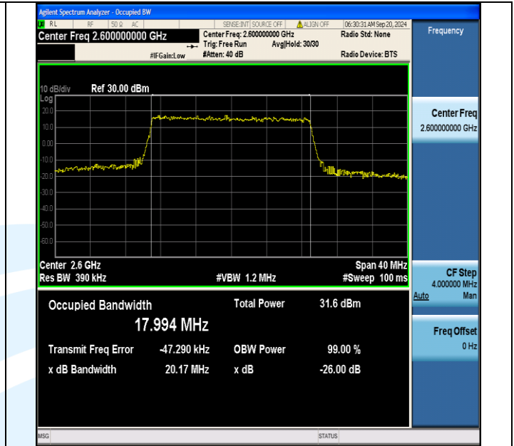
Band41(2555-2655)-20MHz-QPSK-40690-100RB#0-PASS
