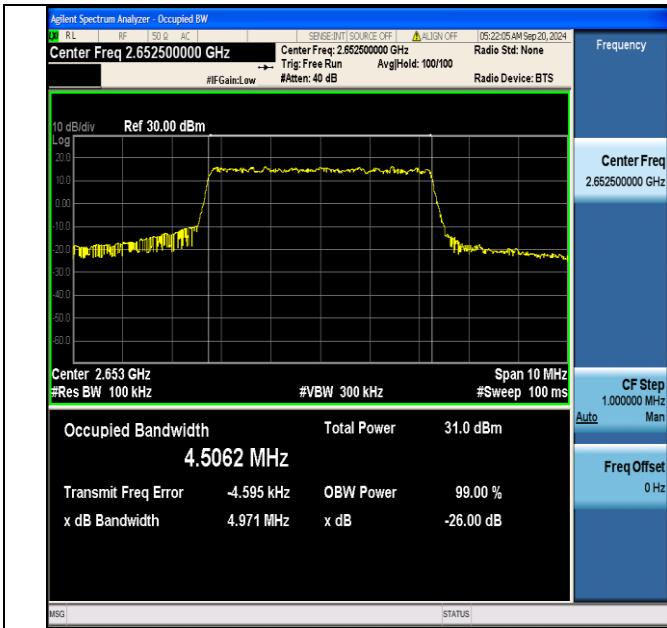
Band41(2555-2655)-5MHz-QPSK-41215-25RB#0-PASS
