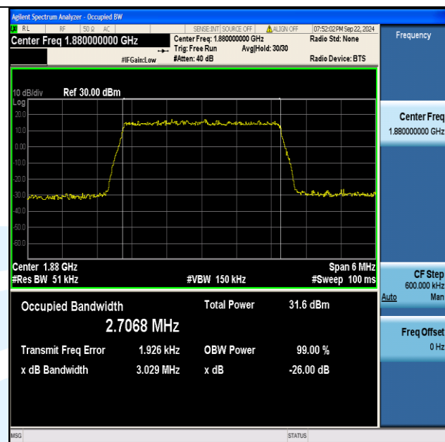
Band2-3MHz-QPSK-18900-15RB#0-PASS
