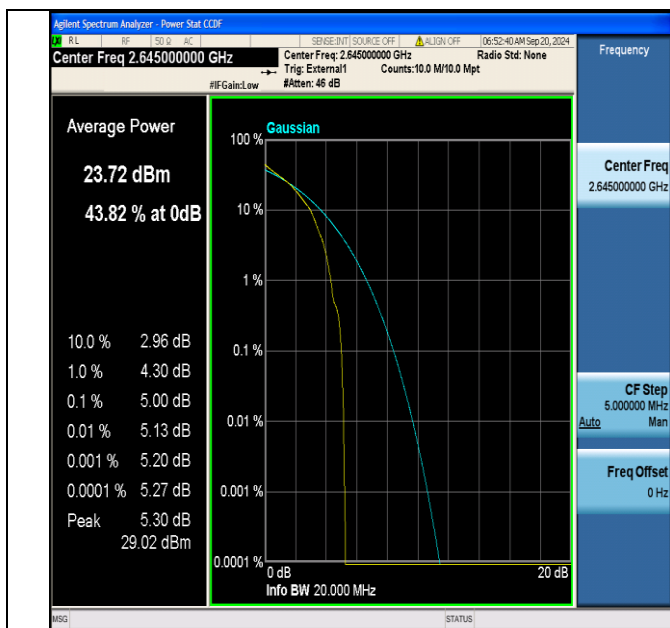
Band41(2555-2655)-20MHz-QPSK-41140-1RB#0-PASS
