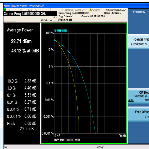
Band41(2555-2655)-20MHz-QPSK-40340-100RB#0-PASS
