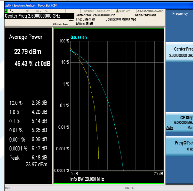
Band41(2555-2655)-20MHz-QPSK-40690-100RB#0-PASS
