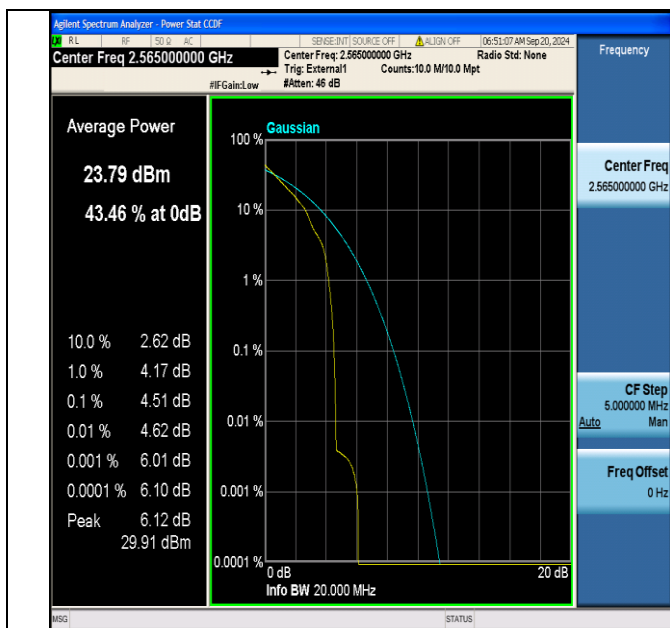
Band41(2555-2655)-20MHz-QPSK-40340-1RB#0-PASS
