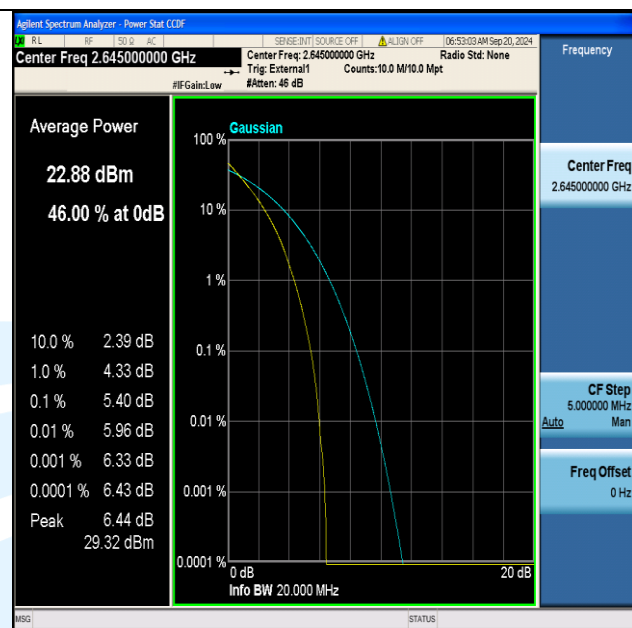
Band41(2555-2655)-20MHz-QPSK-41140-100RB#0-PASS
