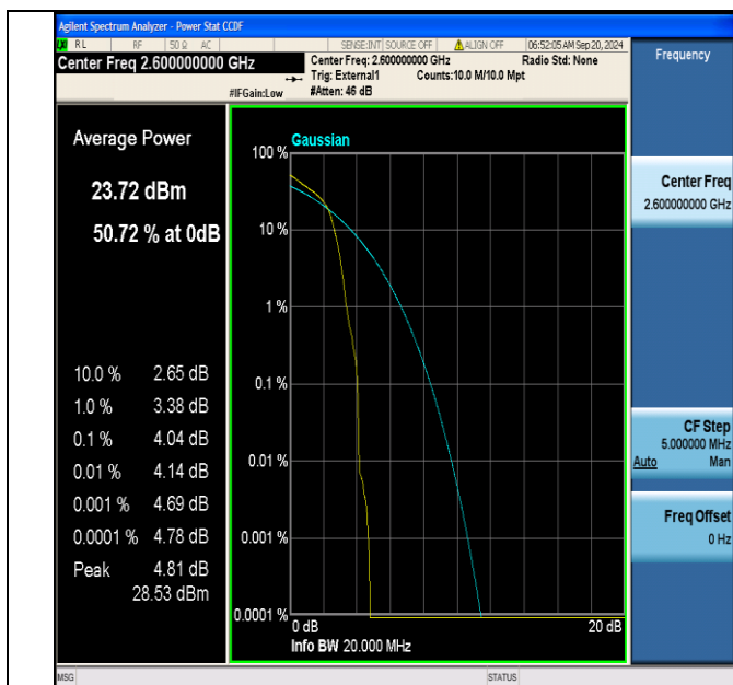
Band41(2555-2655)-20MHz-16QAM-40690-1RB#0-PASS
