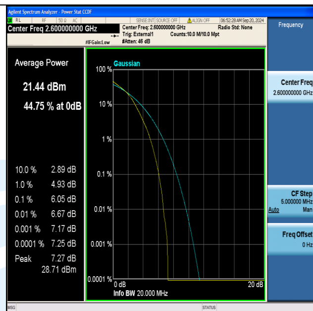
Band41(2555-2655)-20MHz-16QAM-40690-100RB#0-PASS
