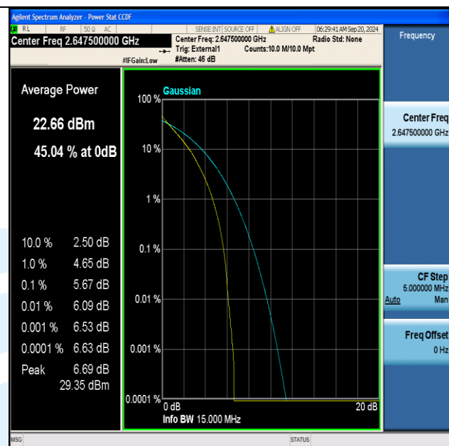
Band41(2555-2655)-15MHz-QPSK-41165-75RB#0-PASS
