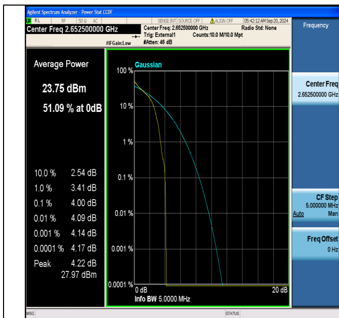
Band41(2555-2655)-5MHz-QPSK-41215-1RB#0-PASS
