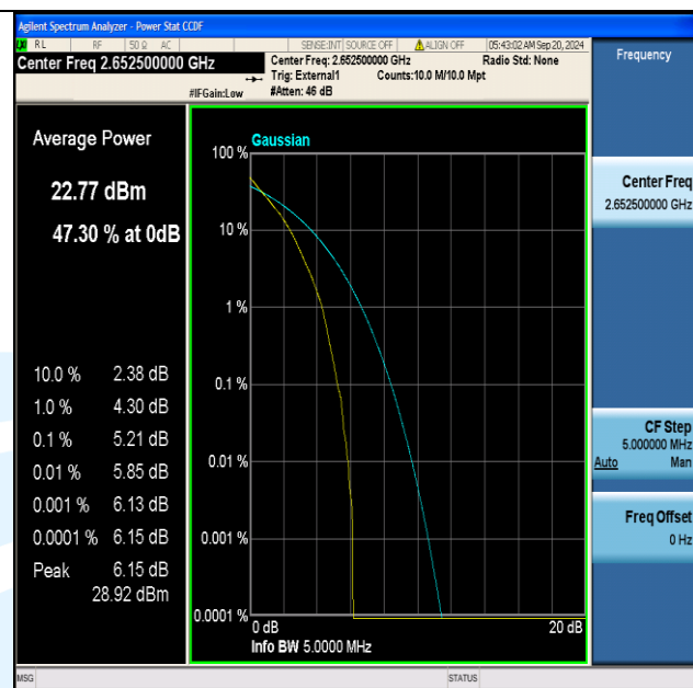
Band41(2555-2655)-5MHz-QPSK-41215-25RB#0-PASS
