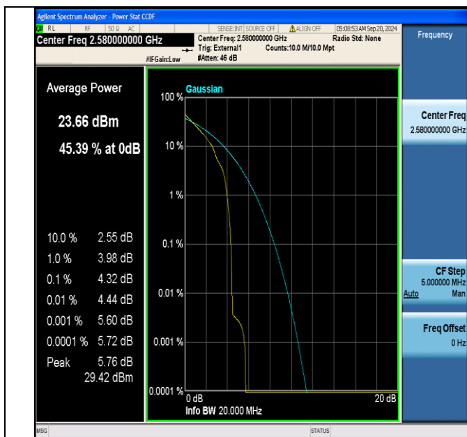
Band38-20MHz-QPSK-37850-1RB#0-PASS
