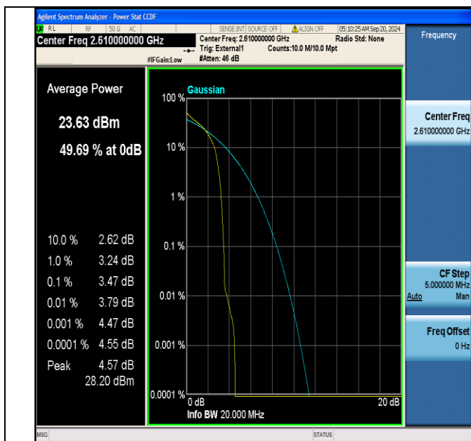
Band38-20MHz-QPSK-38150-1RB#0-PASS
