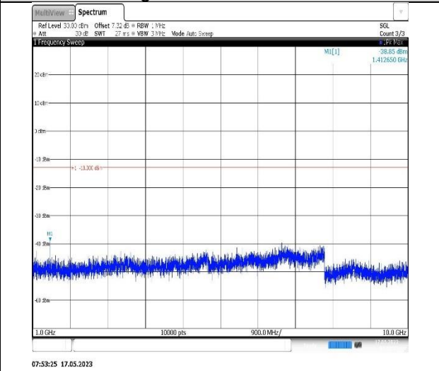
Band12-3MHz-QPSK-23165-1RB#0-Range2:1000~10000MHz
