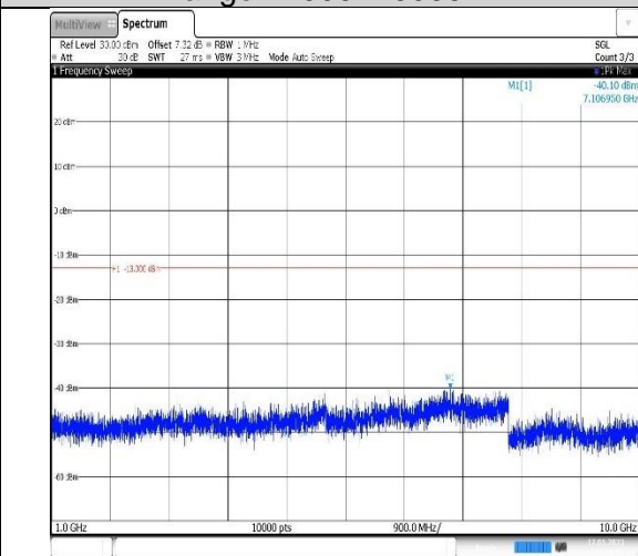
Band12-5MHz-QPSK-23155-1RB#0- Range2:1000~10000MHz
