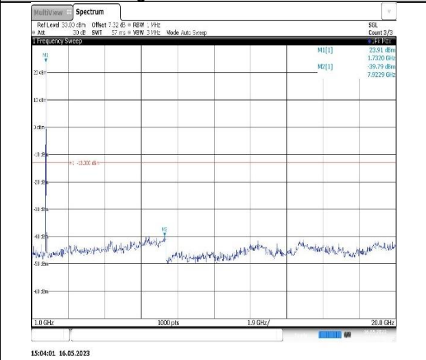
Band4-20MHz-QPSK-20300-1RB#0-Range2:1000~20000MHz
