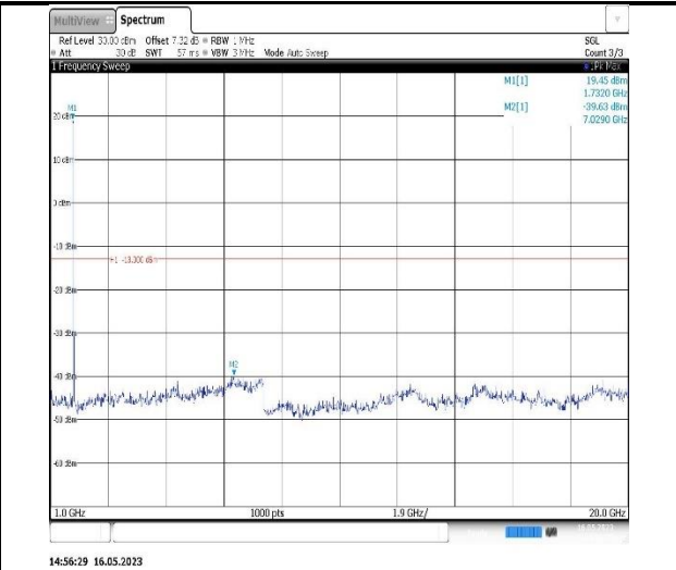
Band4-20MHz-QPSK-20050-1RB#0-Range2:1000~20000MHz
