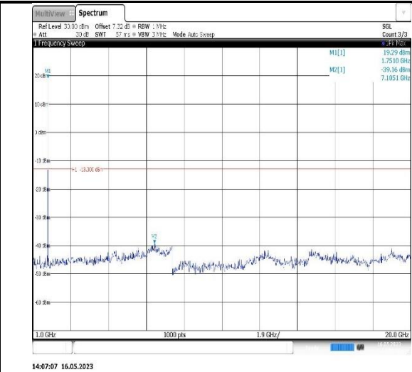
Band4-10MHz-QPSK-20000-1RB#0-Range2:1000~20000MHz
