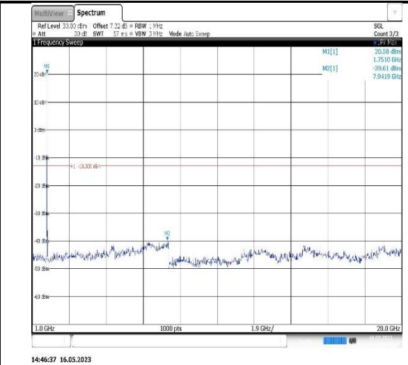
Band4-15MHz-QPSK-20025-1RB#0-Range2:1000~20000MHz
