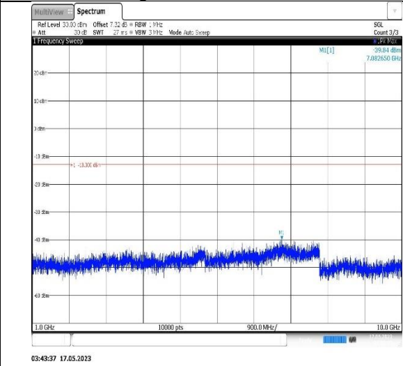
Band5-5MHz-QPSK-20525-1RB#0- Range2:1000~10000MHz
