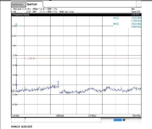
Band4-5MHz-QPSK-20375-1RB#0- Range2:1000~20000MHz
