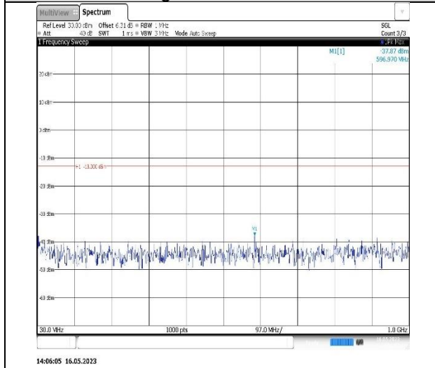
Band4-5MHz-QPSK-20375-1RB#0- Range1:30~1000MHz
