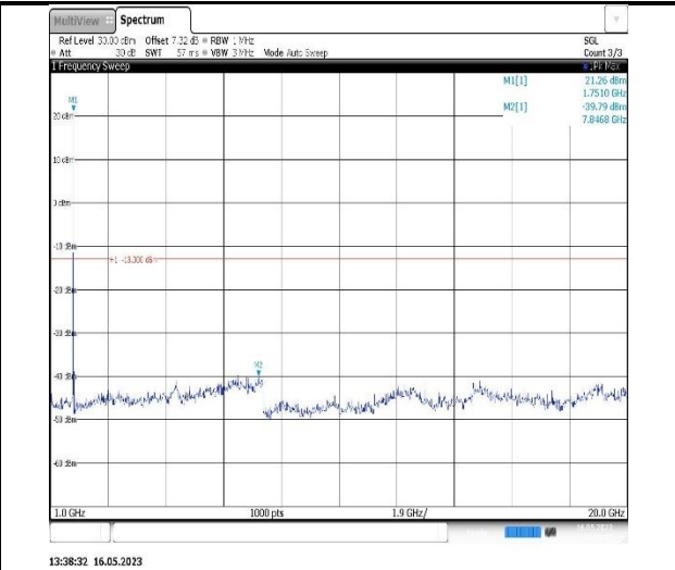
Band4-5MHz-QPSK-19975-1RB#0- Range2:1000~20000MHz
