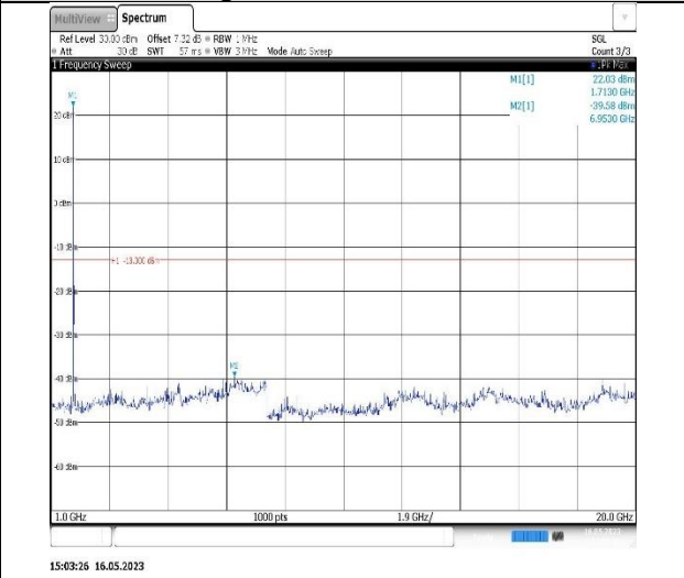
Band4-20MHz-QPSK-20175-1RB#0-Range2:1000~20000MHz
