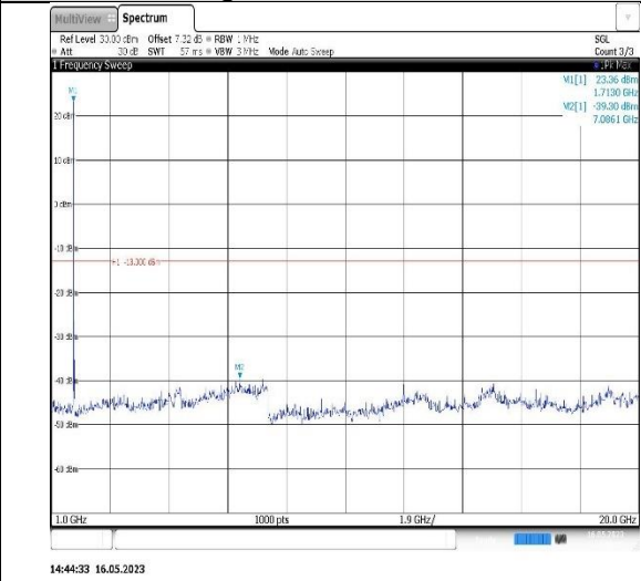
Band4-10MHz-QPSK-20175-1RB#0-Range2:1000~20000MHz
