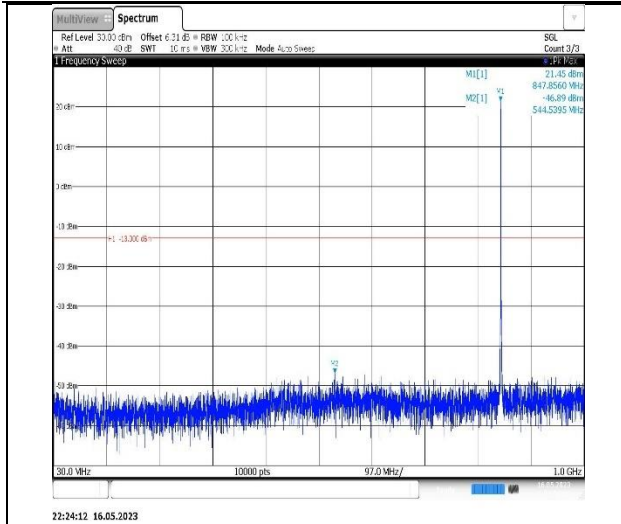
Band5-3MHz-QPSK-20415-1RB#0- Range1:30~1000MHz
