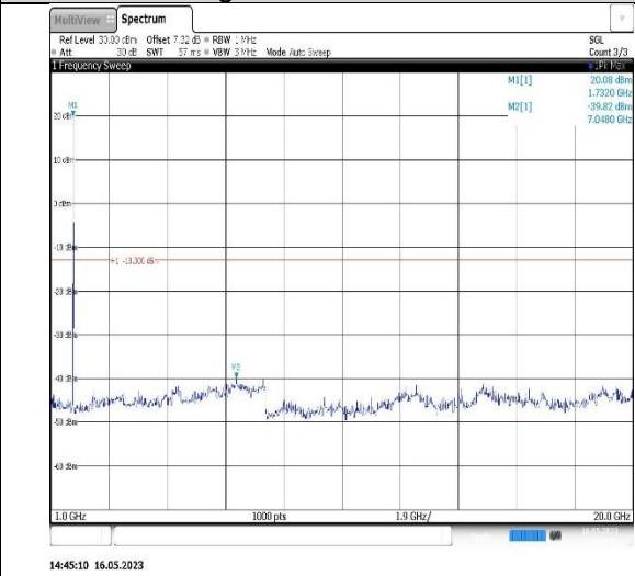
Band4-10MHz-QPSK-20350-1RB#0-Range2:1000~20000MHz
