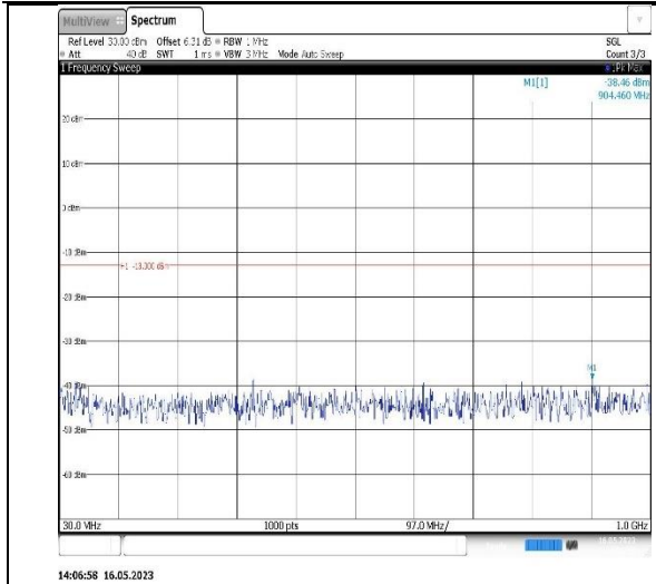
Band4-10MHz-QPSK-20000-1RB#0-Range1:30~1000MHz
