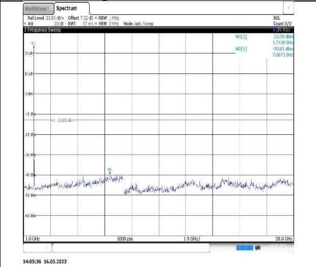
Band4-5MHz-QPSK-20175-1RB#0- Range2:1000~20000MHz
