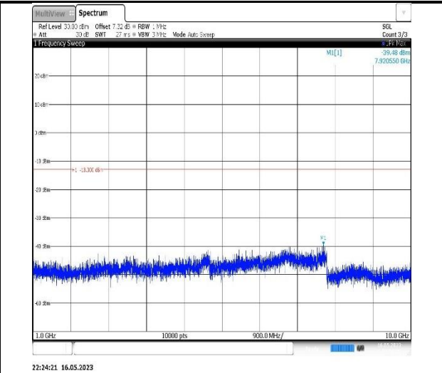
Band5-3MHz-QPSK-20415-1RB#0- Range2:1000~10000MHz
