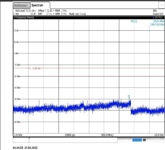
Band5-5MHz-QPSK-20425-1RB#0- Range2:1000~10000MHz
