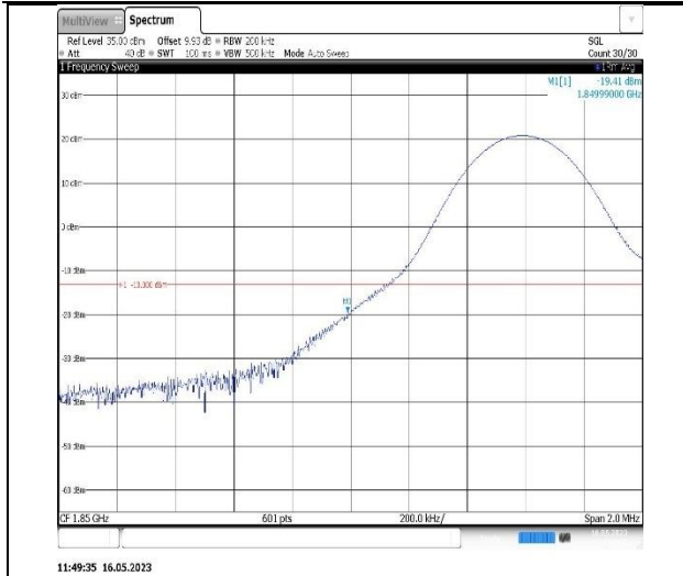
Band2-10MHz-QPSK-18650-50RB#0
