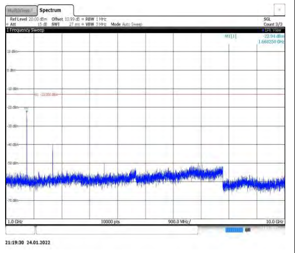
Band5-5MHz-QPSK-20525-1RB#0-Range2:10 00~10000MHz
