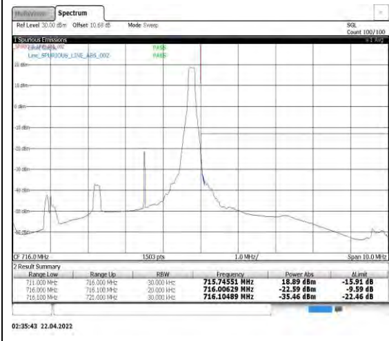
Band12-3MHz-QPSK-23165-1RB#14
