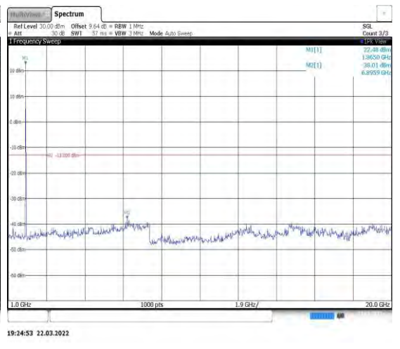
Band2-20MHz-QPSK-18900-1RB#0-Range2:1 000~20000MHz
