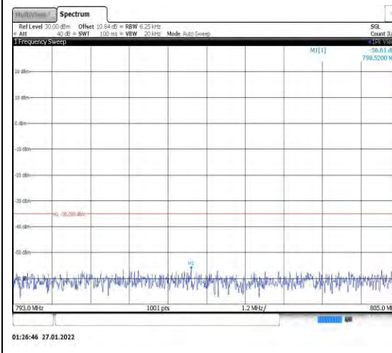
Band13-5MHz-QPSK-23255-1RB#0-Range 4:793~805MHz
