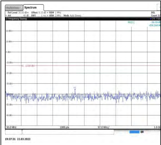
Band4-10MHz-QPSK-20000-1RB#0-Range 1:30~1000MHz
