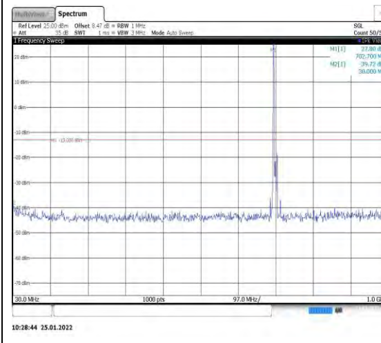
Band12-10MHz-QPSK-23095-1RB#0-Rang e1:30~1000MHz
