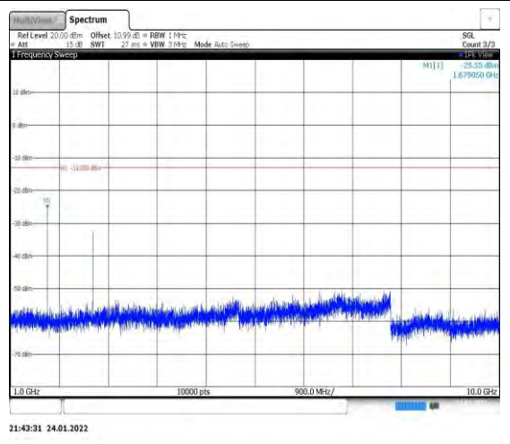
Band5-10MHz-QPSK-20600-1RB#0-Range2:1 000~10000MHz
