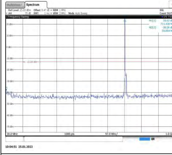
Band12-5MHz-QPSK-23155-1RB#0-Range 1:30~1000MHz
