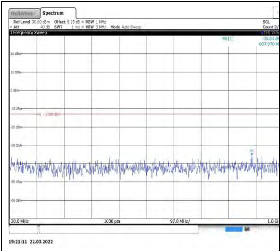
Band2-10MHz-QPSK-18650-1RB#0-Range 1:30~1000MHz
