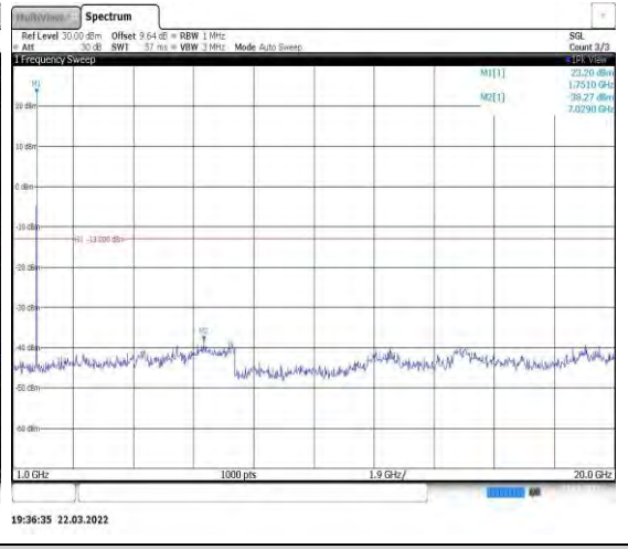
Band4-5MHz-QPSK-20375-1RB#0-Range2:10 00~20000MHz
