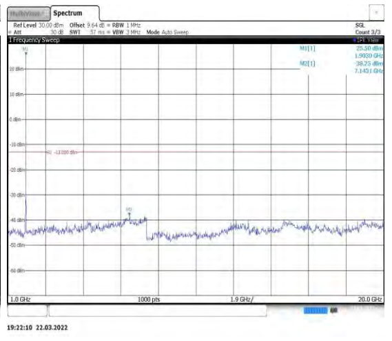
Band2-10MHz-QPSK-19150-1RB#0-Range2:1 000~20000MHz
