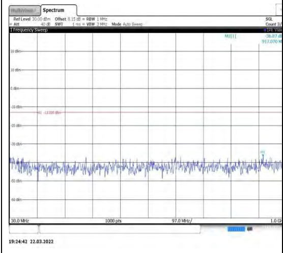
Band2-20MHz-QPSK-18900-1RB#0-Range 1:30~1000MHz
