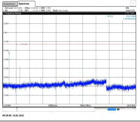
Band12-3MHz-QPSK-23165-1RB#0-Range2:1 000~10000MHz
