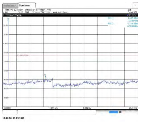
Band4-15MHz-QPSK-20325-1RB#0-Range2:1 000~20000MHz
