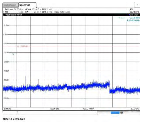
Band5-10MHz-QPSK-20525-1RB#0-Range2:1 000~10000MHz
