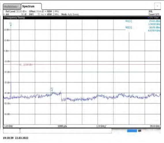
Band2-5MHz-QPSK-19175-1RB#0-Range2:10 00~20000MHz
