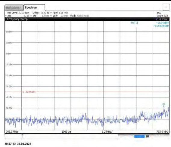
Band13-5MHz-QPSK-23205-1RB#0-Range3:7 63~775MHz
