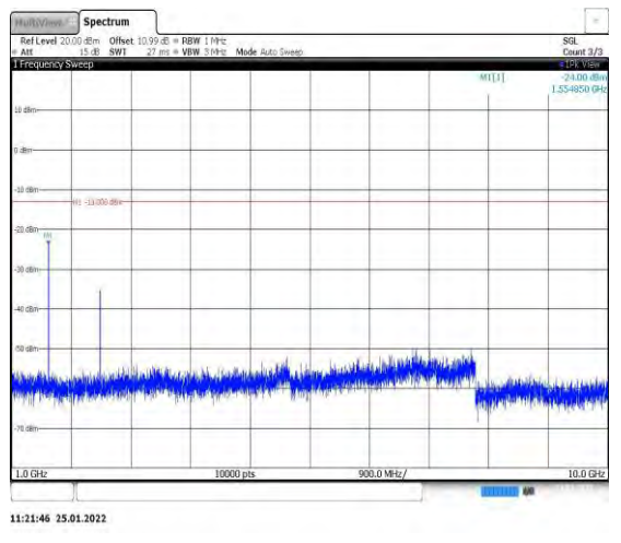
Band13-10MHz-QPSK-23230-1RB#0-Range2: 1000~10000MHz
