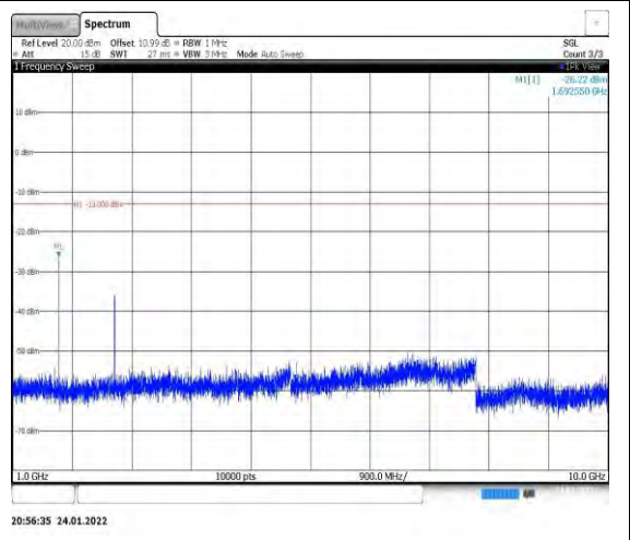
Band5-3MHz-QPSK-20635-1RB#0-Range2:10 00~10000MHz
