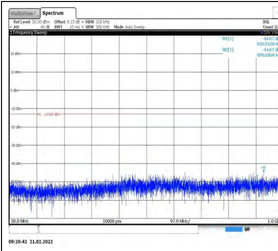
Band13-5MHz-QPSK-23255-1RB#0-Range 1:30~1000MHz
