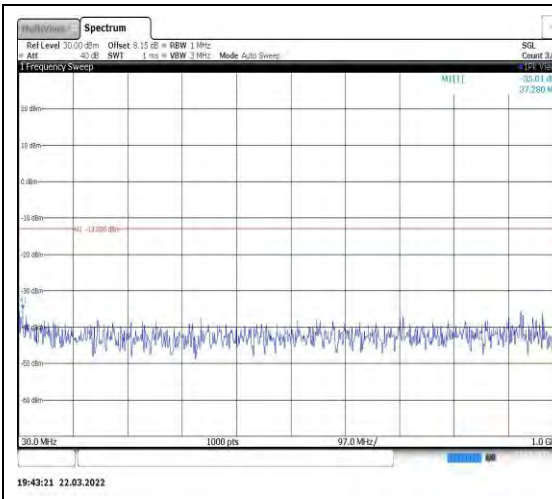
Band4-20MHz-QPSK-20050-1RB#0-Range 1:30~1000MHz
