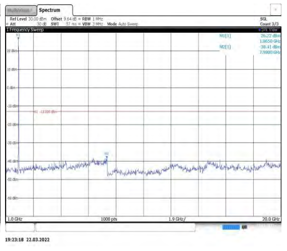
Band2-15MHz-QPSK-18900-1RB#0-Range2:1 000~20000MHz
