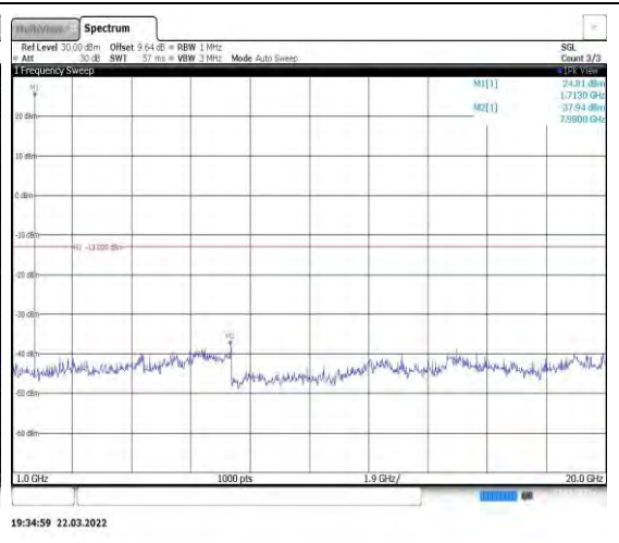
Band4-5MHz-QPSK-19975-1RB#0-Range2:10 00~20000MHz
