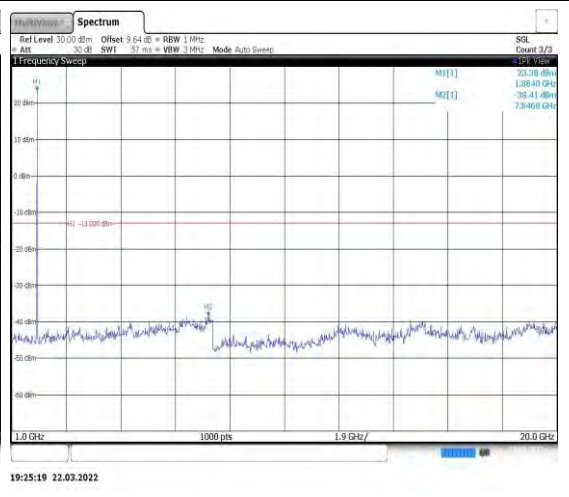
Band2-20MHz-QPSK-19100-1RB#0-Range2:1 000~20000MHz
