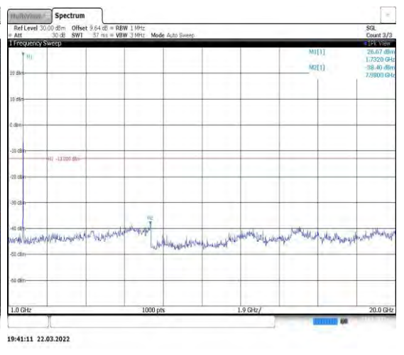
Band4-15MHz-QPSK-20175-1RB#0-Range2:1 000~20000MHz
