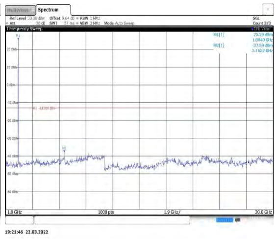
Band2-10MHz-QPSK-18900-1RB#0-Range2:1 000~20000MHz
