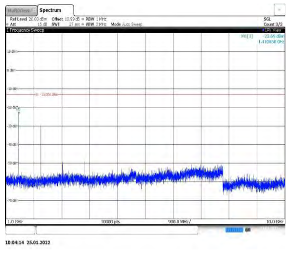
Band12-5MHz-QPSK-23095-1RB#0-Range2:1 000~10000MHz
