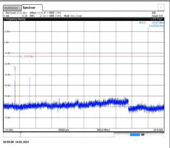
Band5-3MHz-QPSK-20415-1RB#0-Range2:10 00~10000MHz
