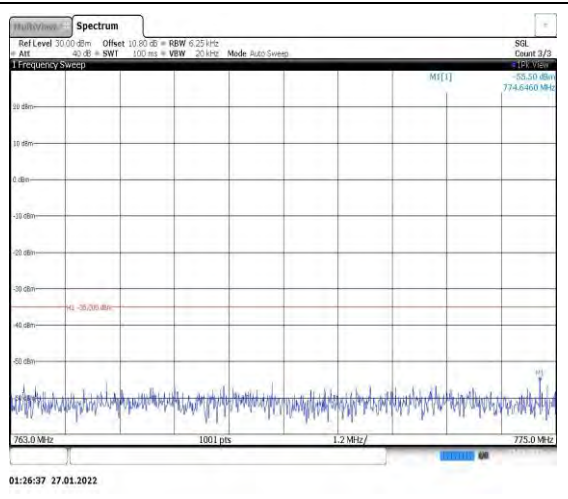
Band13-5MHz-QPSK-23255-1RB#0-Range3:7 63~775MHz
