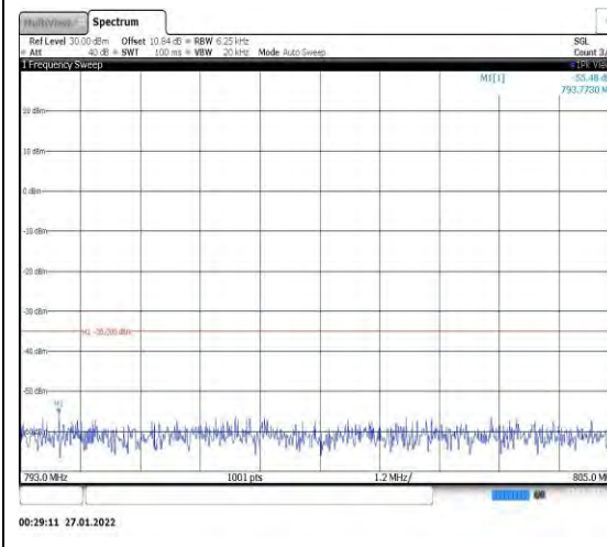
Band13-5MHz-QPSK-23230-1RB#0-Range 4:793~805MHz
