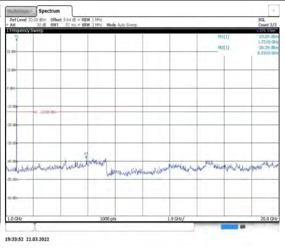
Band4-3MHz-QPSK-20385-1RB#0-Range2:10 00~20000MHz
