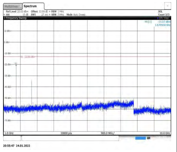
Band5-3MHz-QPSK-20525-1RB#0-Range2:10 00~10000MHz
