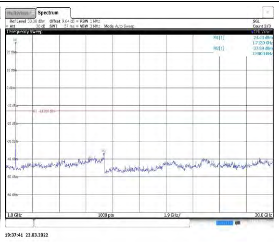
Band4-10MHz-QPSK-20000-1RB#0-Range2:1 000~20000MHz
