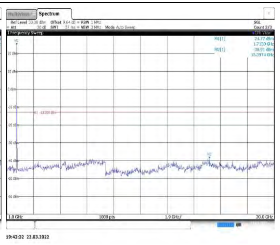
Band4-20MHz-QPSK-20050-1RB#0-Range2:1 000~20000MHz
