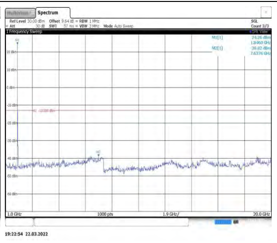
Band2-15MHz-QPSK-18675-1RB#0-Range2:1 000~20000MHz
