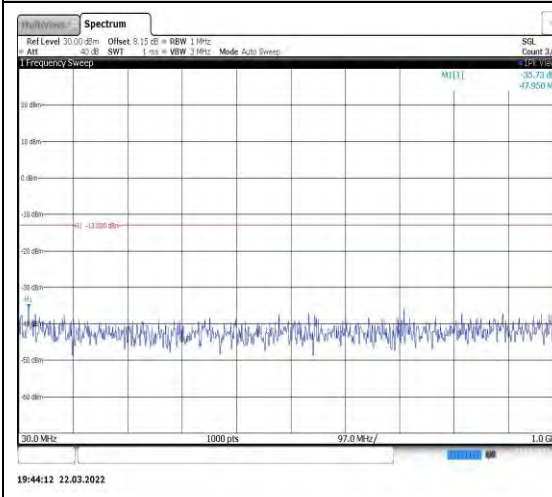
Band4-20MHz-QPSK-20300-1RB#0-Range 1:30~1000MHz
