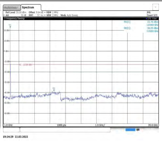
Band2-20MHz-QPSK-18700-1RB#0-Range2:1 000~20000MHz
