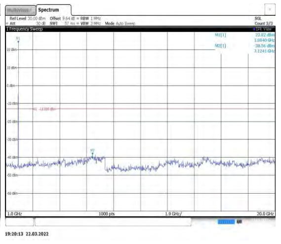
Band2-5MHz-QPSK-18900-1RB#0-Range2:10 00~20000MHz
