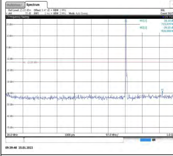
Band12-3MHz-QPSK-23165-1RB#0-Range 1:30~1000MHz
