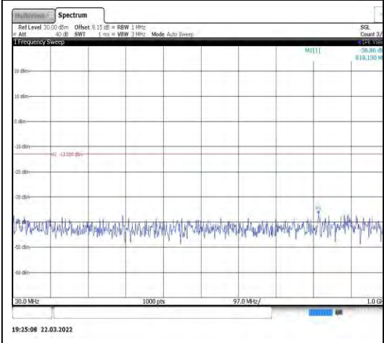
Band2-20MHz-QPSK-19100-1RB#0-Range 1:30~1000MHz
