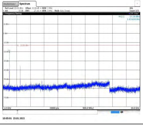
Band12-5MHz-QPSK-23155-1RB#0-Range2:1 000~10000MHz
