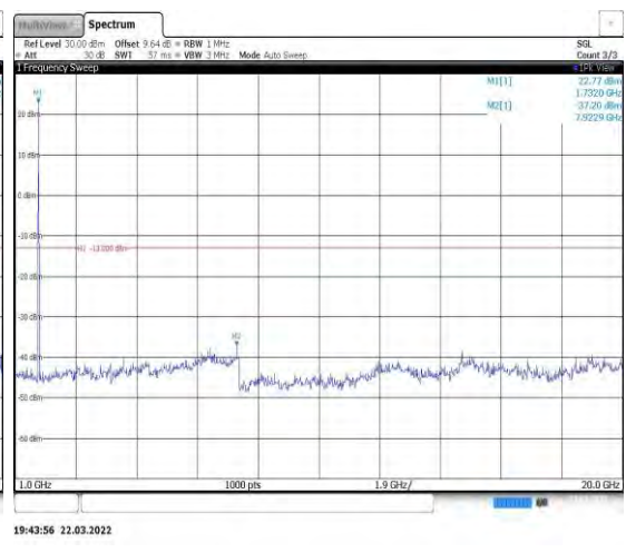
Band4-20MHz-QPSK-20175-1RB#0-Range2:1 000~20000MHz
