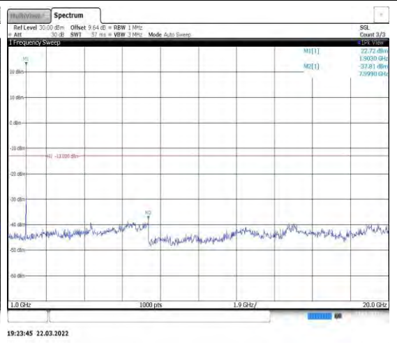
Band2-15MHz-QPSK-19125-1RB#0-Range2:1 000~20000MHz
