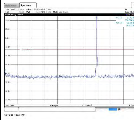
Band12-10MHz-QPSK-23130-1RB#0-Rang e1:30~1000MHz
