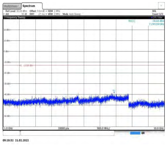
Band13-5MHz-QPSK-23255-1RB#0-Range2:1 000~10000MHz
