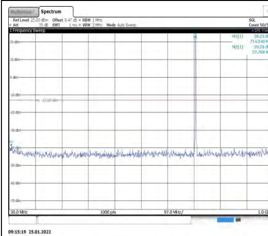
Band12-1.4MHz-QPSK-23173-1RB#0-Rang e1:30~1000MHz
