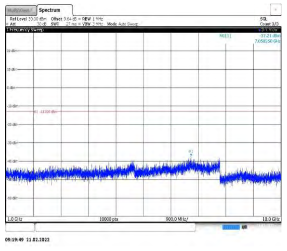
Band13-5MHz-QPSK-23230-1RB#0-Range2:1 000~10000MHz
