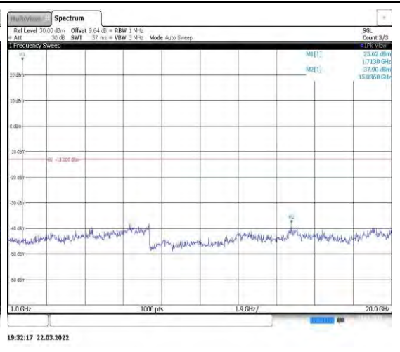
Band4-3MHz-QPSK-19965-1RB#0-Range2:10 00~20000MHz
