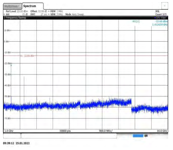
Band12-3MHz-QPSK-23095-1RB#0-Range2:1 000~10000MHz
