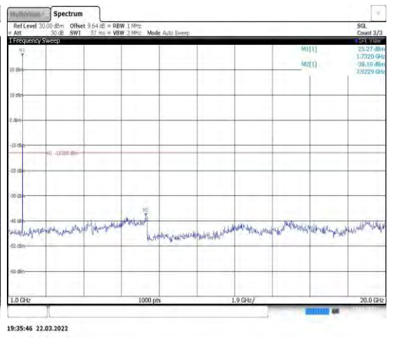
Band4-5MHz-QPSK-20175-1RB#0-Range2:10 00~20000MHz
