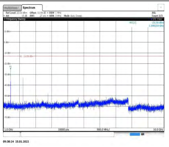
Band12-3MHz-QPSK-23025-1RB#0-Range2:1 000~10000MHz
