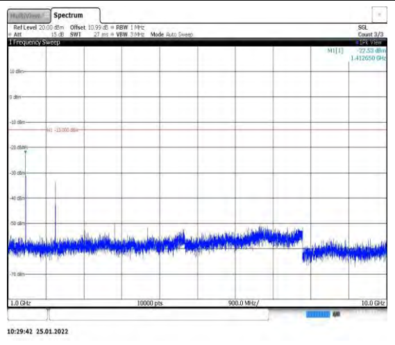
Band12-10MHz-QPSK-23130-1RB#0-Range2: 1000~10000MHz
