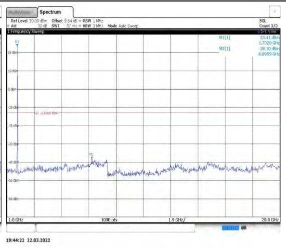
Band4-20MHz-QPSK-20300-1RB#0-Range2:1 000~20000MHz
