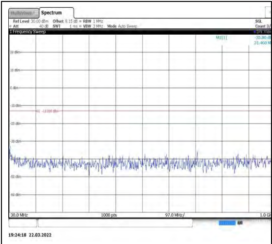
Band2-20MHz-QPSK-18700-1RB#0-Range 1:30~1000MHz
