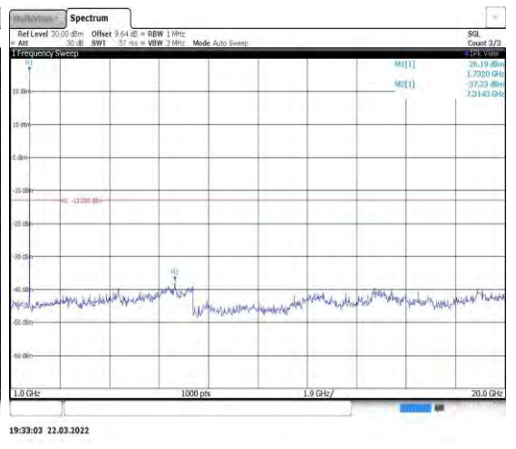
Band4-3MHz-QPSK-20175-1RB#0-Range2:10 00~20000MHz
