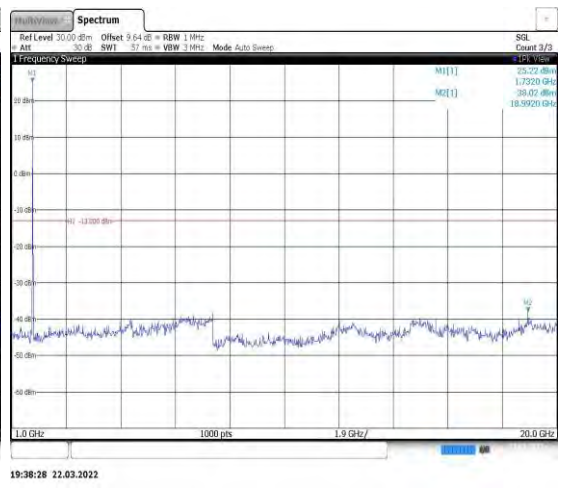
Band4-10MHz-QPSK-20175-1RB#0-Range2:1 000~20000MHz
