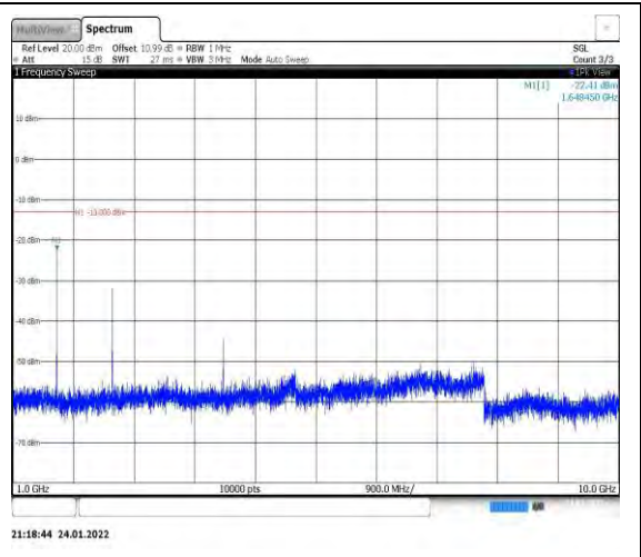
Band5-5MHz-QPSK-20425-1RB#0-Range2:10 00~10000MHz
