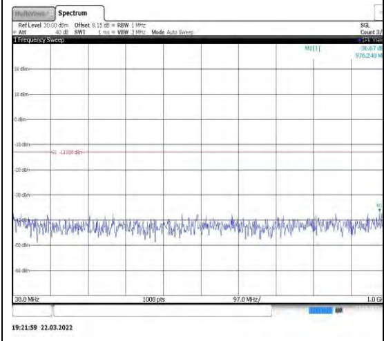
Band2-10MHz-QPSK-19150-1RB#0-Range 1:30~1000MHz
