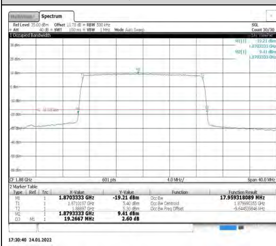
Band2-20MHz-QPSK-18900-100RB#0
