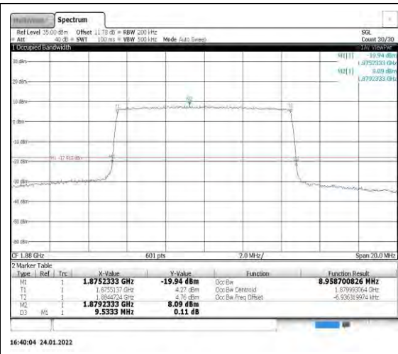
Band2-10MHz-16QAM-18900-50RB#0
