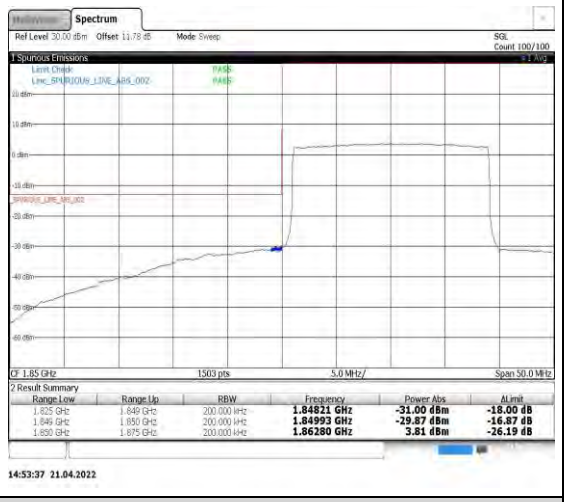
Band2-20MHz-16QAM-18700-100RB#0
