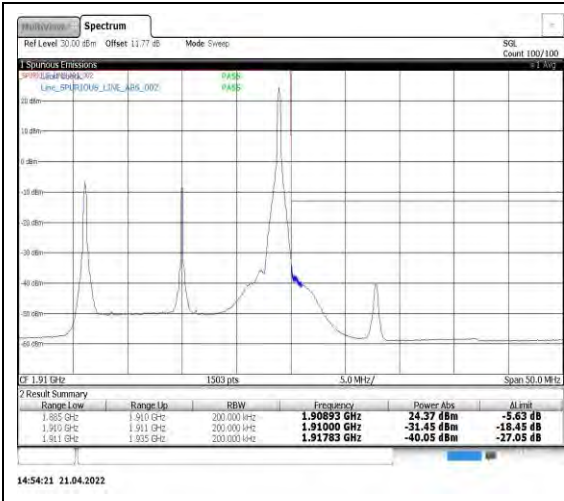
Band2-20MHz-QPSK-19100-1RB#99
