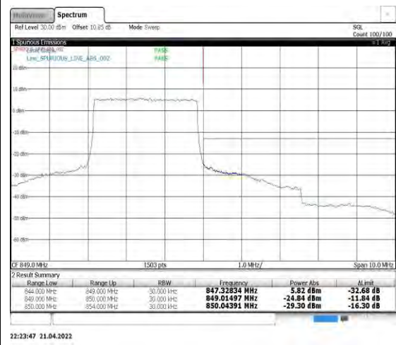
Band5-3MHz-QPSK-20635-15RB#0
