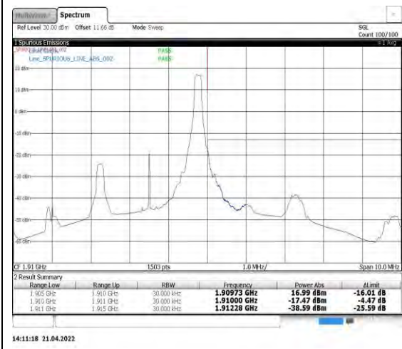
Band2-3MHz-QPSK-19185-1RB#14
