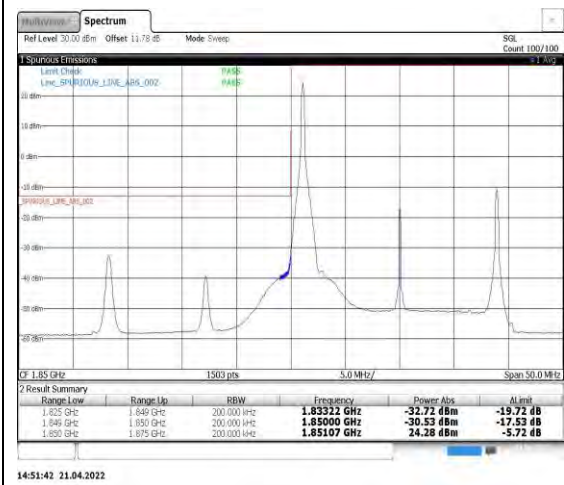
Band2-20MHz-QPSK-18700-1RB#0
