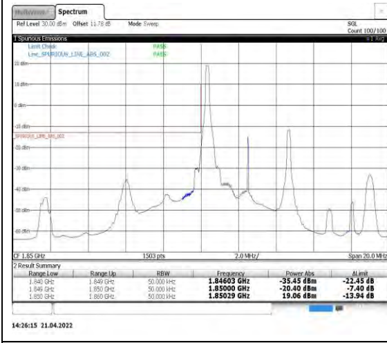
Band2-5MHz-QPSK-18625-1RB#0
