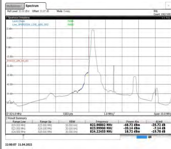
Band5-3MHz-QPSK-20415-1RB#0
