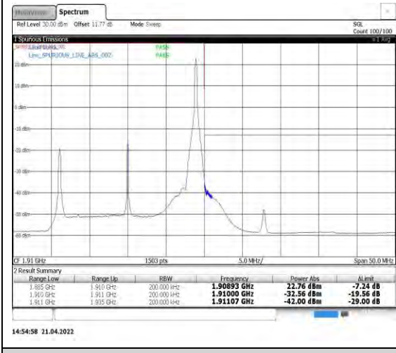
Band2-20MHz-16QAM-19100-1RB#99
