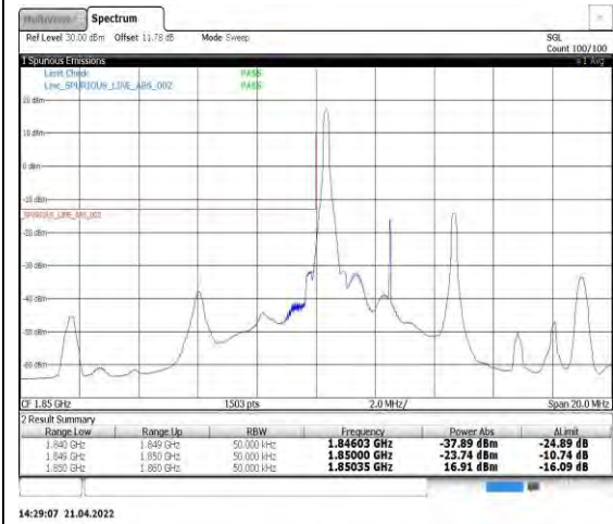
Band2-5MHz-16QAM-18625-1RB#0
