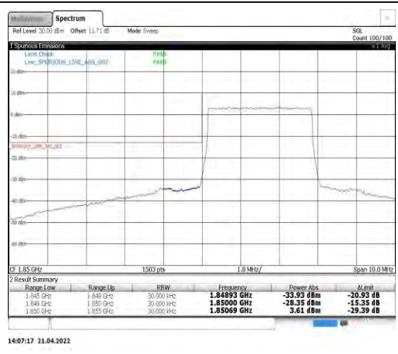
Band2-3MHz-16QAM-18615-15RB#0
