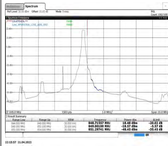
Band5-3MHz-QPSK-20635-1RB#14
