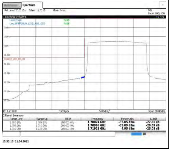
Band4-20MHz-QPSK-20050-100RB#0
