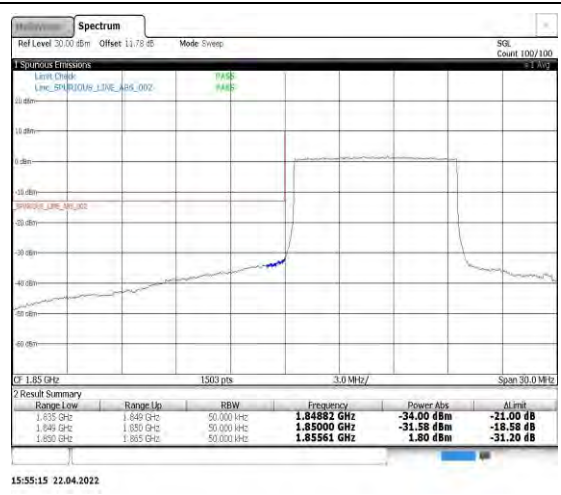
Band2-10MHz-QPSK-18650-50RB#0
