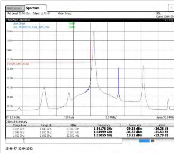
Band2-10MHz-QPSK-18650-1RB#0
