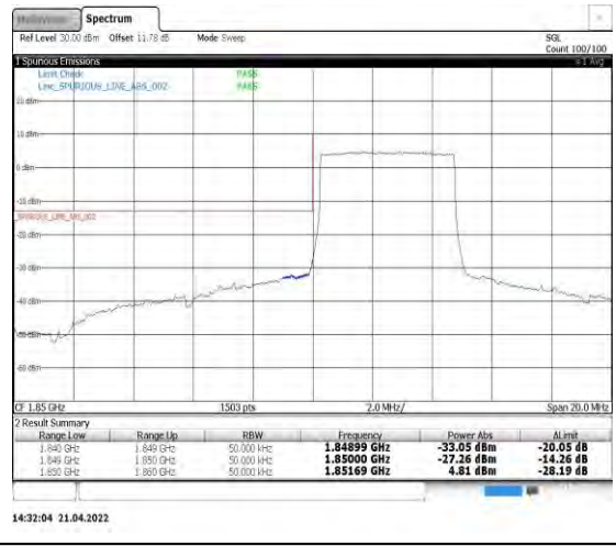
Band2-5MHz-QPSK-18625-25RB#0
