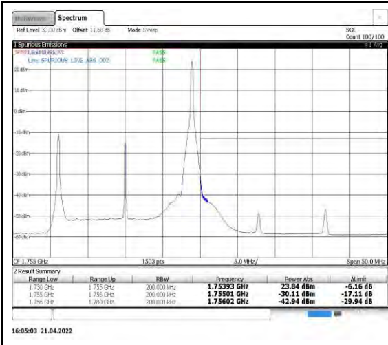
Band4-20MHz-QPSK-20300-1RB#99
