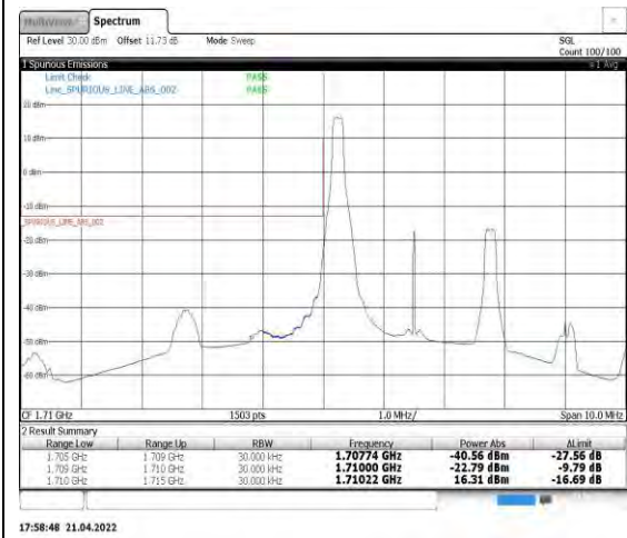
Band4-3MHz-QPSK-19965-1RB#0
