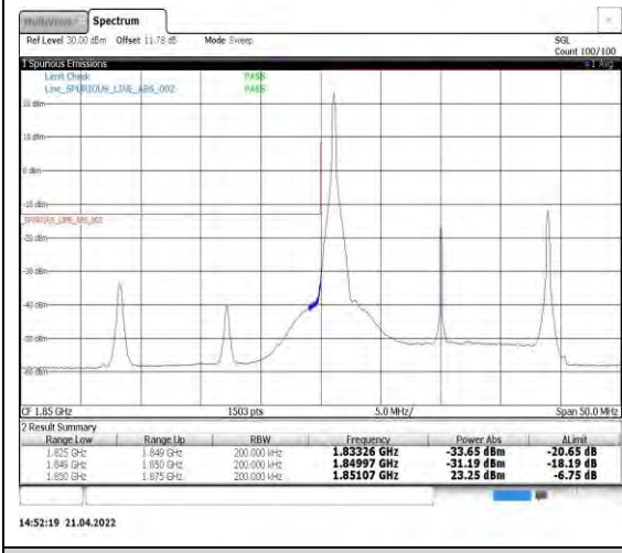
Band2-20MHz-16QAM-18700-1RB#0
