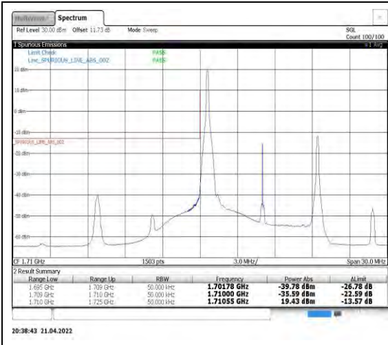
Band4-10MHz-QPSK-20000-1RB#0
