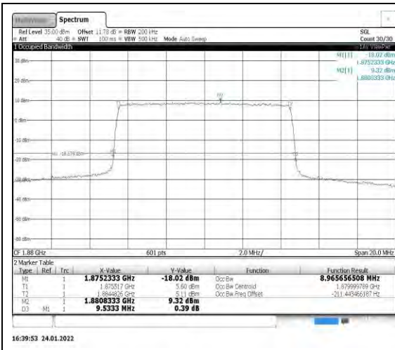
Band2-10MHz-QPSK-18900-50RB#0
