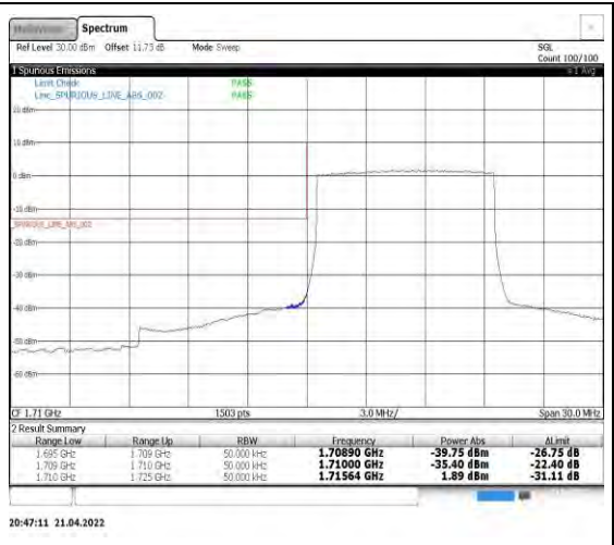
Band4-10MHz-QPSK-20000-50RB#0
