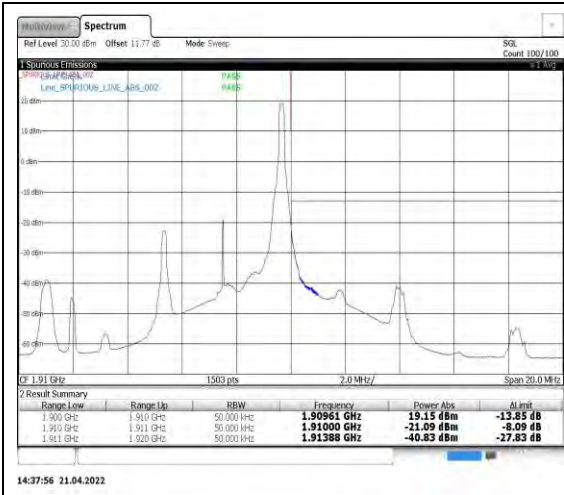
Band2-5MHz-QPSK-19175-1RB#24
