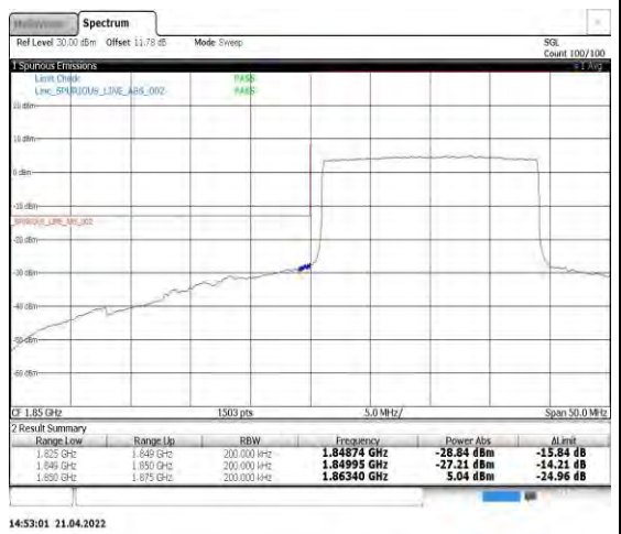
Band2-20MHz-QPSK-18700-100RB#0
