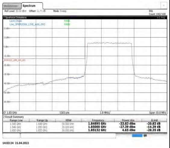
Band2-3MHz-QPSK-18615-15RB#0
