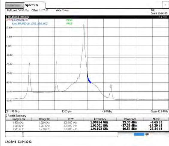
Band2-15MHz-16QAM-19125-1RB#74
