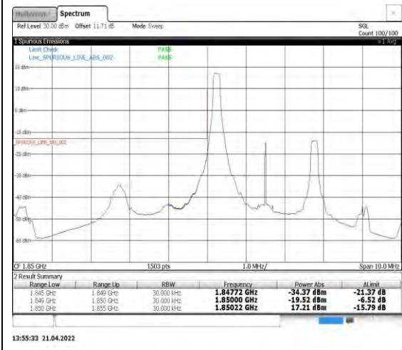
Band2-3MHz-QPSK-18615-1RB#0
