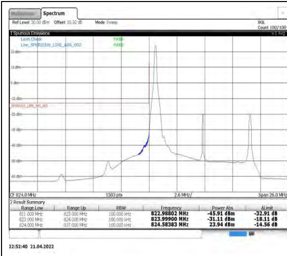
Band5-10MHz-QPSK-20450-1RB#0
