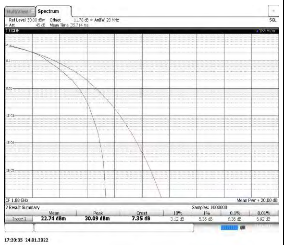
Band2-15MHz-16QAM-18900
