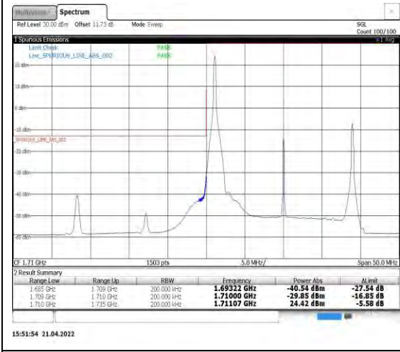
Band4-20MHz-QPSK-20050-1RB#0
