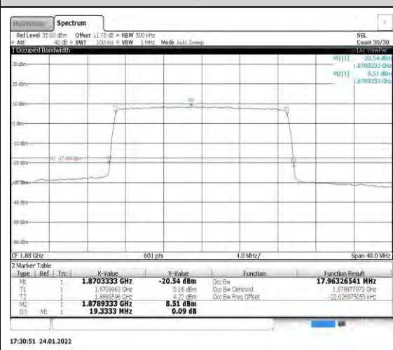
Band2-20MHz-16QAM-18900-100RB#0
