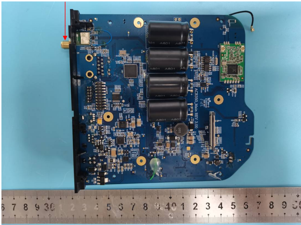
GNSS Port
