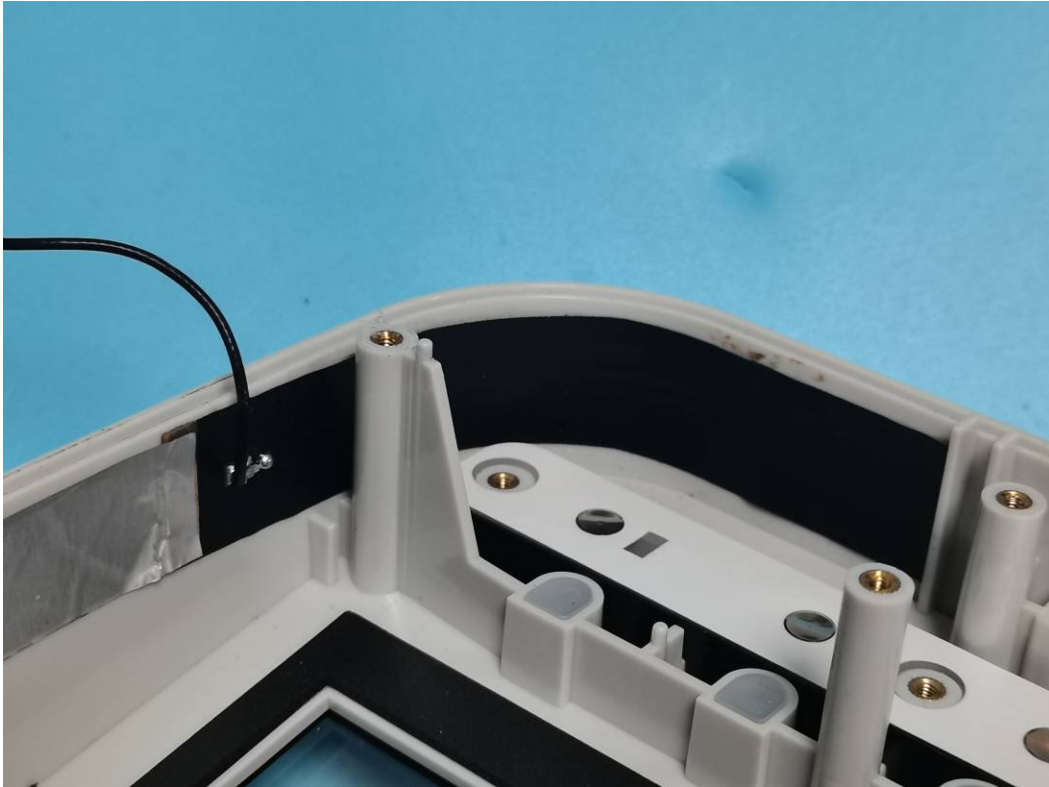
GSM & WCDMA & LTE Antenna
