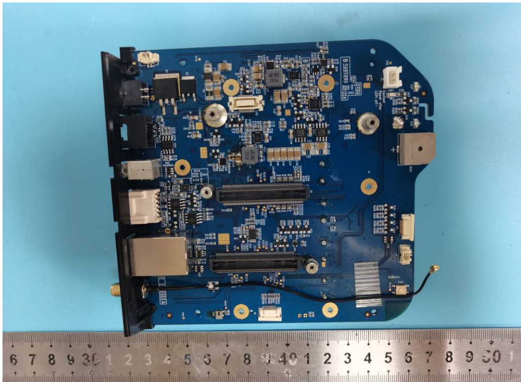
GNSS Port
