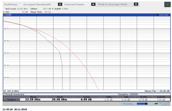
Figure 8.4-8: AGC -0.5 dB 707 MHz PAR UL
