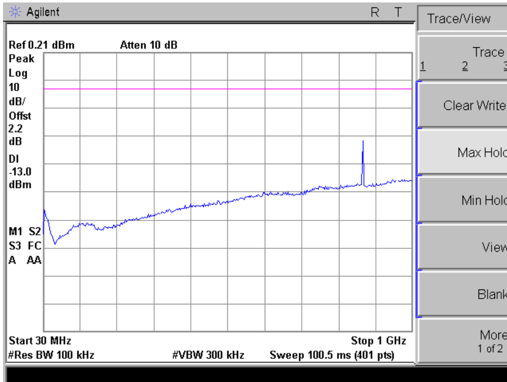
869MHz 30-1000MHz
