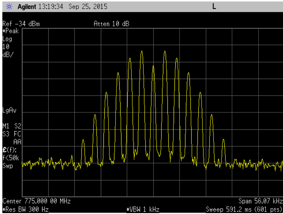
25KHz 775MHz Mod out Mask B +3dB
