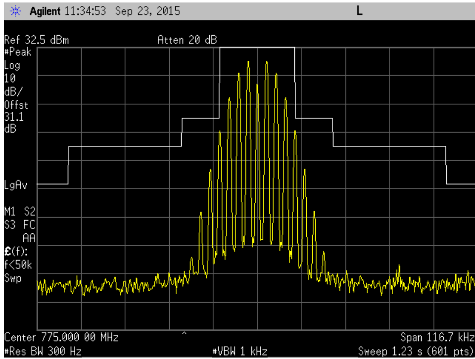
25KHz 775MHz Mod out mask C +3dB
