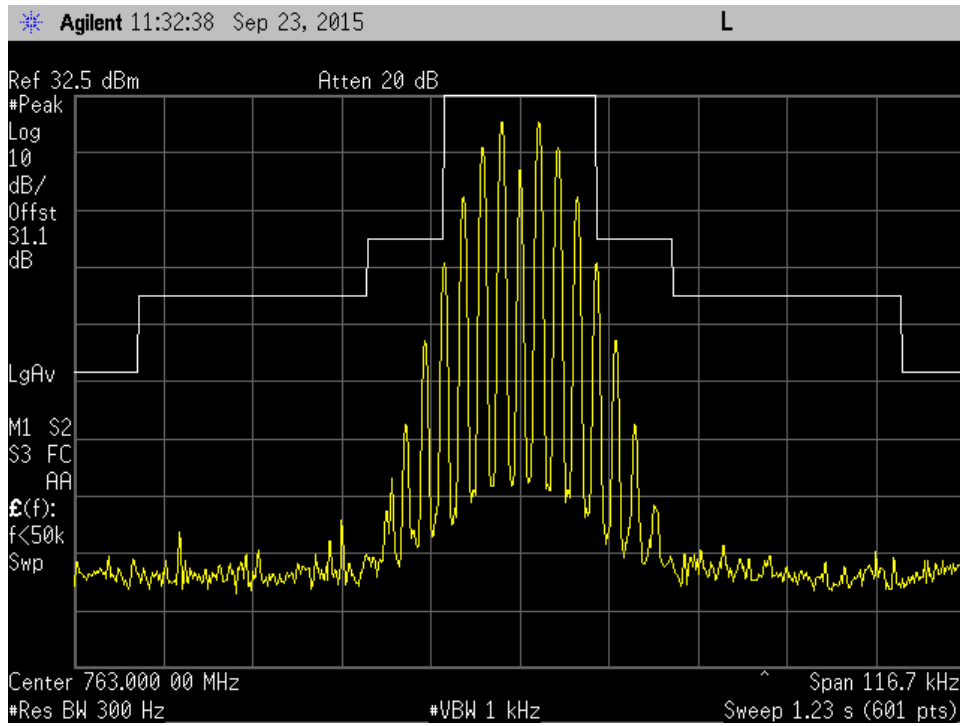
25KHz 763MHz Mod out mask C +3dB
