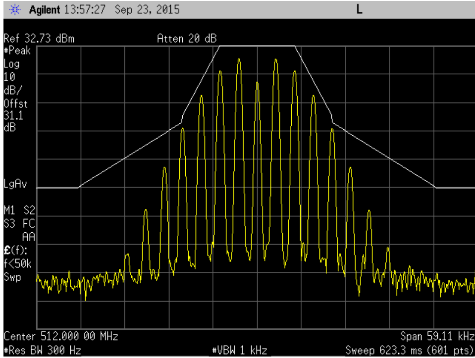
25kHz 512MHz Mod out mask C
