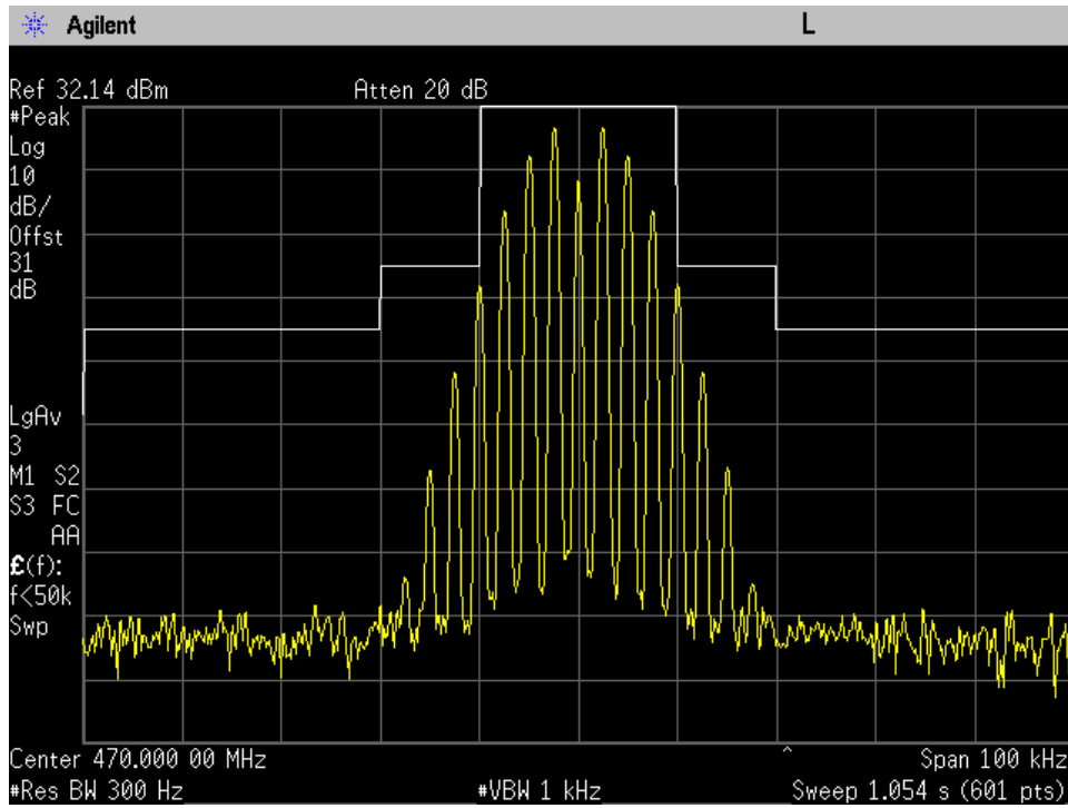
25KHz 470MHz Mod out Mask B
