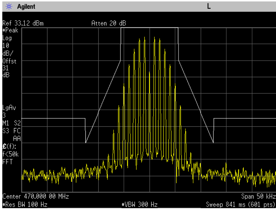
12.5KHz 470MHz Mod out Mask D
