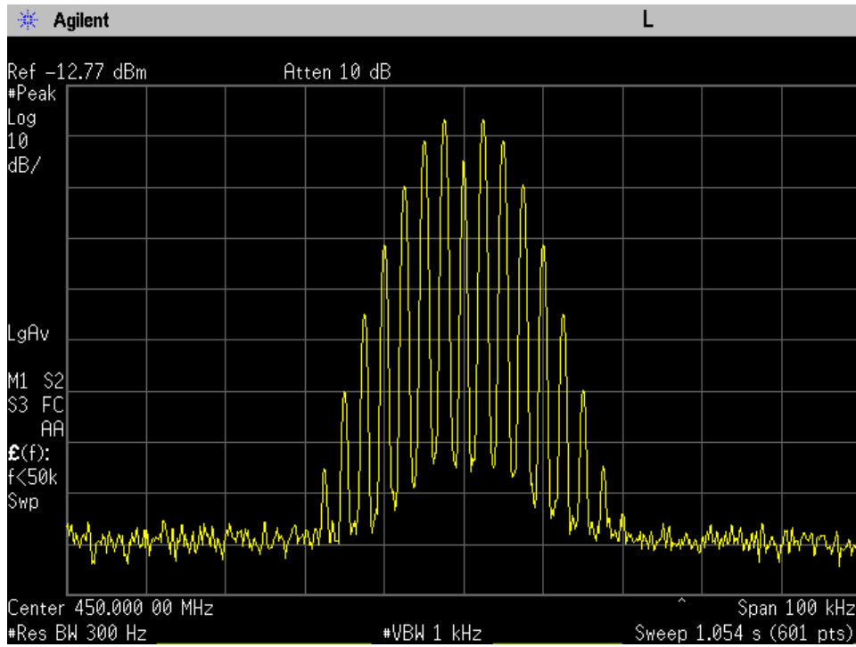
25KHz 450MHz Mod out Mask B +3dB
