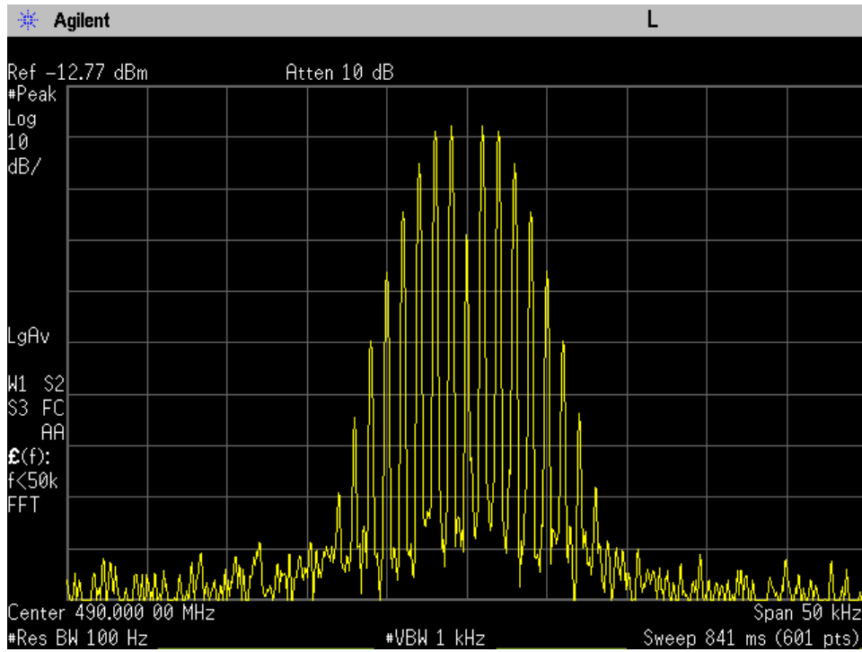
12.5KHz 490MHz Mod out Mask D
