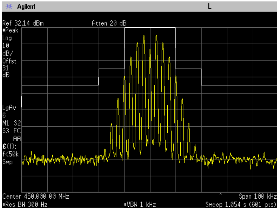
25kHz 450MHz Mod out mask C +3dB
