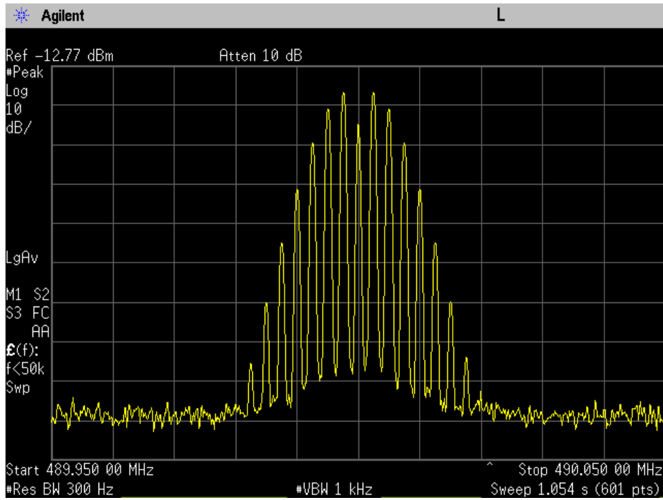
25KHz 490MHz Mod out Mask B +3dB
