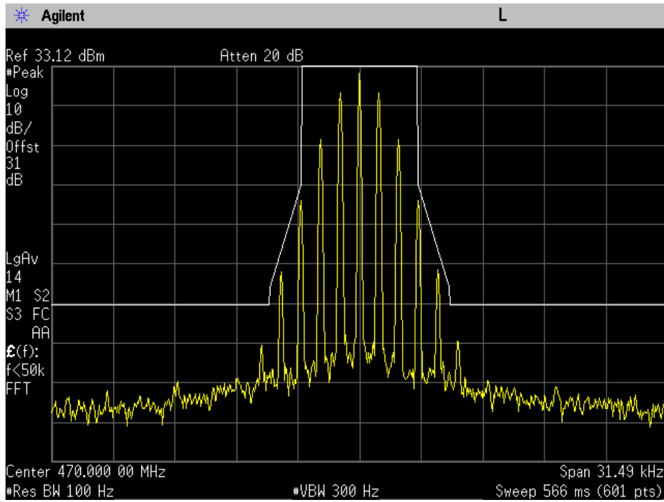
6.25KHz 470MHz Mod out Mask E
