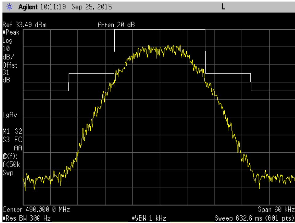
C4FM 490MHz Mod out mask B
