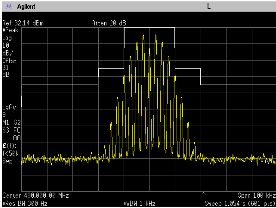
25kHz 490MHz Mod out mask C +3dB
