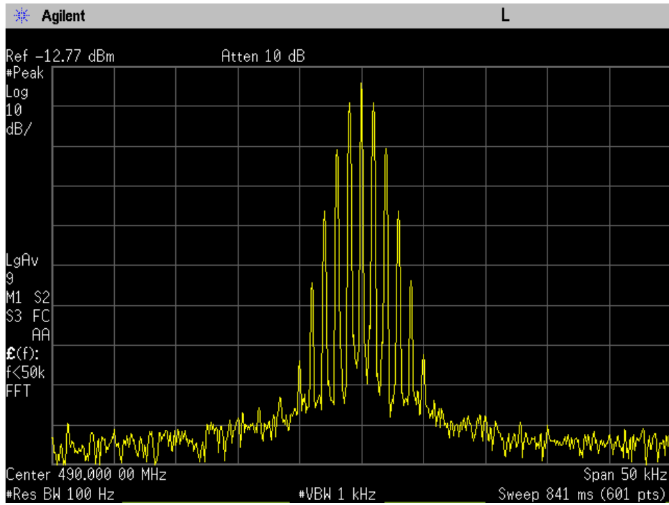
6.25KHz 490MHz Mod out Mask E +3dB
