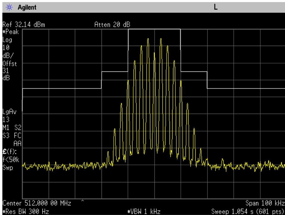
25KHz 512MHz Mod out Mask B
