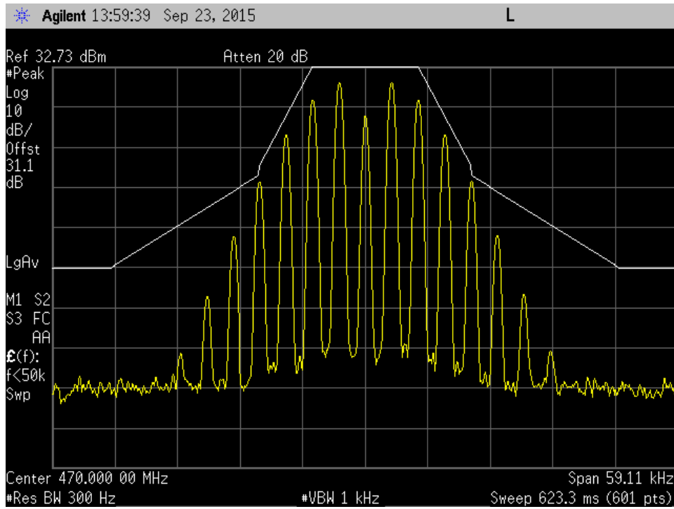
25kHz 470MHz Mod out mask C
