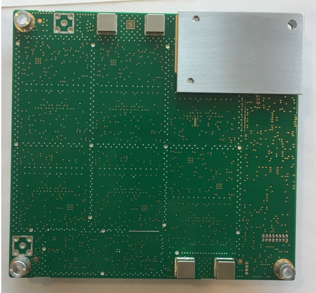
VGA bottom
