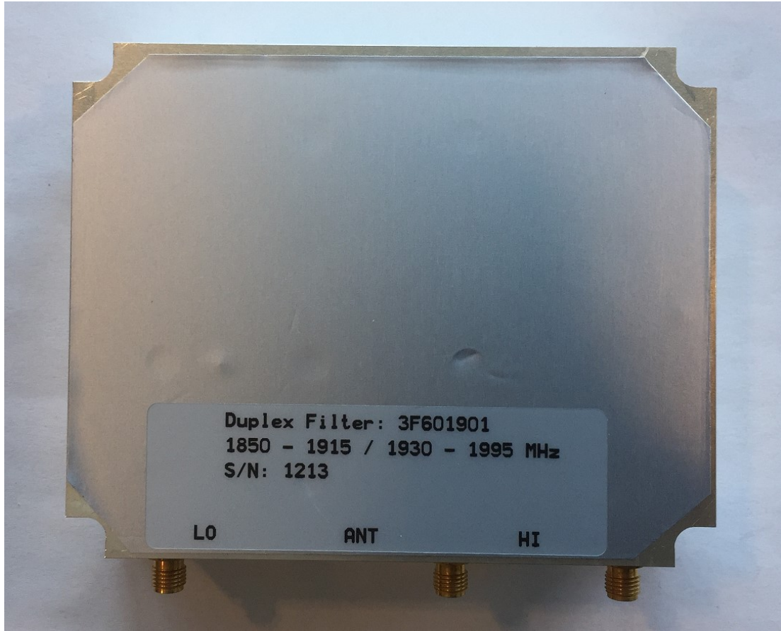
Duplexer top
