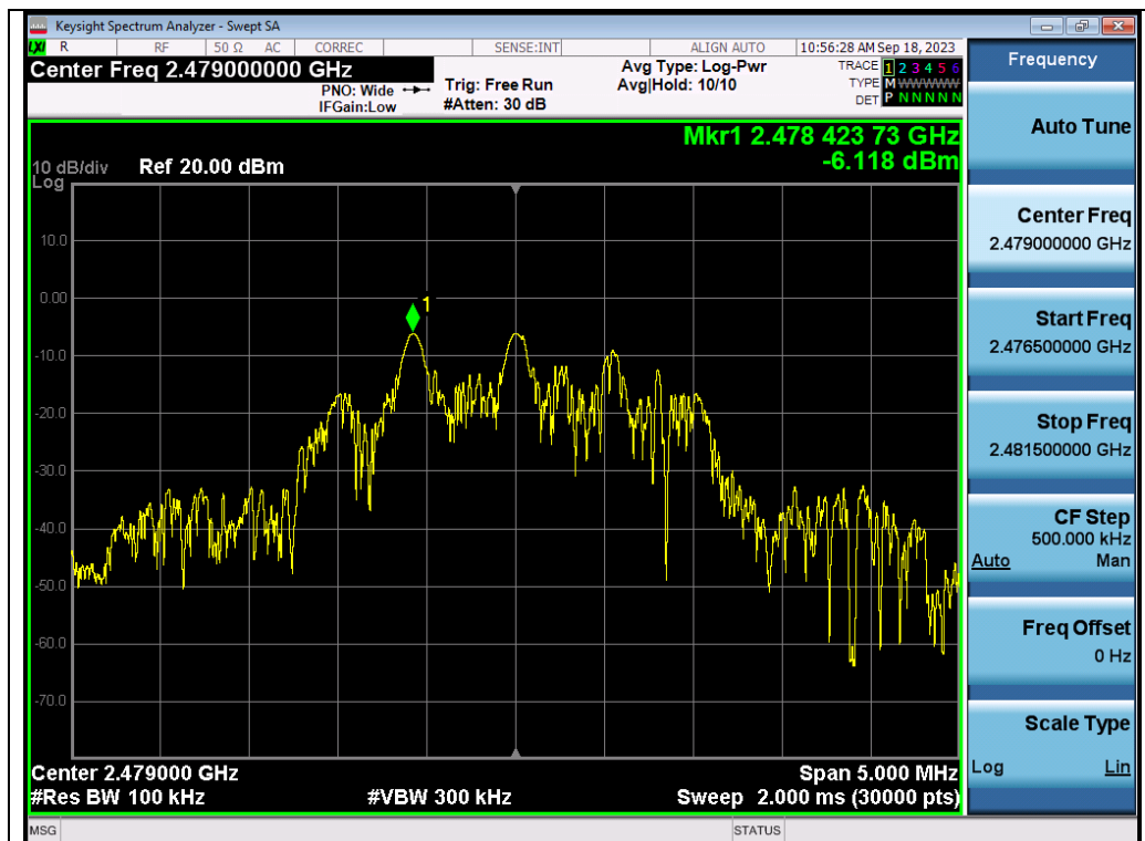
Test_Graph_GFSK_ANT1_2479_Reference Level
