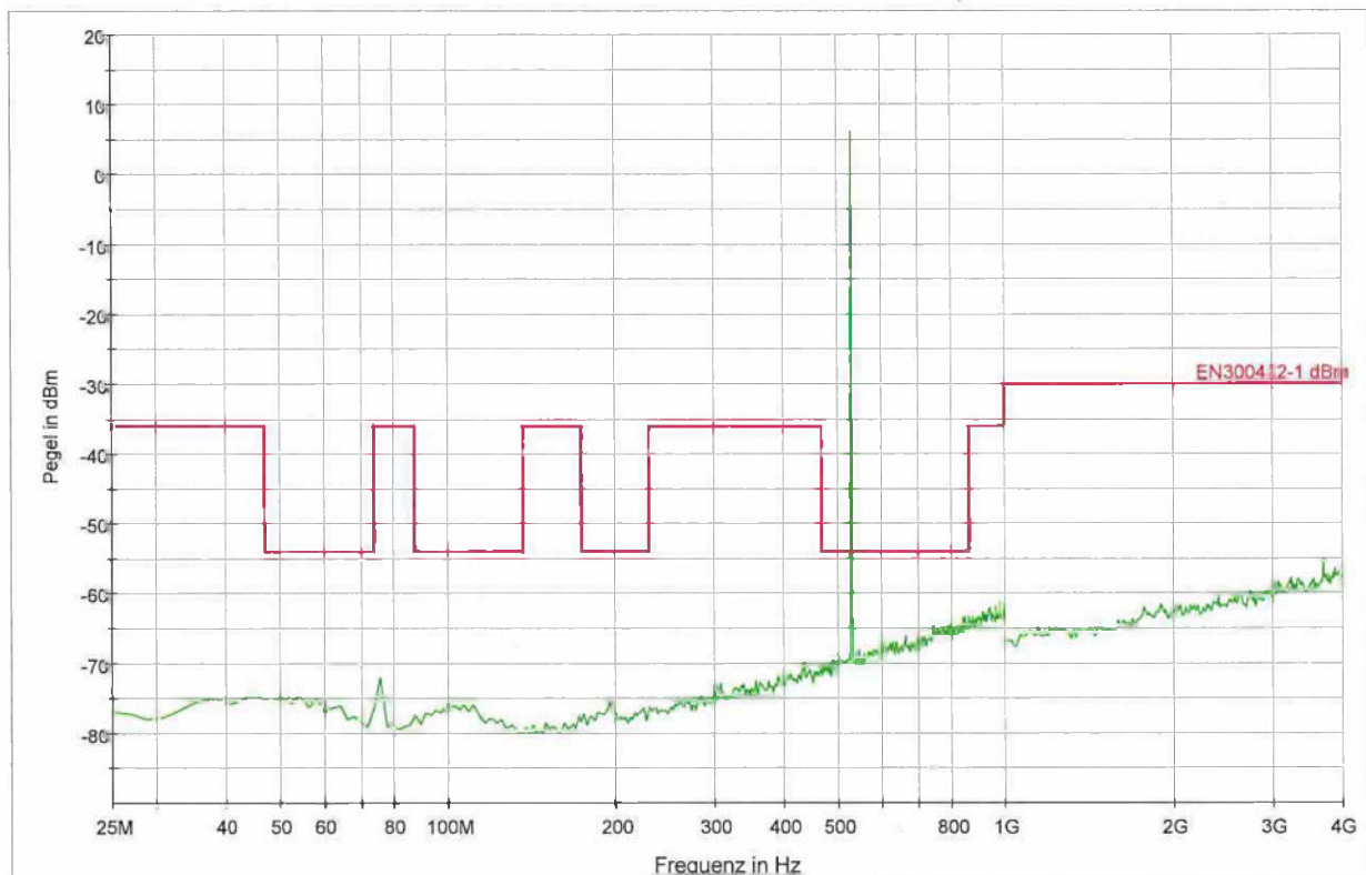
PK+_MAXH(1);HT45_A_CH1_F1 PK+_MAXH(1);HT45_A_CH1_F2 EN300422-1 dBm PK+_CLRWR PK+_MAXH
