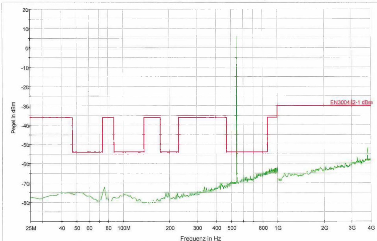
PK+_MAXH(1):HT45_A_CH2_F1 PK+_MAXH(1):HT45_A_CH2_F2 EN300422-1 dBm PK+_CLRWR PK+_MAXH
