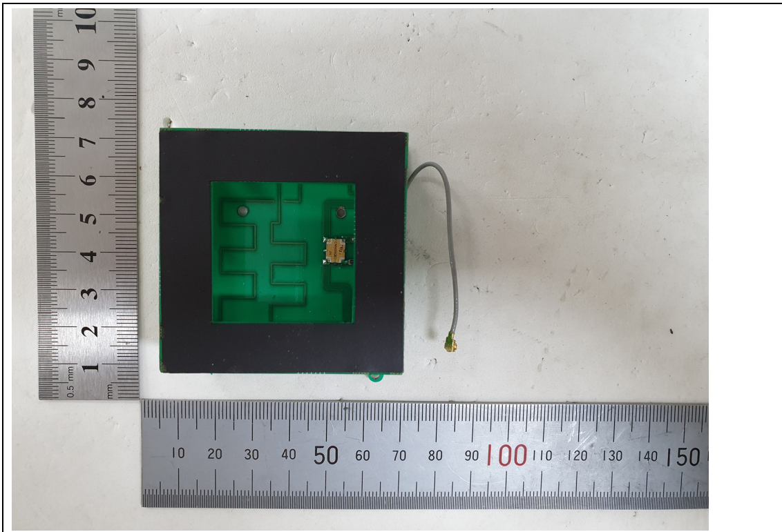
<RFID Antenna>
