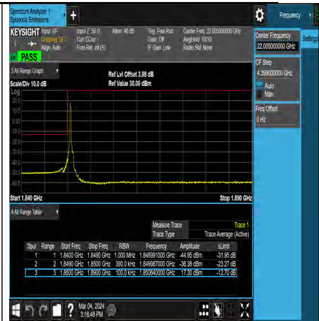
NTVN-N25-PC3-15-40-L-DFT-QPSK-Edge_1RB_Left-Ant0-PASS
