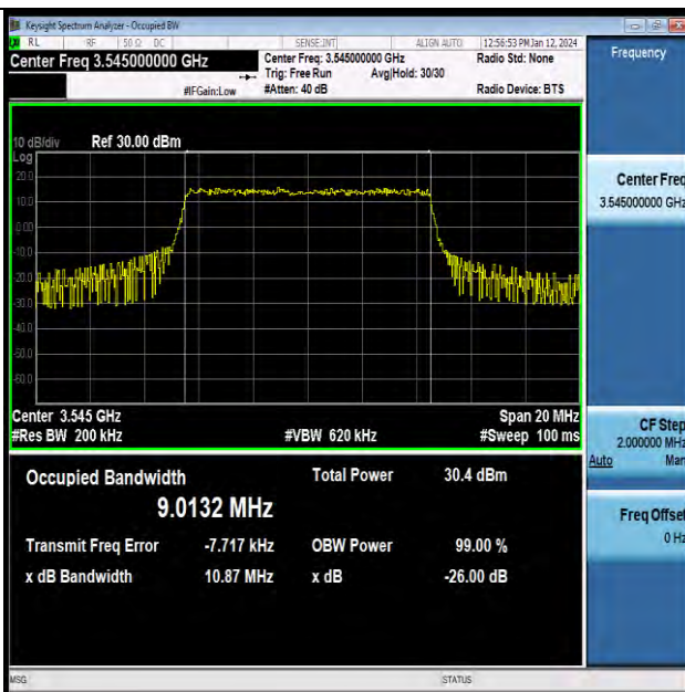
42(3450-3550)-10MHz-QPSK-43040-50RB#0-PASS
