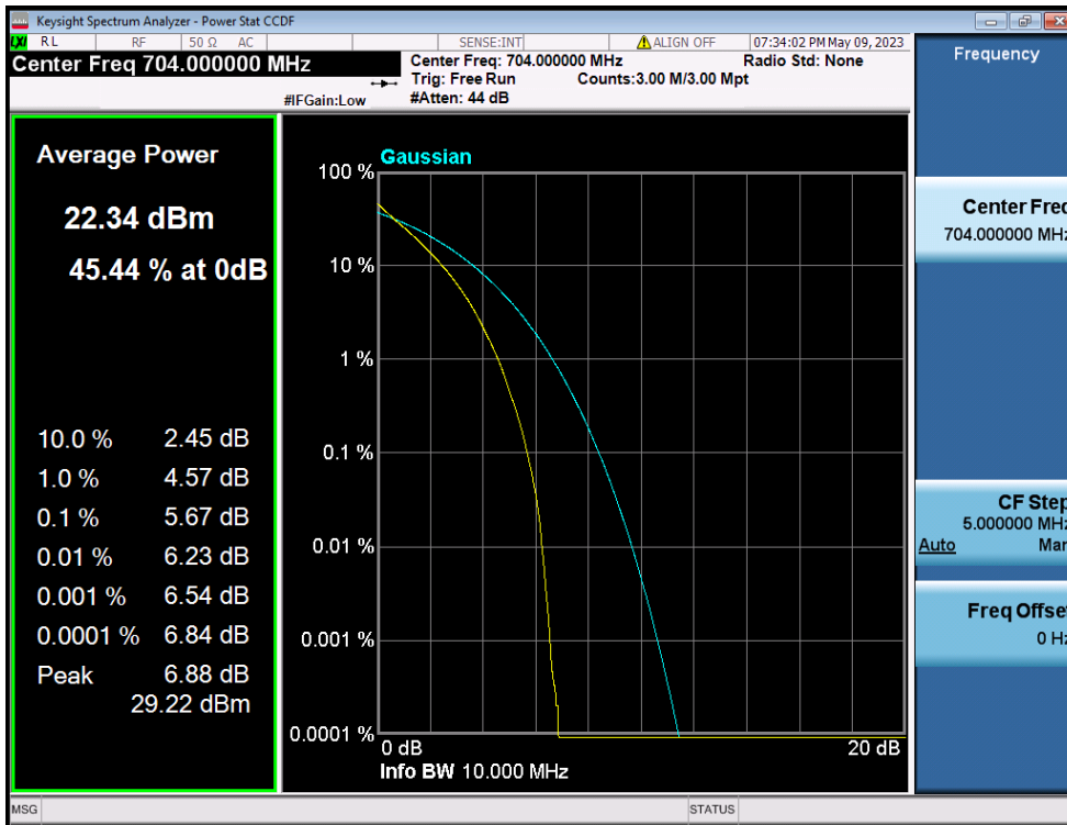
LTE Band 12(17) / 10MHz / QPSK - RB Size 50
