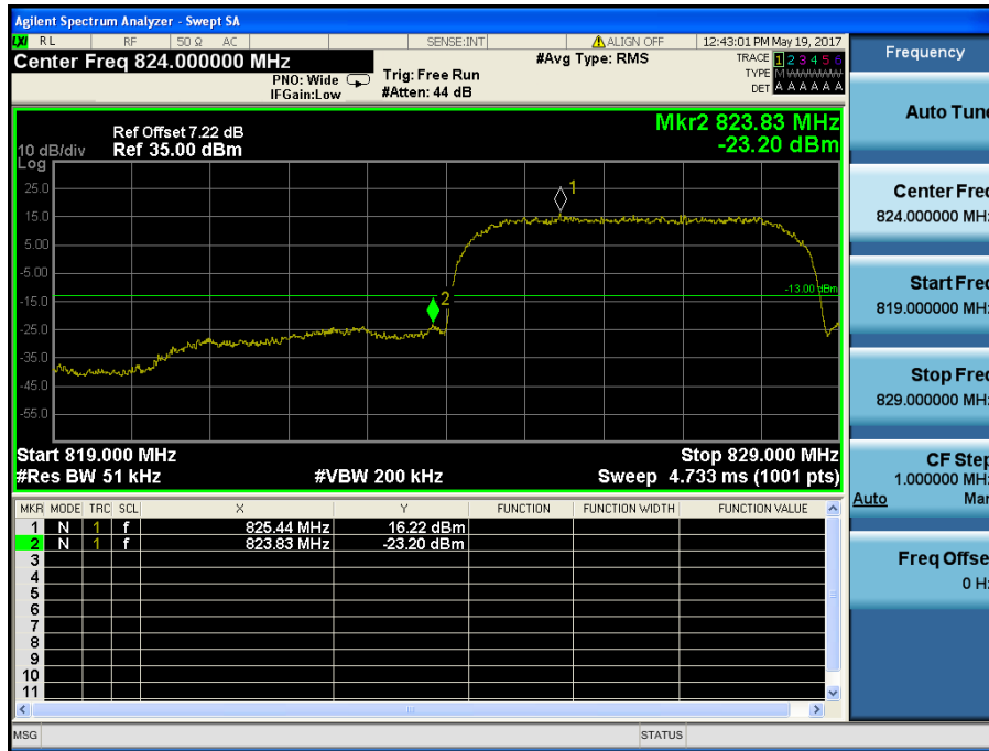
WCDMA850& Channel: 4132
