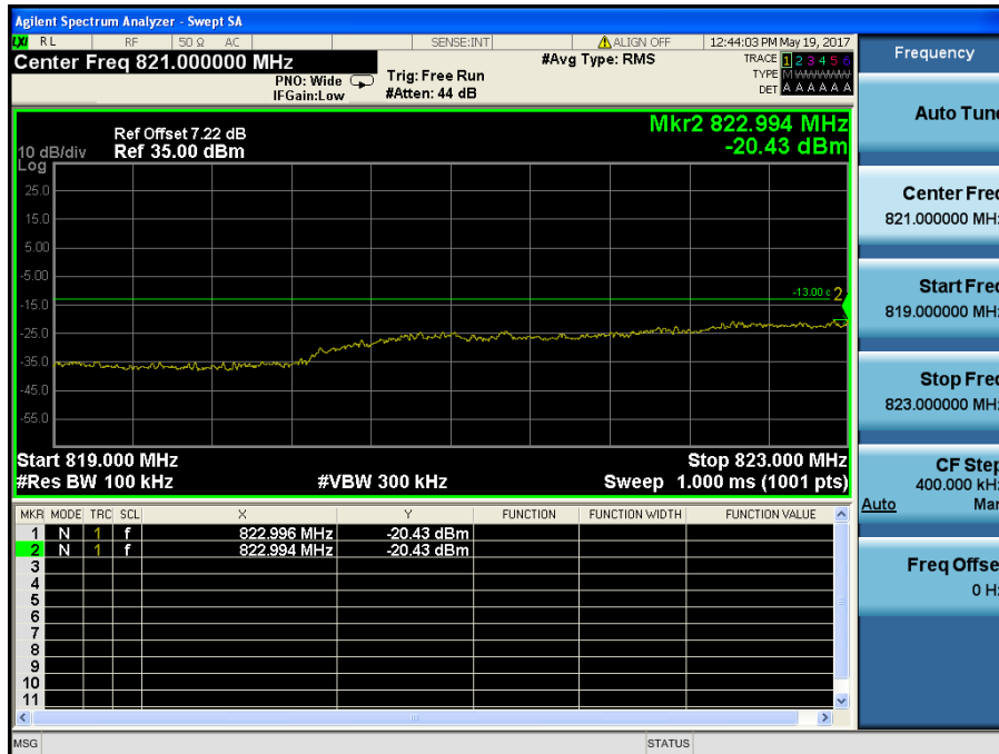
WCDMA850& Channel: 4132
